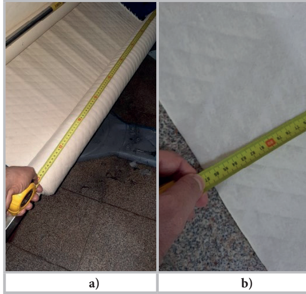
Görsel 1.12: Yuvarlak örme makinesinde üretilen kumaşın a) mekanik ve b) ham kumaş eni ölçümü
