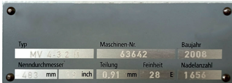
Görsel 1.3: Örme makinesi etiket levhasında incelik bilgisi
