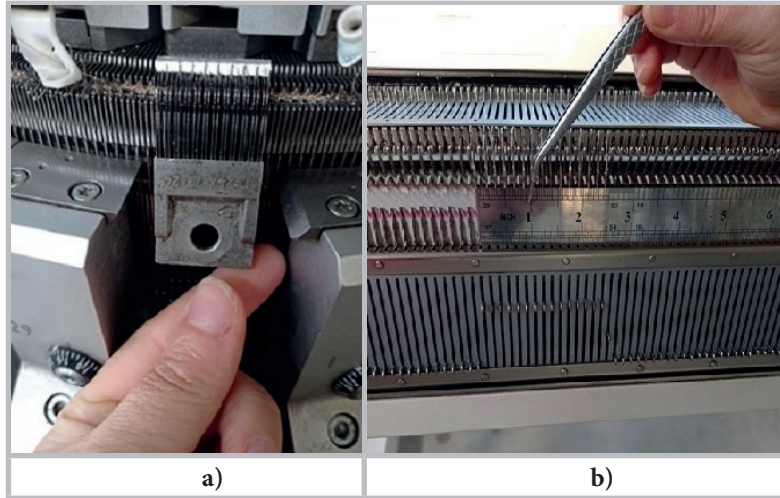
Görsel 1.2: a) Mastar ve b) cetvel ile makine inceliği ölçümü
