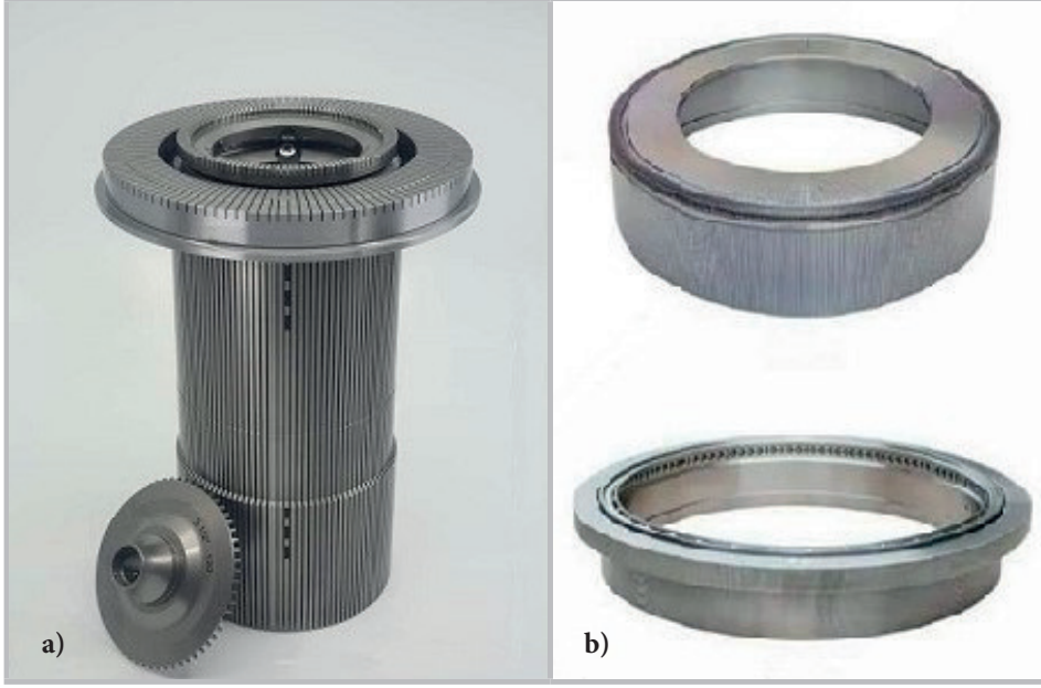
Görsel 1.4: Yuvarlak a) çorap ve b) penye örme makinelerinde kullanılan farklı çapta kovanlar
