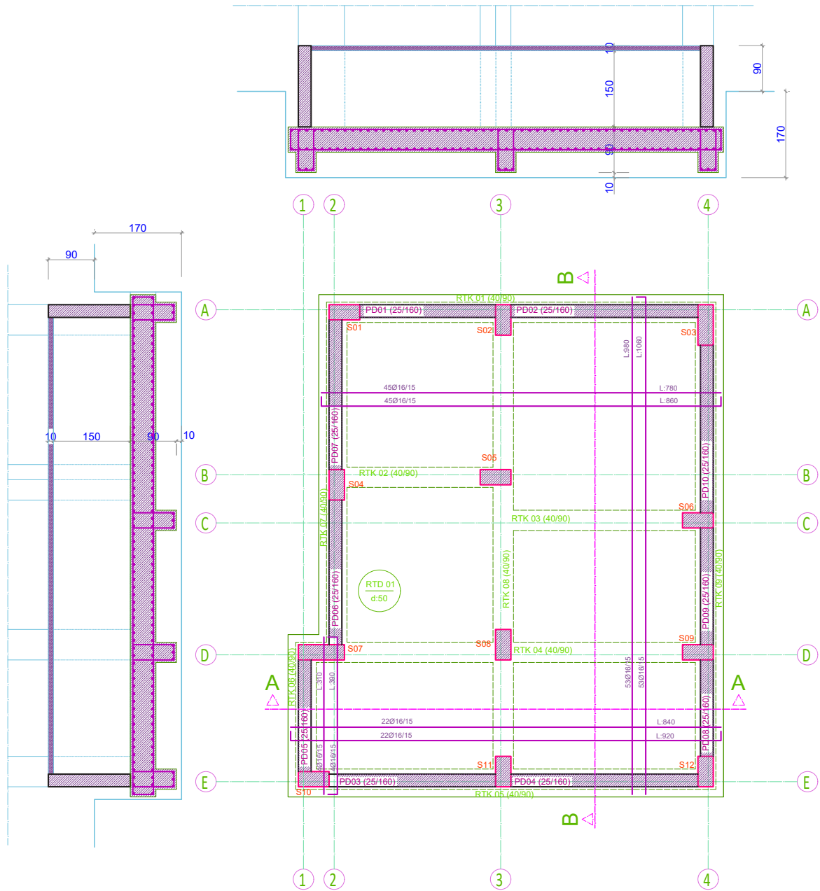
Çizim 9.11: Altan kirişli radye temel donatı çizimi
