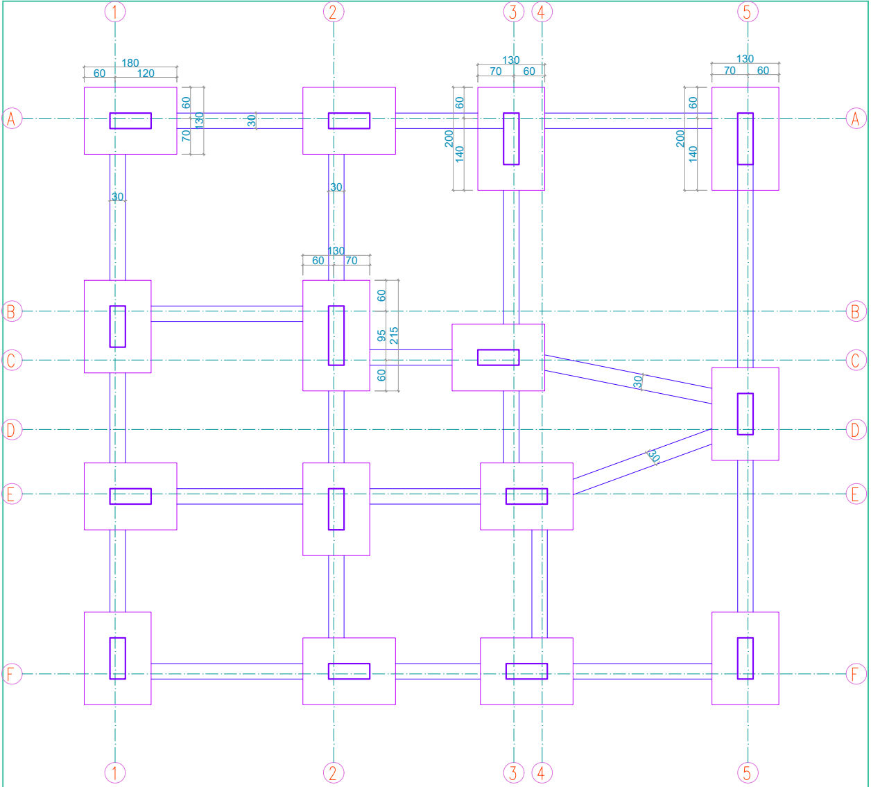
Çizim 8.9: Tekil temel ve bağ kirişi çizimi
