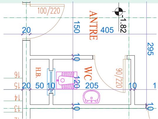
Çizim 7.6: Bodrum kat planı sabit eşya tefrişi
