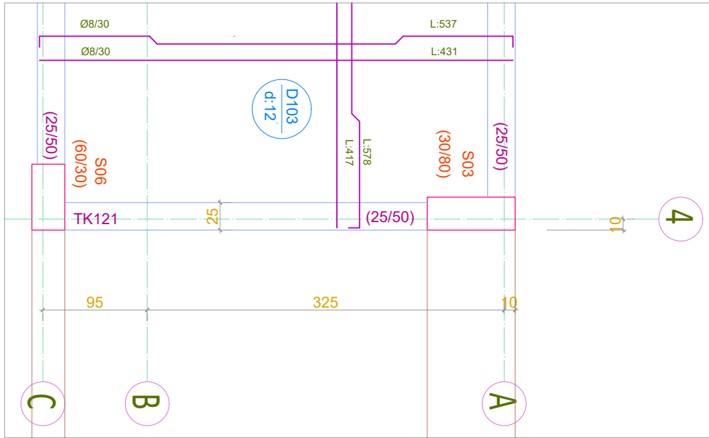
1. NORMAL KAT DÖŞEME KALIP VE DONATI PLANI ÖLÇEK 1/50
