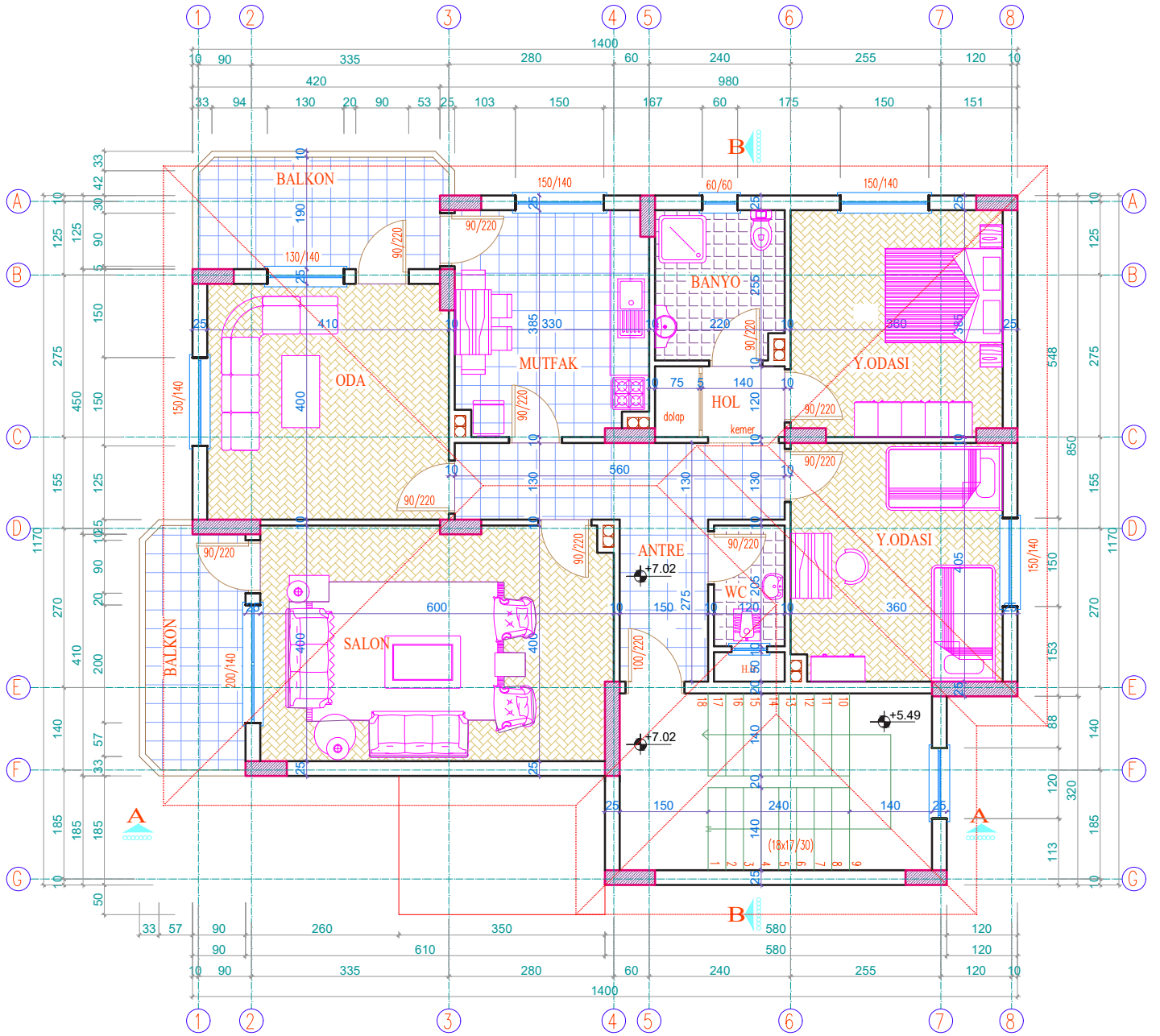
NORMAL KAT PLANI ÖLÇEK 1/50
