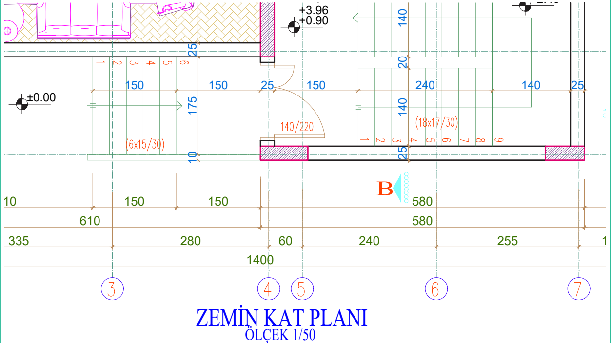
Çizim 5.14: Pafta ismi ve ölçek yazısı
