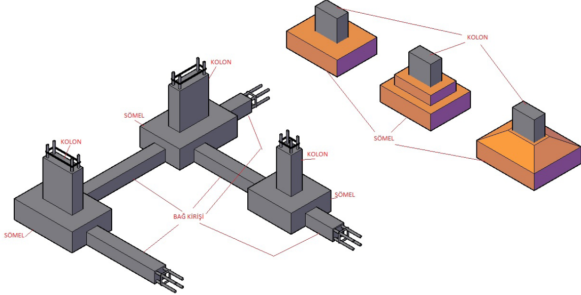
Görsel 8.2: Düz kademeli ve eğik tekil (münferit) temeller
