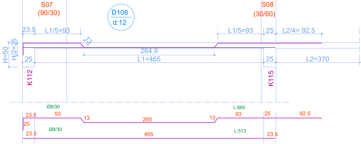
Çizim 11.9: Döşeme donatılarının çizimi ve hesaplanması
