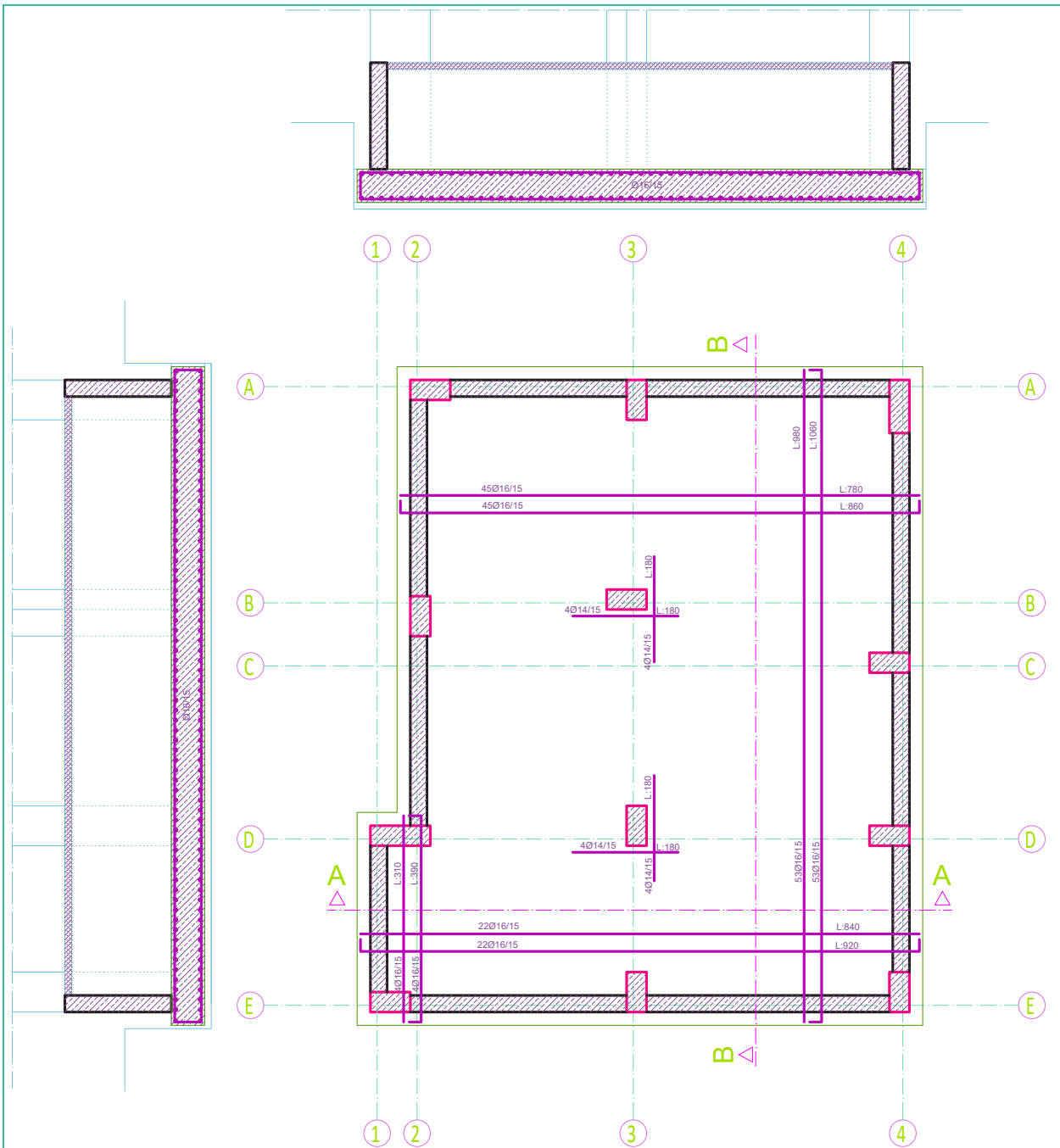
Çizim 9.4: Düz radye temel donatı çizimi
