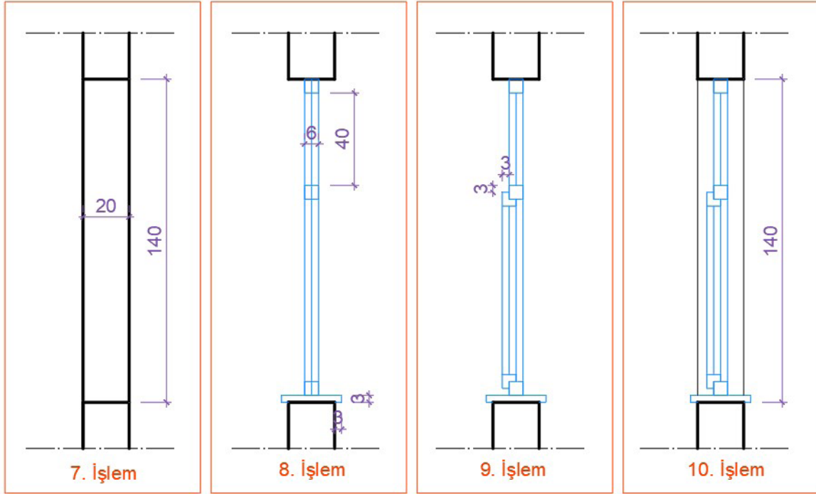
PENCERE A-A KESİTİ
