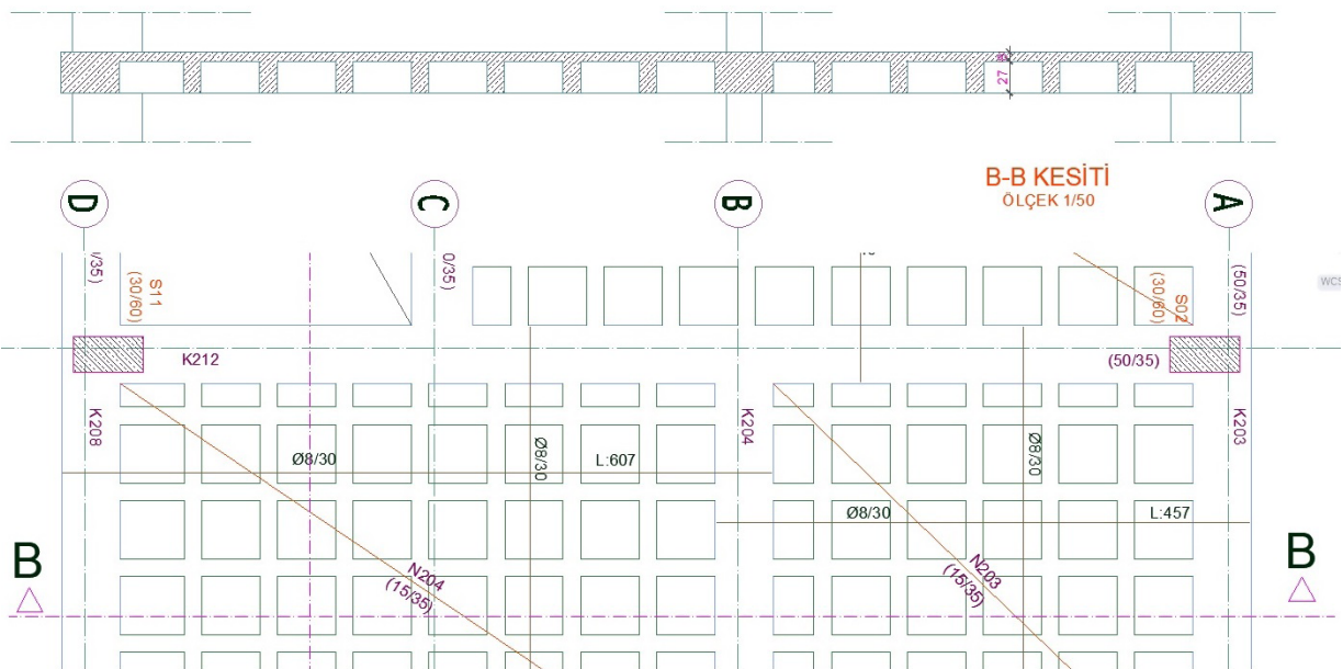
Çizim 13.10: Kaset döşeme B-B kesit çizimi
