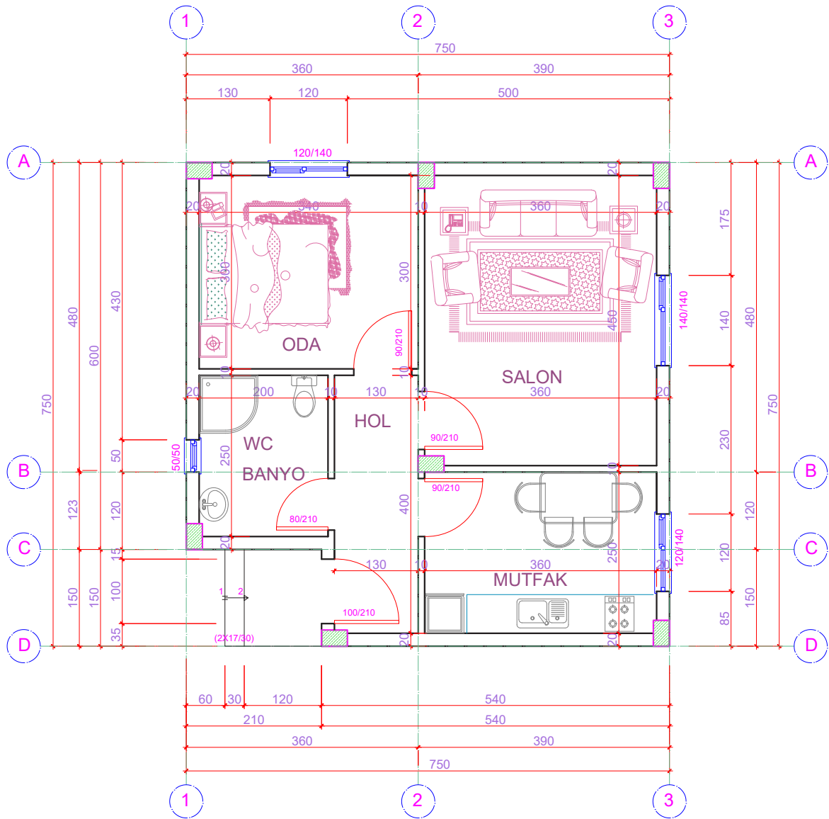
Çizim 4.5: Kat planı dış çizgisel ölçülendirme
