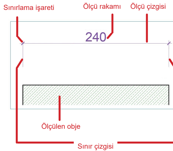
Görsel 4.3: Çizgisel ölçülendirme elemanları
