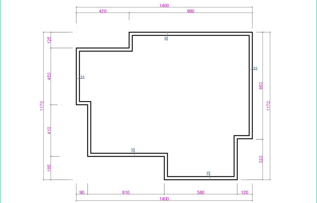
Çizim 5.7: Zemin kat planı dış duvarların çizimi
