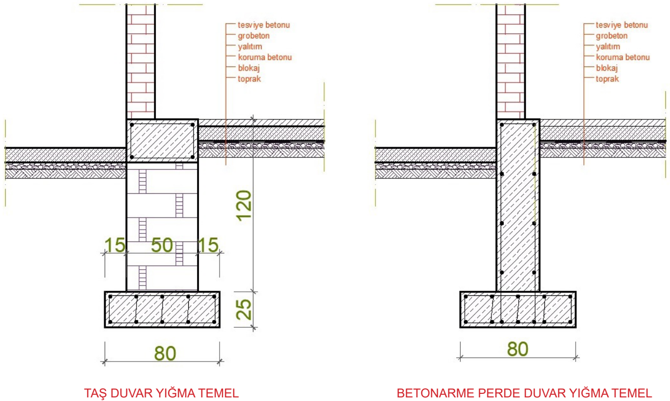
Görsel 8.1: Yığma temel planı çeşitleri
