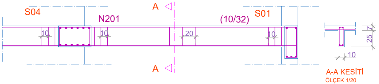
Çizim 15.3: Nervür kiriş görünüş ve kesit içerisine donatı çizimi
