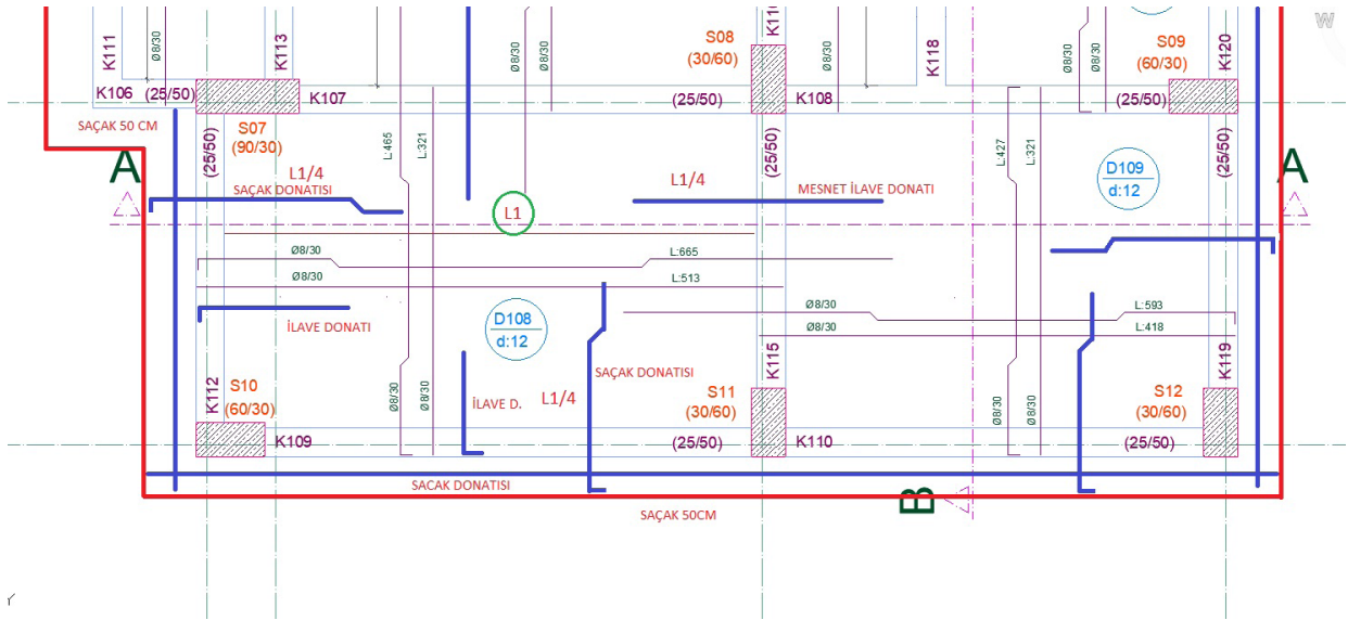
Görsel 11.3: Çatı döşeme planı üzerinde mesnet ve saçak ilave donatıları
