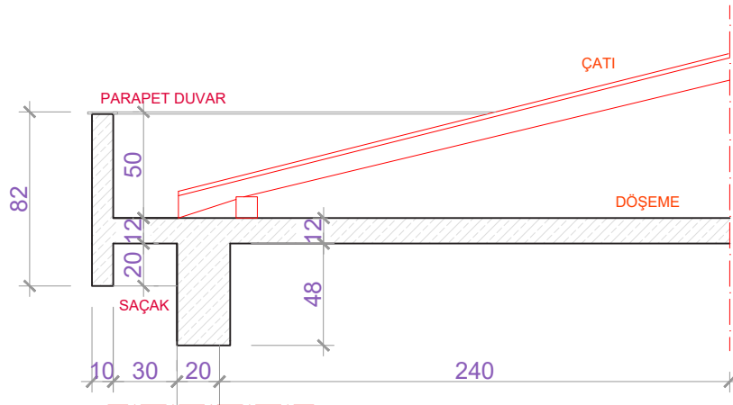
A-A KESİTİ
