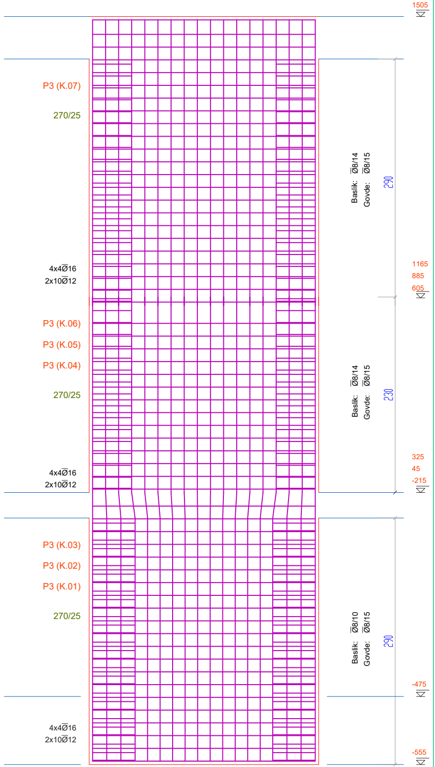
Çizim 16.12: Asansör perde duvarı çatıdan temele donatı detayı çizimi
