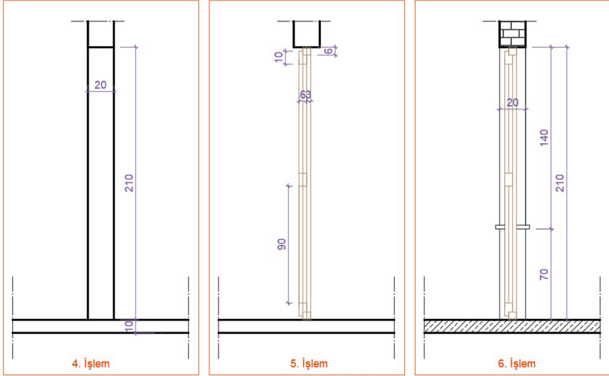
TOPAL KAPI KESİTİ
