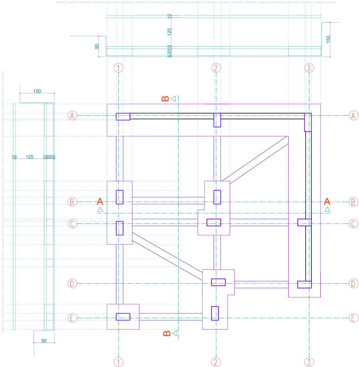
Çizim 8.23: Birleşik temel planı kesit taşıma çizgileri
