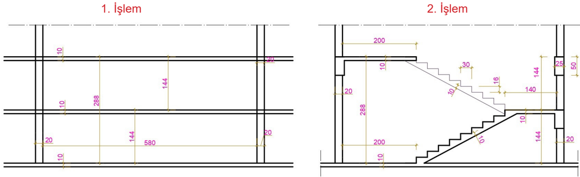
Çizim 3.9: Merdiven A-A kesit çizimi aşamaları
