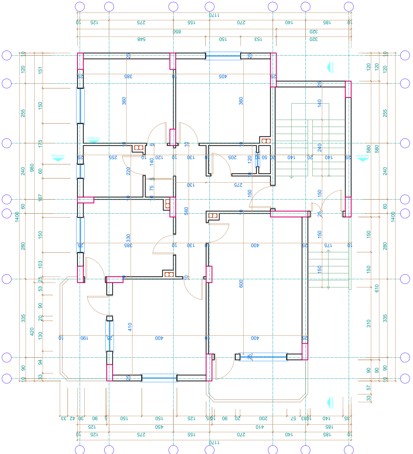
Çizim 6.2: Normal kat planı iç ve dış ölçülendirme
