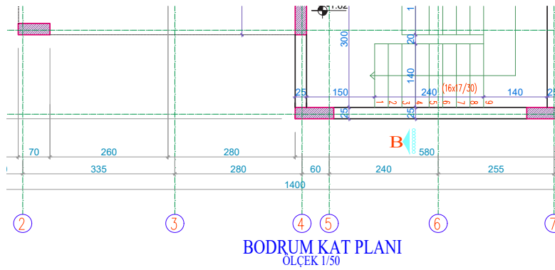
Çizim 7.5: Bodrum kat planı pafta ismi ve ölçek yazımı
