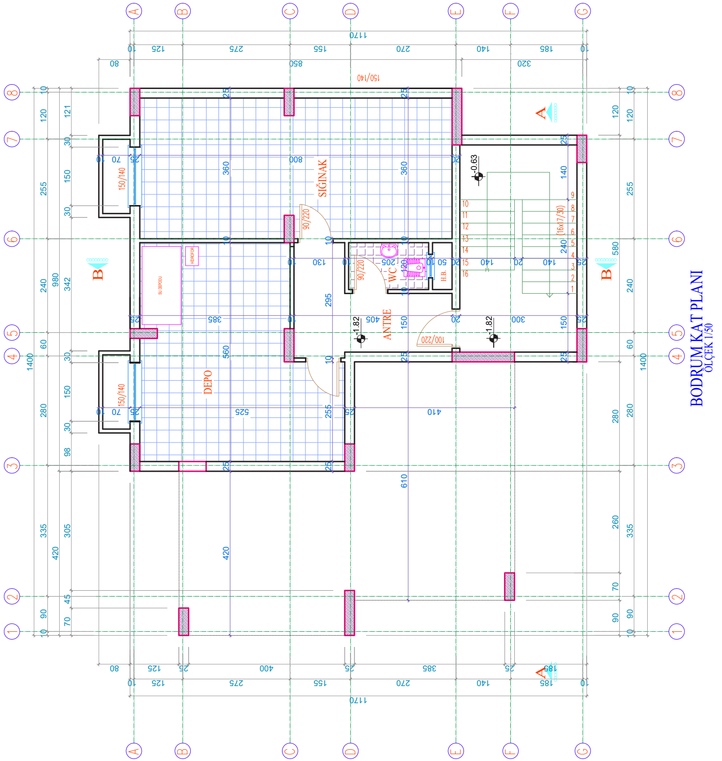
Çizim 7.8: Bodrum kat planı tarama çizimi
