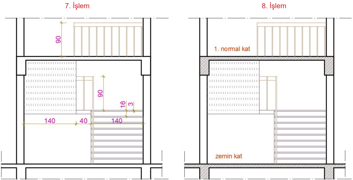
Çizim 3.11: Merdiven görünüş çizim aşamaları
