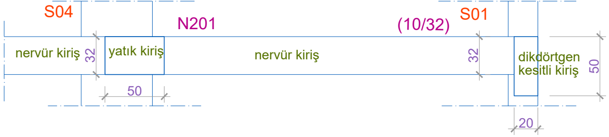
Çizim 15.2: Nervür kiriş görünüş çizimi
