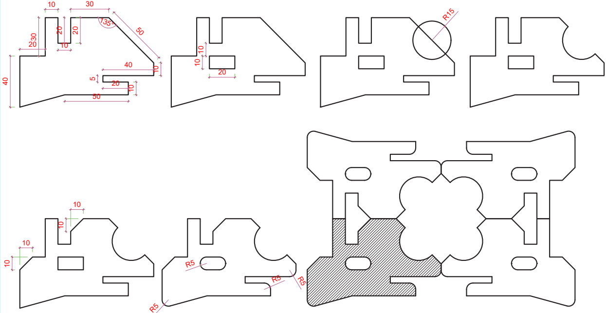
Çizim 2.2: İki boyutlu geometrik şeklin çizim aşamaları
