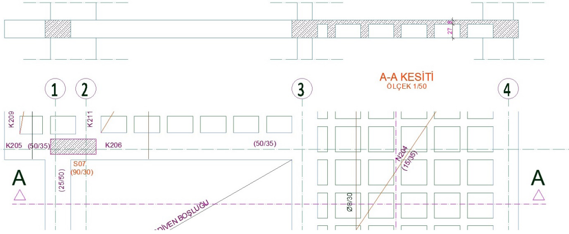
Çizim 13.9: Kaset döşeme A-A kesit çizimi
