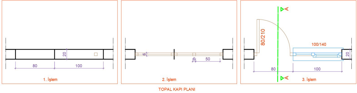
Çizim 2.16: Topal kapi plan çizim aşamaları
