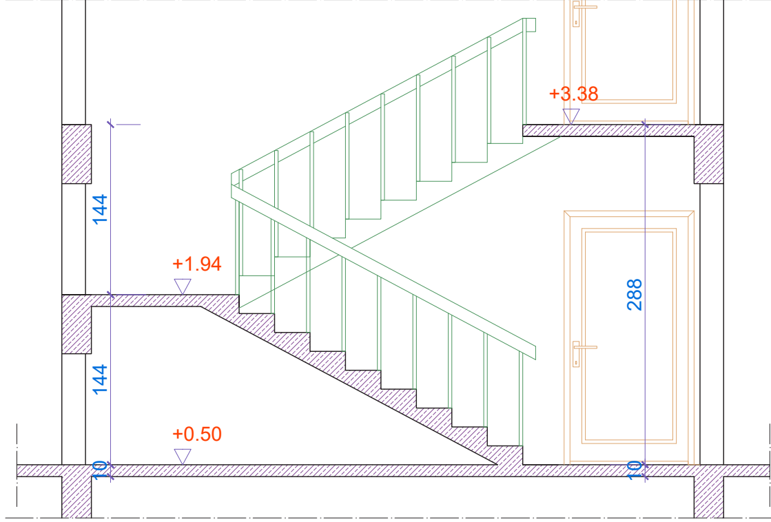
Çizim 16.6: Merdiven kesiti tarama ve ölçölendirme
