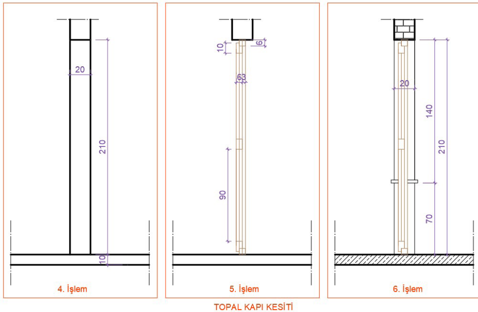
Çizim 2.17: Topal kapi kesit çizim aşamaları
