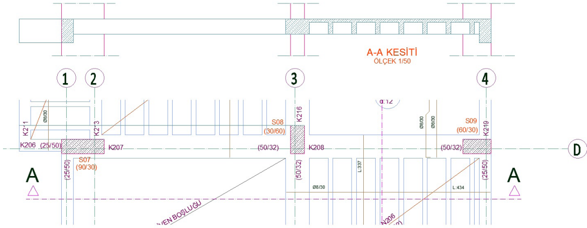
Çizim 12.7: Asmolen döşeme A-A kesit çizimi
