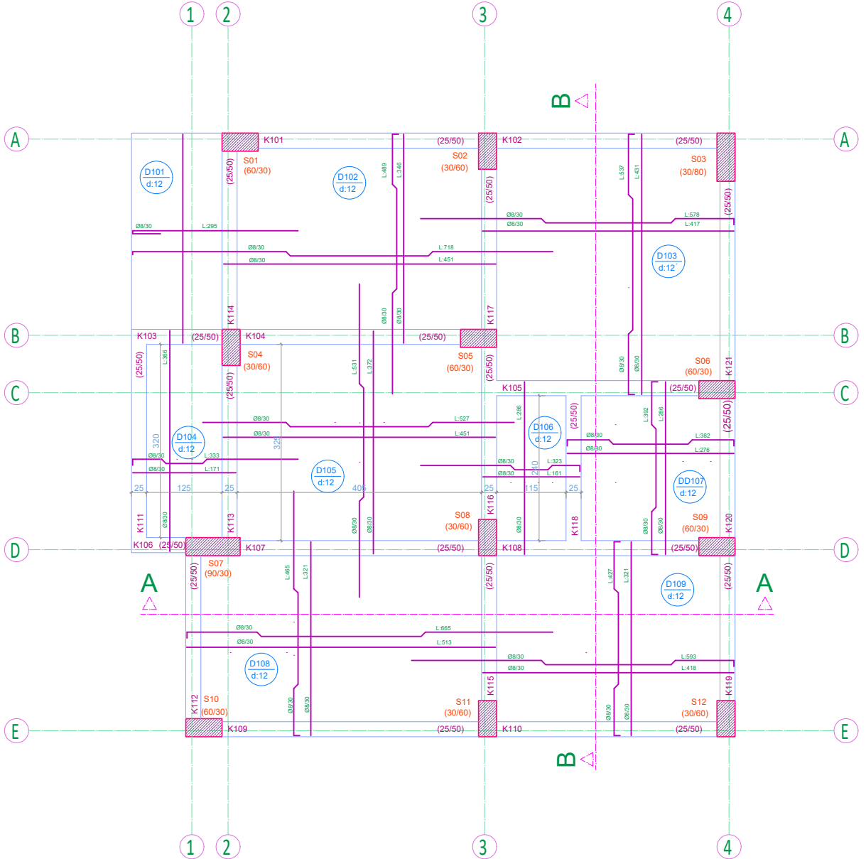
Çizim 11.10: Döşeme donatılarının çizimi ve hesaplanması
