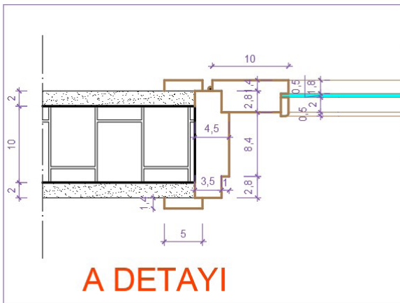
Çizim 2.8: Kapı A ve B detayı
