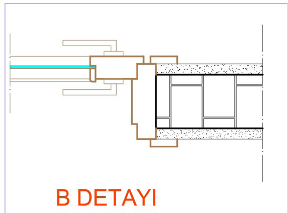
Çizim 2.8: Kapı A ve B detayı
