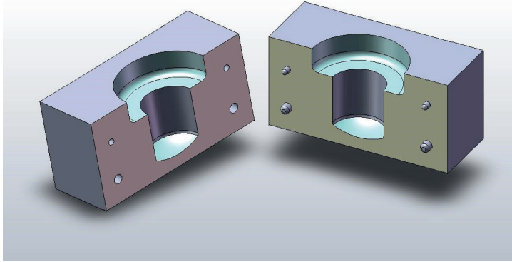
Görsel 6.13: Piston maçası
