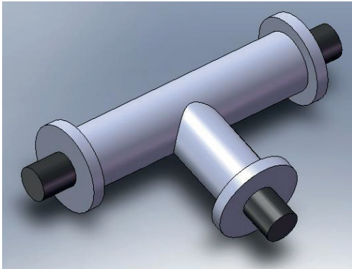
Görsel 4.5: Flaşlı "T" boru modeli
