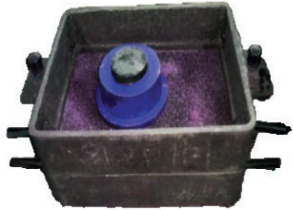
Görsel 6.17: Asma maçalı modelin ana derece üzerine konması
