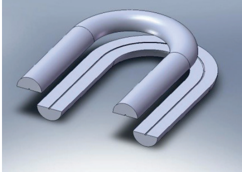
Görsel 4.15: Yarım "U" maçalar
