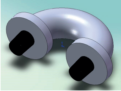
Görsel 3.4: Flanşlı "U" boru modeli
