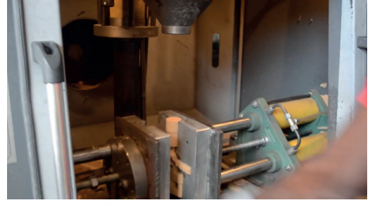
Görsel 5.9: Maça sandığının açılması
