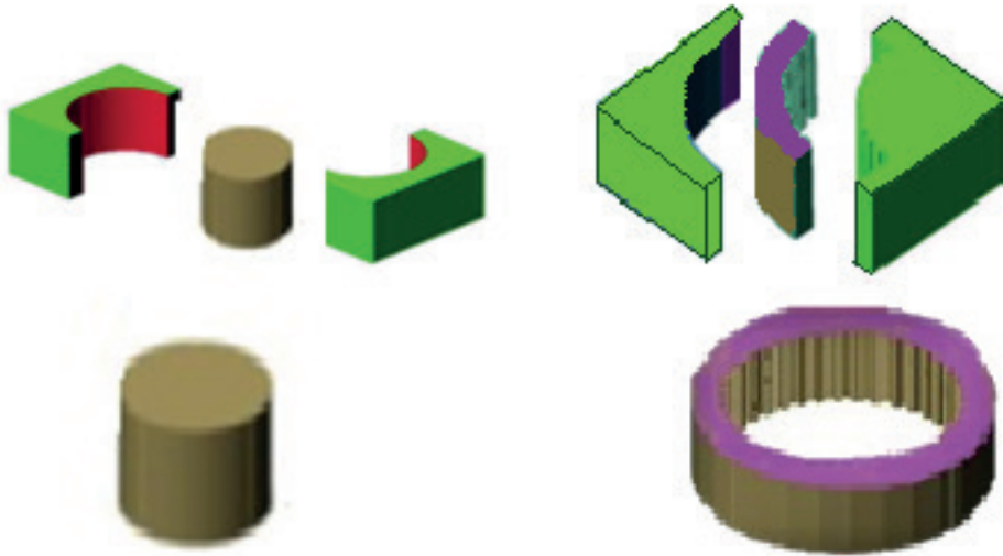
Görsel 6.25: Kütük maça sandıkları ve maçalar
