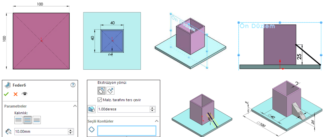
Görsel 2.32: Kırtı modele destek yapma
