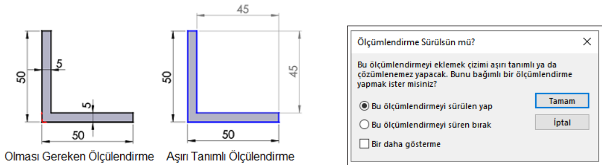
Görsel 1.62: Aşırı tanımlı ölçümlendirme
