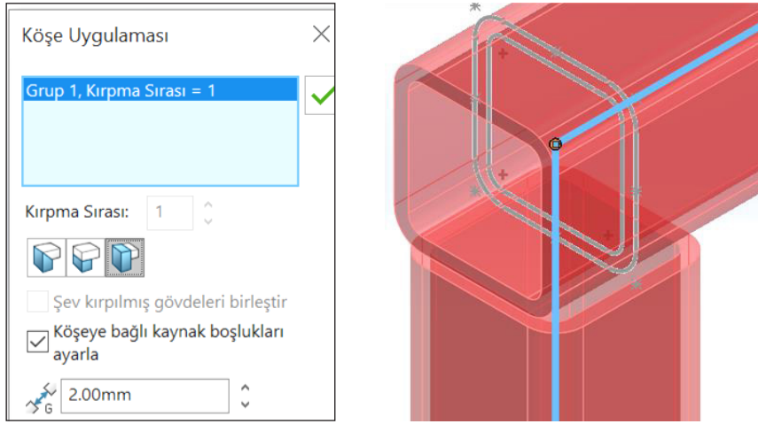
Görsel 4.30: Köşe uygulaması
