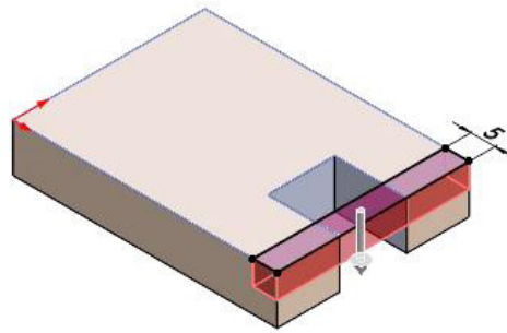
Görsel 2.18: Ekstrüzyon ile kes koşulları
