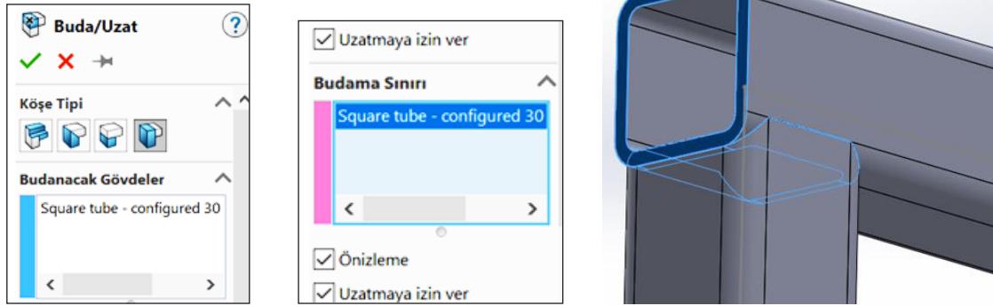
Görsel 4.31: Profili buda /uzat
