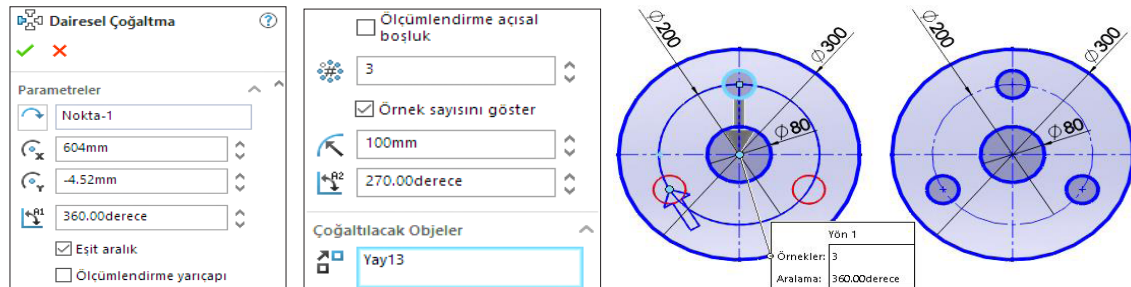
Görsel 1.41: Dairesel çizimi çoğaltma
