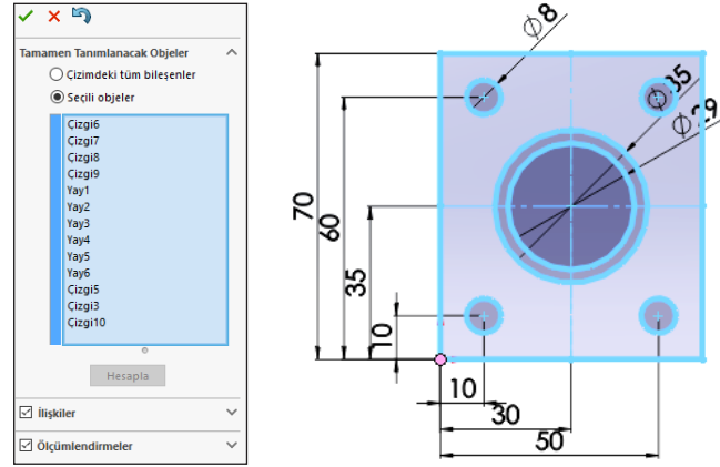
Görsel 1.59: Objeler seçiliyken otomatik ölçümlendirme
