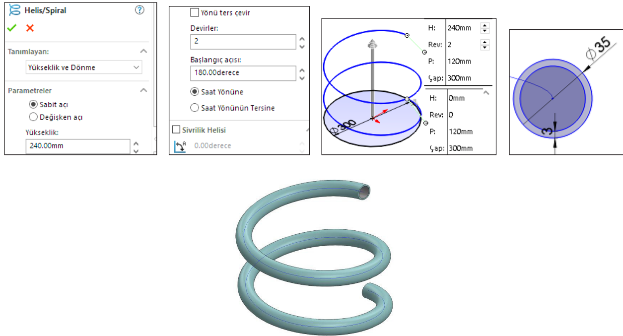
Görsel 2.15: Helis ile süpürerek katı oluşturma
