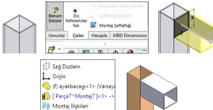
Görsel 4.12: Montajda yeni parça ekleme
