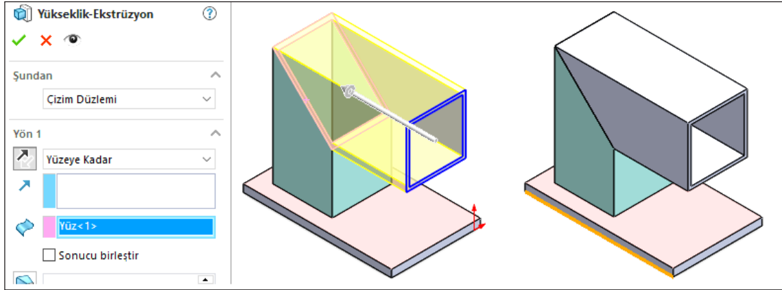
Görsel 2.5: Yüzeye kadar koşulu
