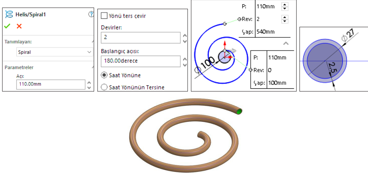
Görsel 2.14: Spiral ile süpürerek katı oluşturma
