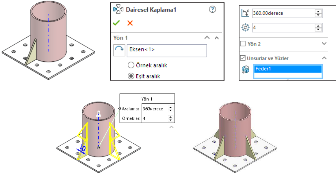
Görsel 2.37: Katı modeli dairesel çoğaltma
