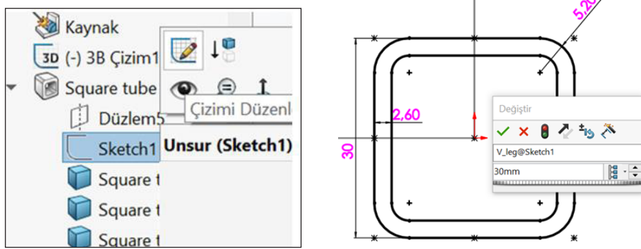
Görsel 4.36: Profil taslağı düzenleme
