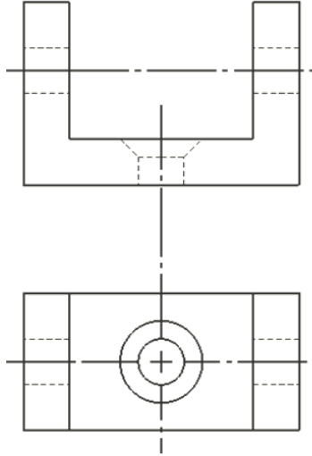
Görsel 5.15: Üst görünüm
