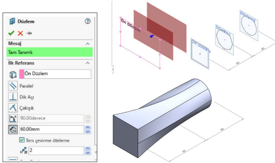
Görsel 2.16: Farklı profiller ile katı oluşturma
