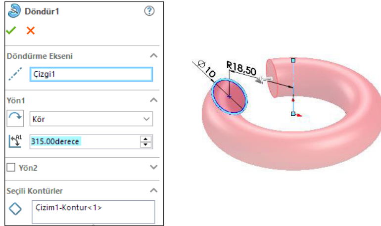
Görsel 2.12: Açılı döndürerek katı oluşturma
