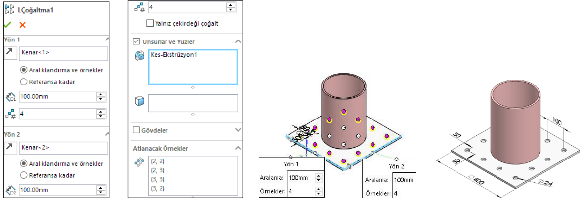
Görsel 2.36: Katı modeli doğrusal çoğaltma
