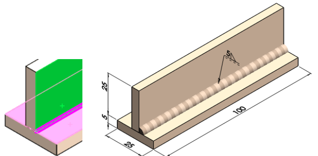
Görsel 4.26: Kaynak parçası komutu ile yapılan alın ve iç köşe kaynakları
