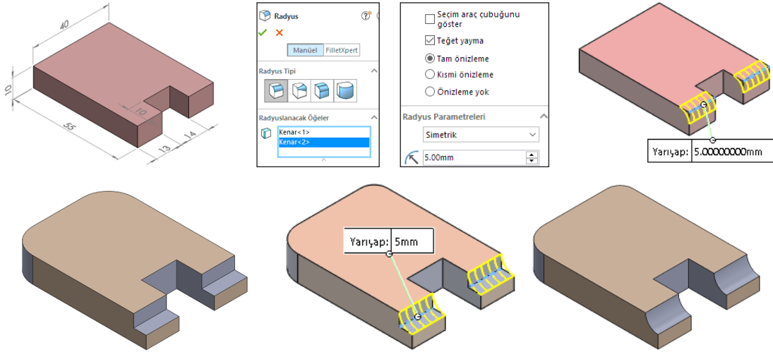
Görsel 2.23: İçe ve dışı yuvarlatma
