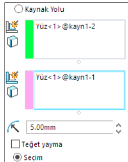
Görsel 4.26: Kaynak parçası komutu ile yapılan alın ve iç köşe kaynakları
