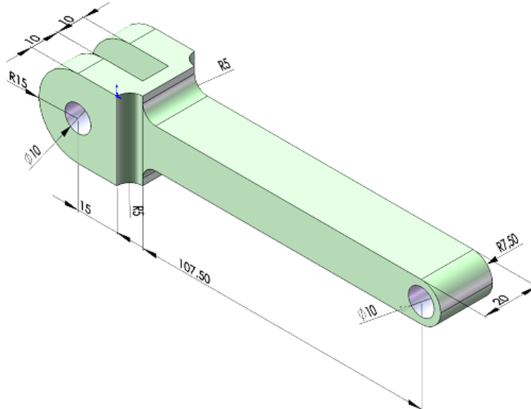
Görsel 2.39: Katı modelin ölçümlendirilmesi
