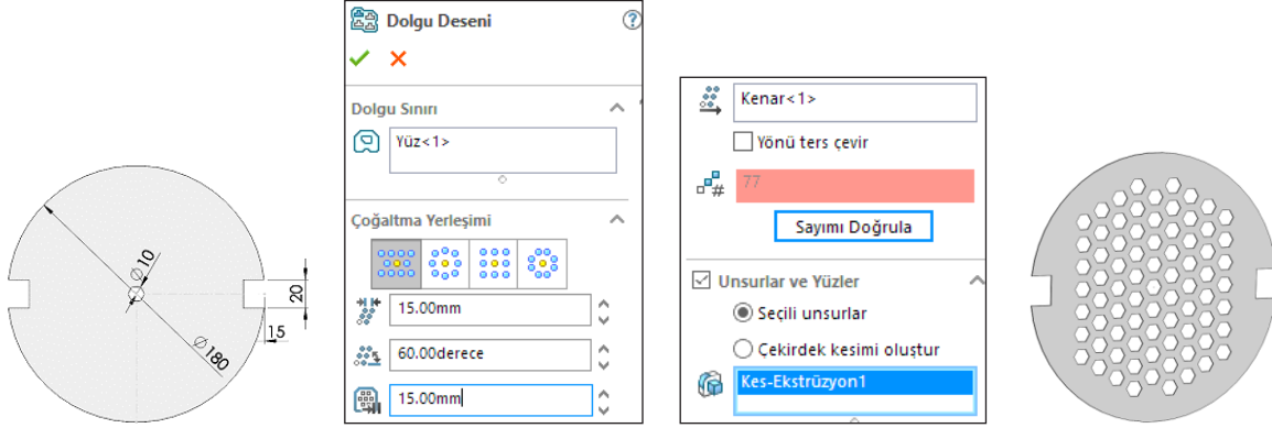
Görsel 2.38: Katı modeli doldurarak çoğaltma
