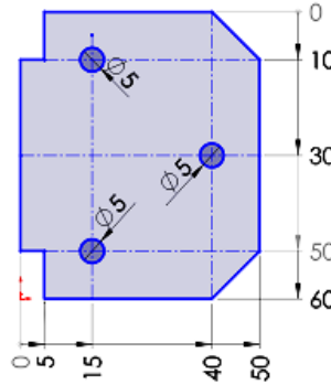
Görsel 1.57: Yatay ve dikey ordinat ölçümlendirme
