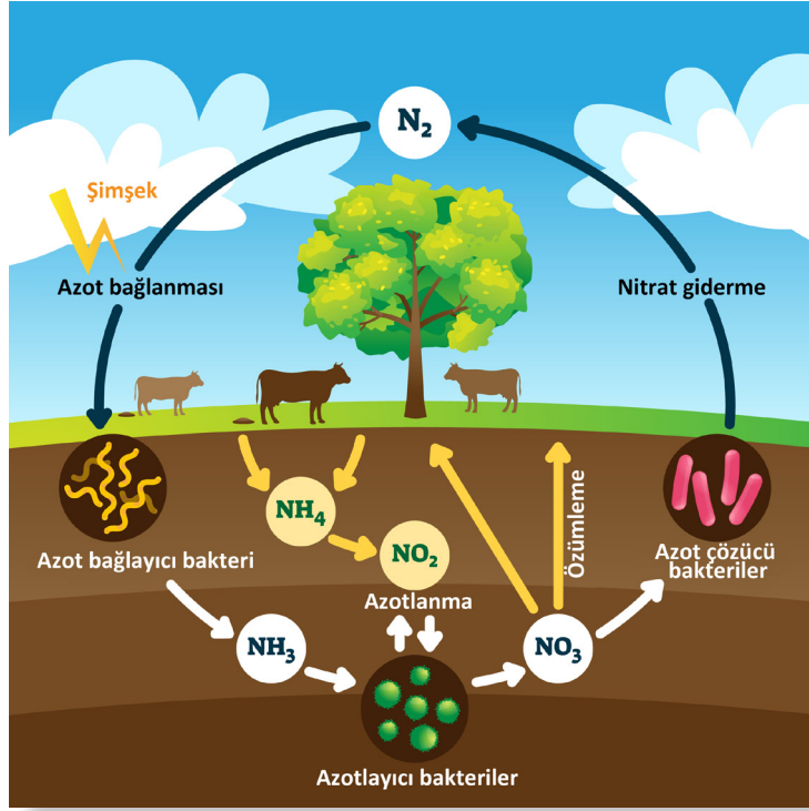
Görsel 2.11: Azot (nitrojen) döngüsü
