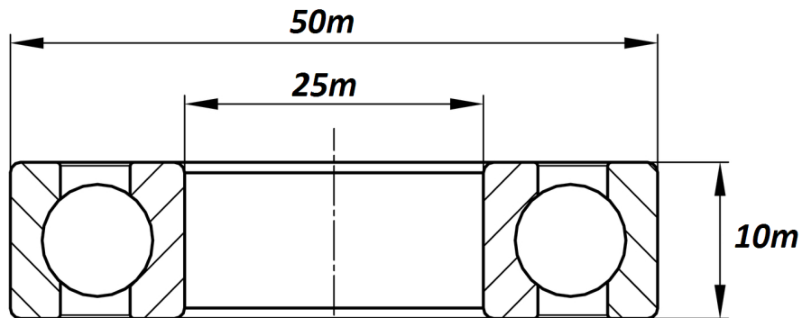
Görsel 1.77: Gerçek ölçüleri verilmiş bir demir konstrüksiyon bağlantı bloğu
