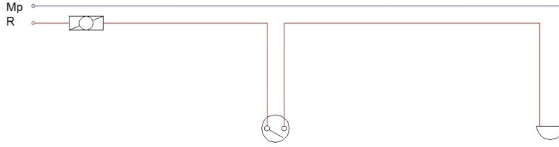
ADİ ANAHTAR TESİSATI AÇIK ŞEMA
