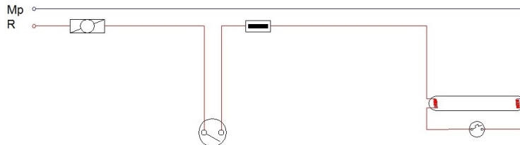
ADİ ANAHTARLI FLORESAN TESİSATI KAPALI ŞEMA
