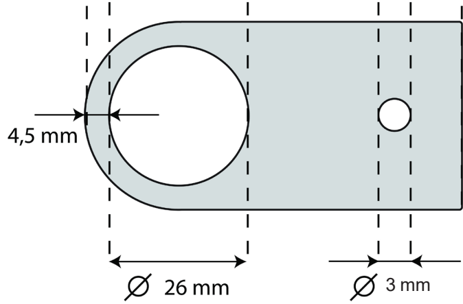
Görsel 1.75: 2:1 büyültme ölçeği ile çizilmiş parça
