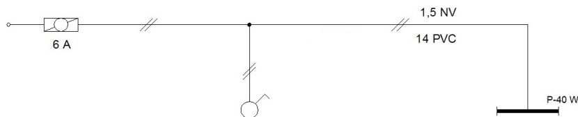
ADİ ANAHTARLI FLORESAN TESİSATI KAPALI ŞEMA
