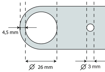
Görsel 1.74: Gerçek ölçekle çizilmiş parça
