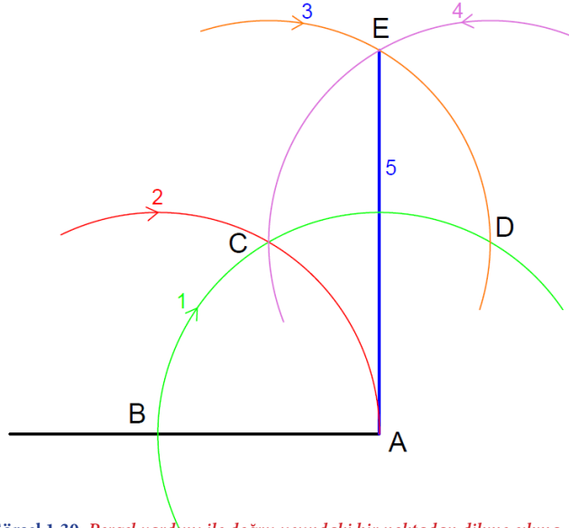
Görsel 1.30: Pergel yardımı ile doğru ucundaki bir noktadan dikme çıkma
