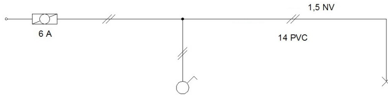
ADİ ANAHTAR TESİSATI KAPALI ŞEMA
