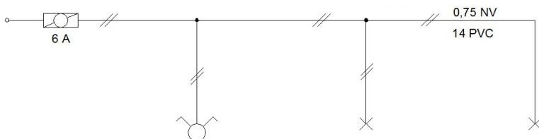
ADİ ANAHTARLI FLORESAN TESİSATI AÇIK ŞEMA
