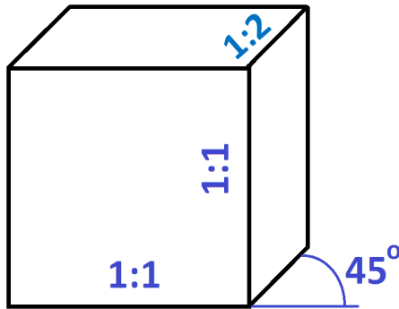
Görsel 1.60: Kabinet perspektif
