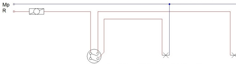
KOMÜTATÖR ANAHTAR TESİSATI AÇIK ŞEMA
