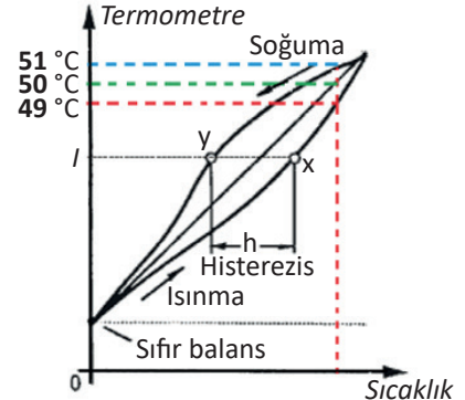
Grafik 1.5. Histerezis grafiği
