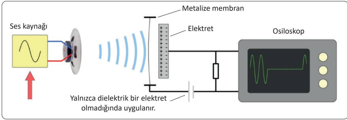
Şekil 1.36: Ses dalgalarının kapasitif etki ile voltaj üretmesi
