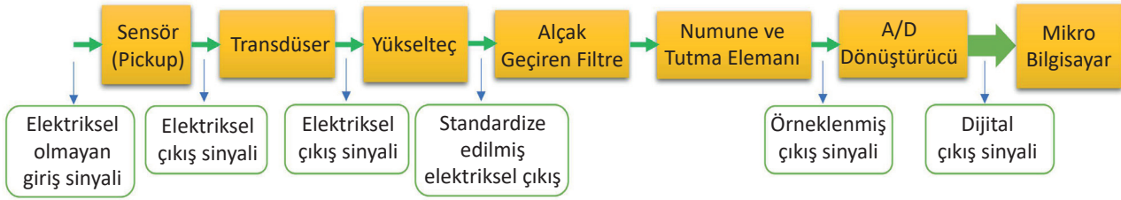
Şekil 1.3: Standart bir ölçüm sistemi blok şeması
