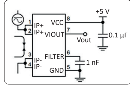
b) ACS712 akım sensörü şeması
