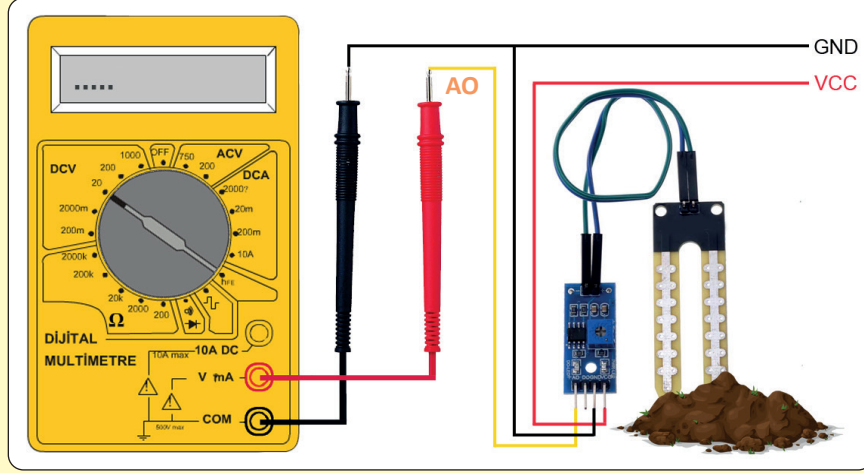
Şekil 2.30: Toprak sensörünün sağlamlık testi ve çalışması
