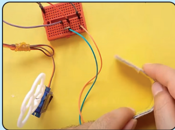
Fotoğraf 1.28: Esnek (flex) sensör
