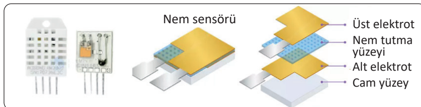
Şekil 2.19: DHT11 iç yapısı
