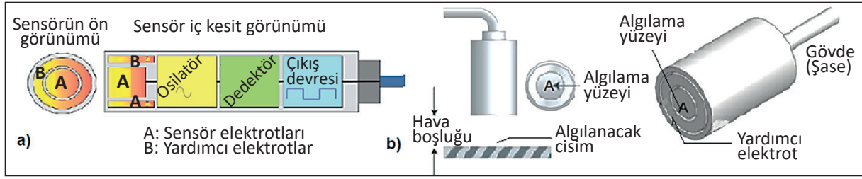
Şekil 2.21: a, b) Kapasitif PNP Proximity (yakınlık) sensörünün yapısı ve blok şeması
