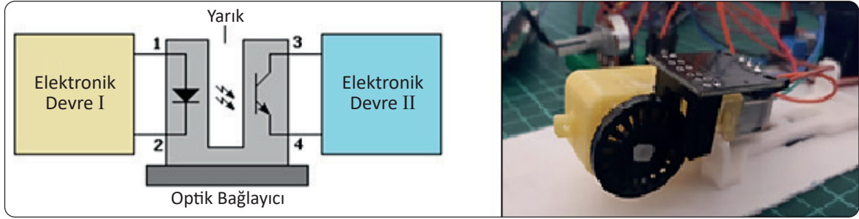
Şekil 2.45: Kızılötesi (IR) oluklu optik hız ölçüm sensörü çalışması
