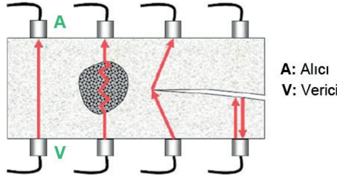
Şekil 2.4: Ultrasonik dalgalarla beton kalitesinin tespit edilmesi
