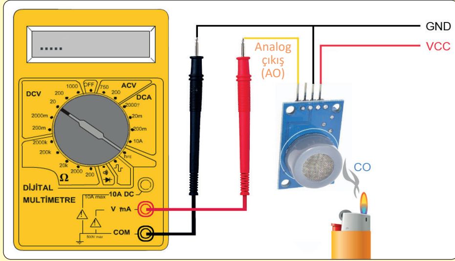
Şekil 2.61: Karbonmonoksit (CO) sensörünün sağamlık testi ve çalışması
