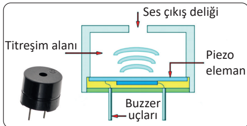
Şekil 1.29: Piezo buzzer ve yapısı
