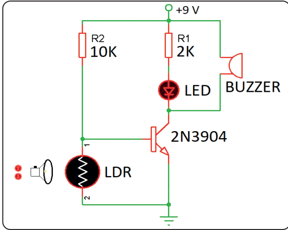
Şekil 1.58: Devre şeması
