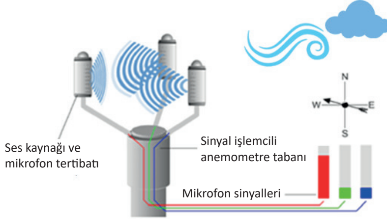
Şekil 1.15: Sonik rüzgar sensörü (anemometre)
