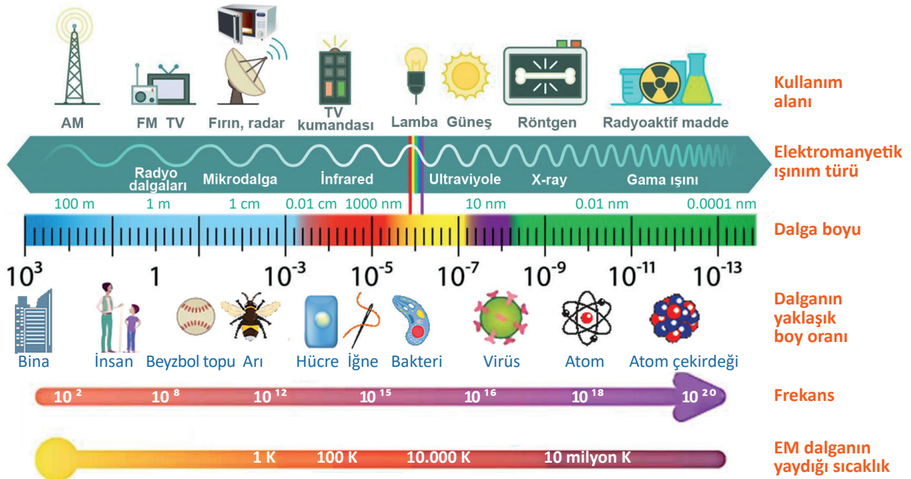
Şekil 2.37: Elektromanyetik ışık spektrumu
