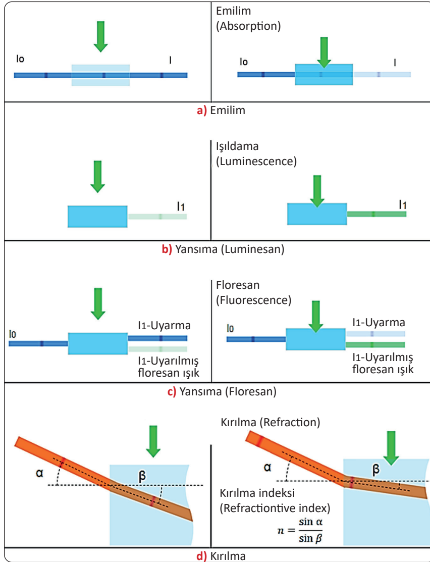
Şekil 2.35: a, b, c, d) Cisimlerin optik özelliklerine göre davranışları (emilme, yansıma ve kırılma)
