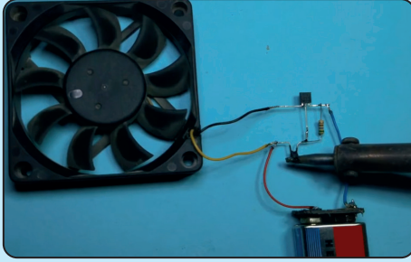
Fotoğraf 1.29: Devrenin çalıştırılması
