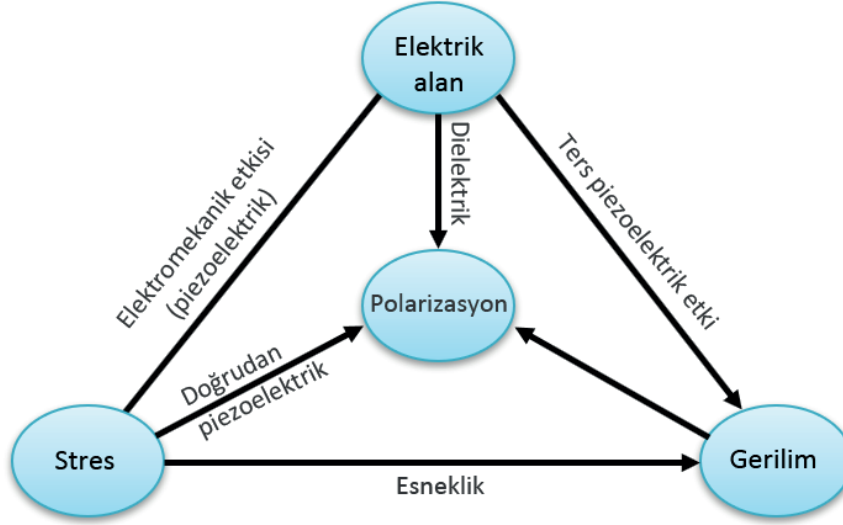
Şekil 1.30: Piezoelektrik etkileşim (elastik özellikler, polarizasyon, elektrik alan)
