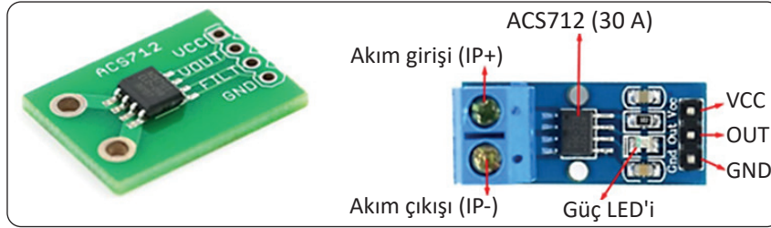
Şekil 2.33: ACS712 akım sensörünün görüntü ve pin bağlantı şeması
