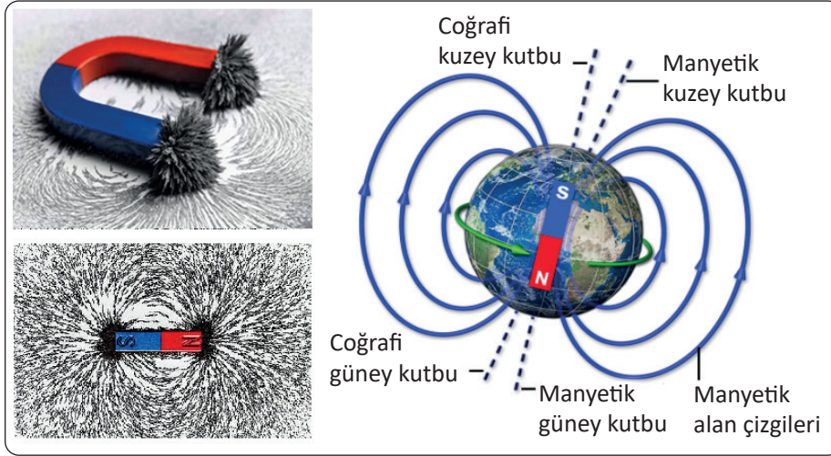
Şekil 1.48: Manyetik kuvvet çizgilerinin oluşumu
