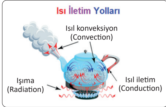
Şekil 2.16: Isı iletim yolları
