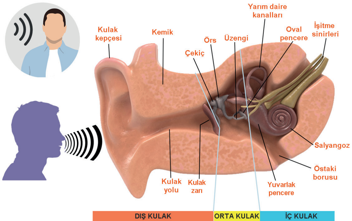
Şekil 1.22: Kulakta işitmenin oluşumu
