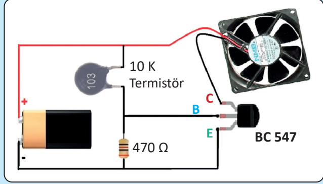
Şekil 1.44: Devre şeması (Görünüşü)
