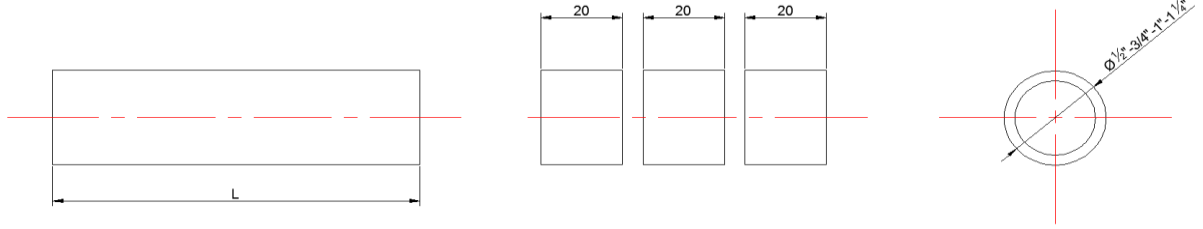
Görsel4.9: Kesilecek boru ölçüleri
