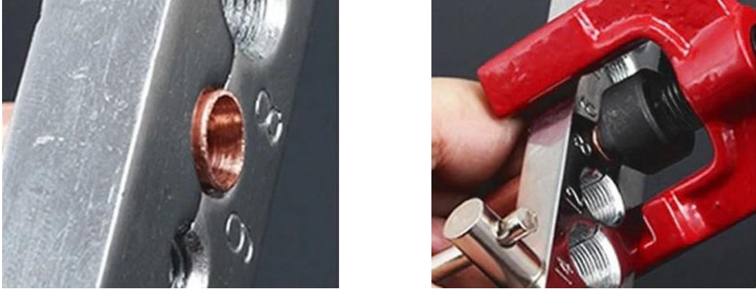
Görsel 6.14: Havşa yapım aşamaları
