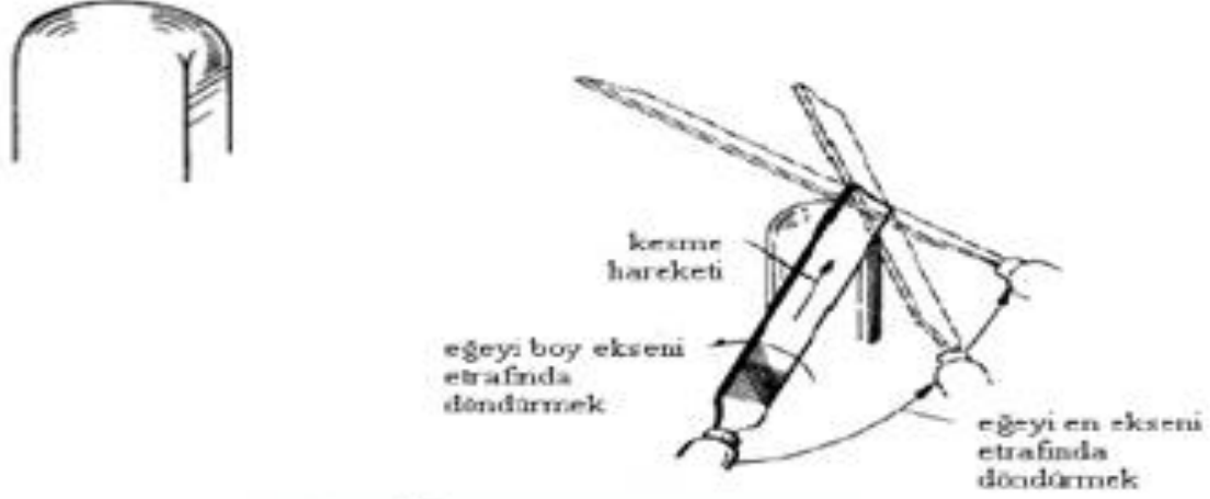
Görsel 3.15: Küresel yüzeylerin eğelenmesi
