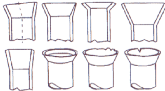
Görsel 6.15: Hatalı havşa örnekleri
