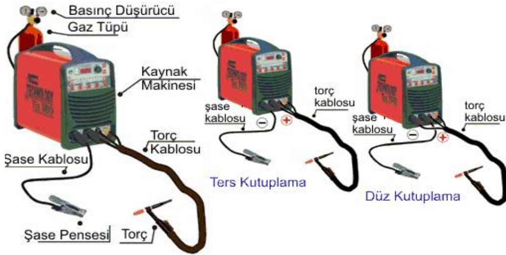
Görsel 13.10: TİG kaynak makinesi kutuplama
