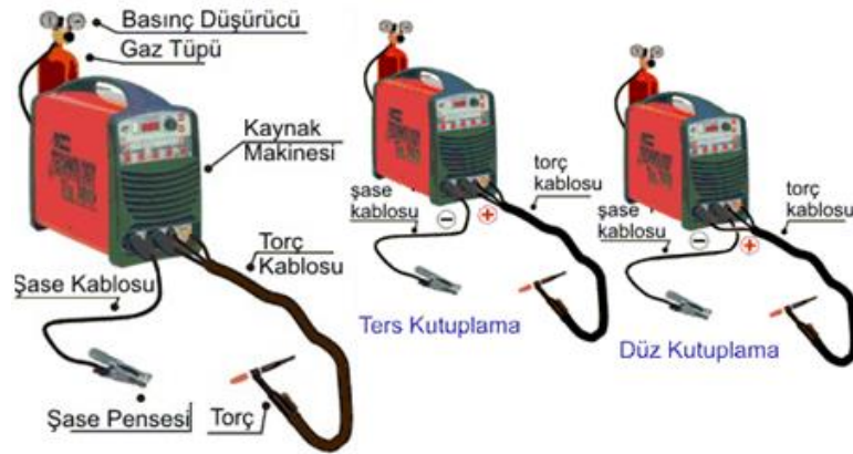
Görsel 13.6:TİG kaynak makinesi kutuplama
