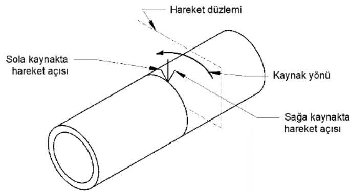
Görsel 12.28: Hareket düzlemi üzerinde çalışma açısı
