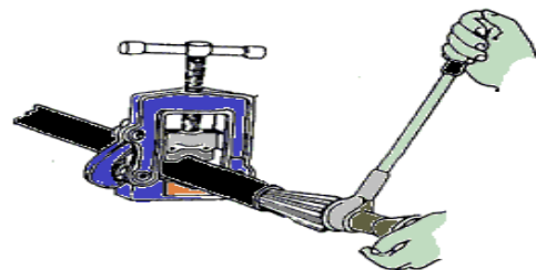
Görsel4.8: Rayba ile çapak temizleme
