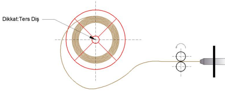
Görsel 12.16: Makaranın yuvaya oturtulmasında oluşacak hatalar
