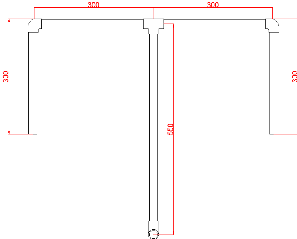
Görsel 5.11: Polipropilen boru kaynak bağlantısı
