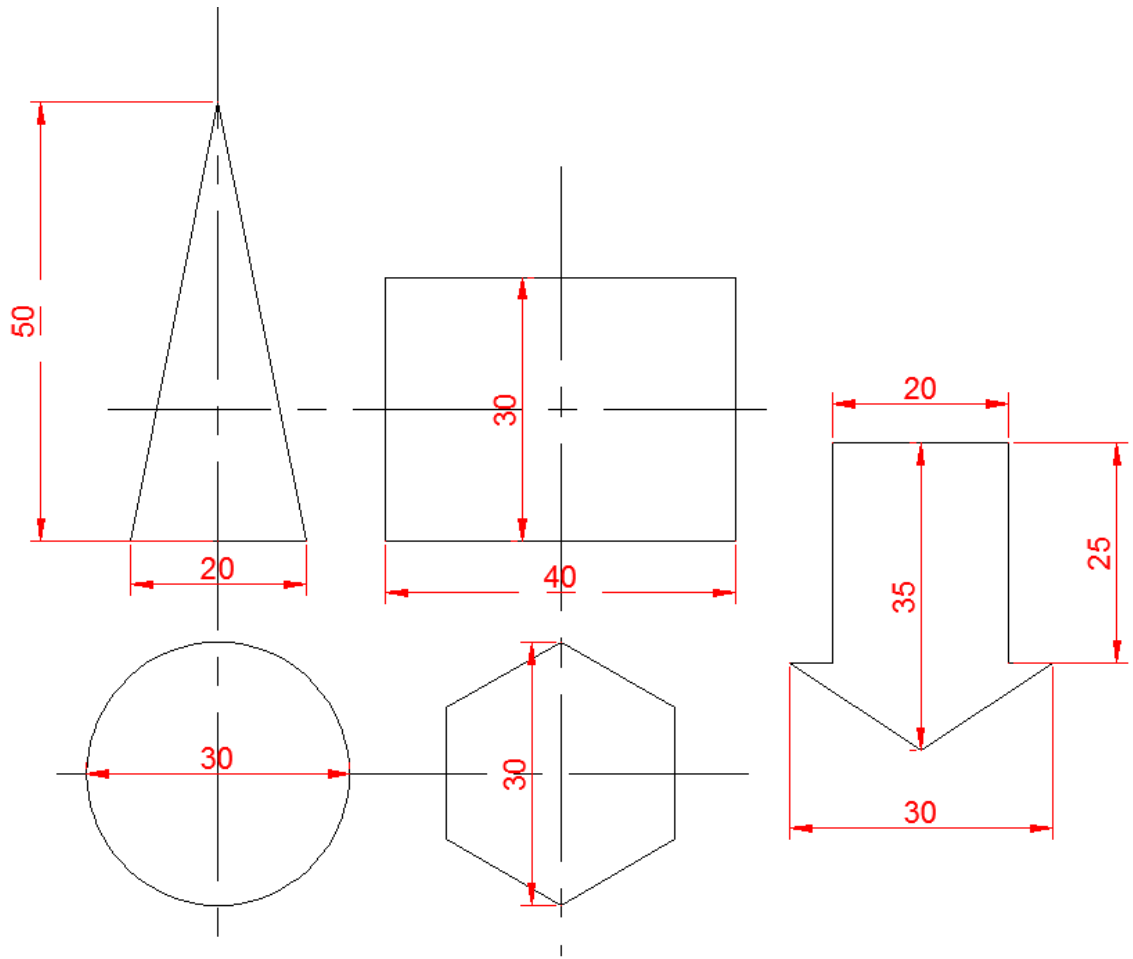
Görsel 2.28: Sac üzerine markalama çizimleri
