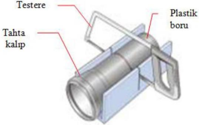
Görsel 5.14: PVCboru kesme kalıbı
