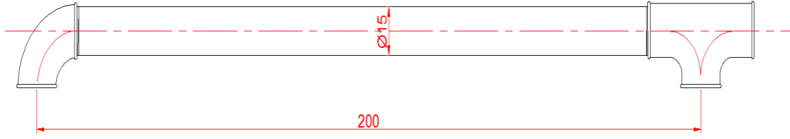
Görsel 4.35: Fittings sıkılmış boru ölçüsü
