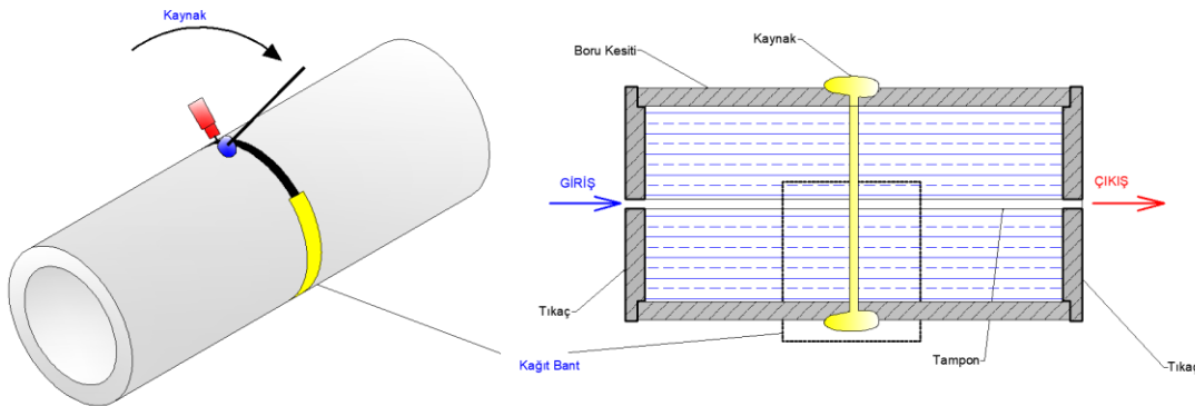
Görsel 13.13: Tampon gaz kullanılarak yapılan boru kaynağı
