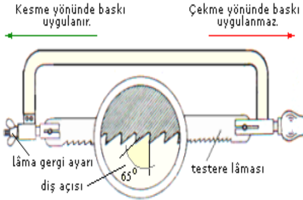
Görsel 4.2: Testere laması takma yönü
