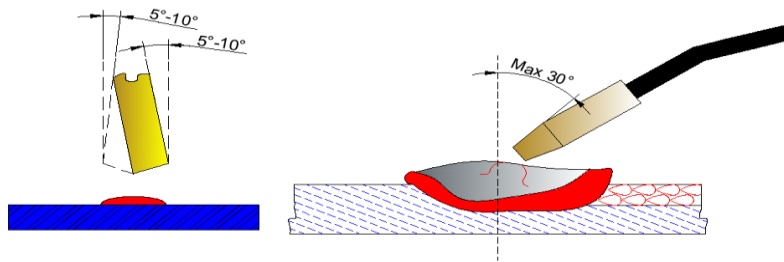
Görsel 12.14: Torcu iş parçasına göre konumu
