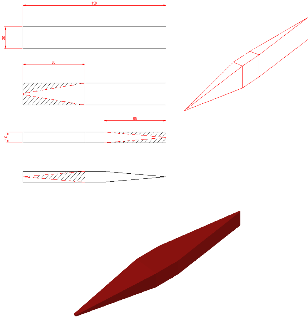
Görsel 3.18: Kaynakçı çekici ölçüleri
