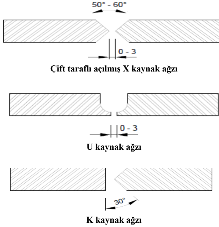
Görsel 9.1: Kaynak ağzı çeşitleri
