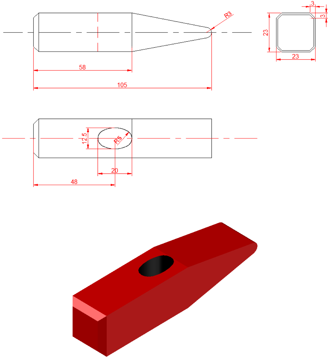
Görsel 3.17: Tesviyeci çekici ölçüleri
