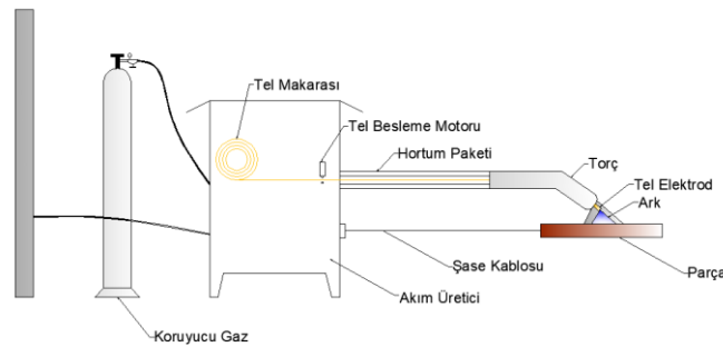
Görsel 12.2: MİG-MAGkaynak donanımları
