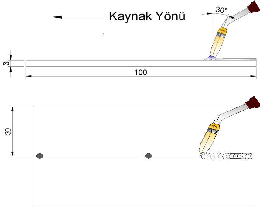
Görsel 12.19: Kaynak yapılacak metalin ölçüsü ve kaynak yönü
