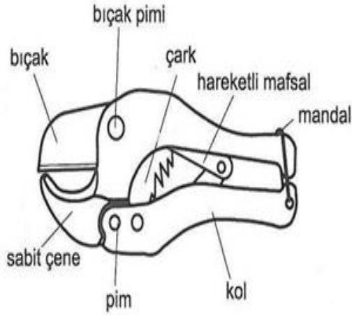
Görsel 5.3: Polipropilen boru kesme makası
