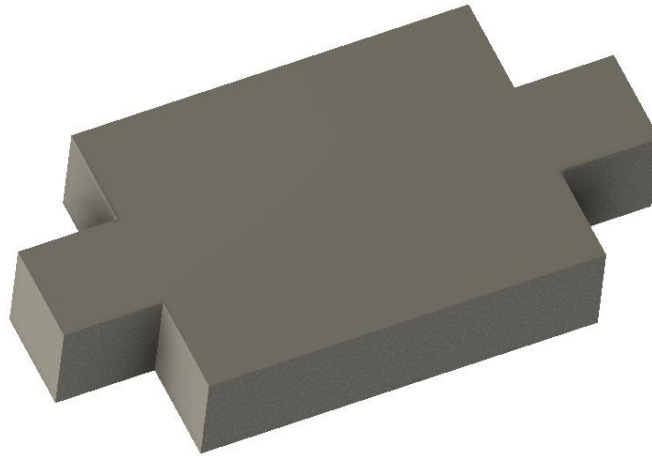
Görsel 2.34: Kesim parçası ölçüleri
