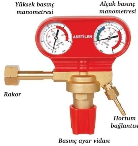
Görsel 8.3: Asetilen basınç düşürücüsü
