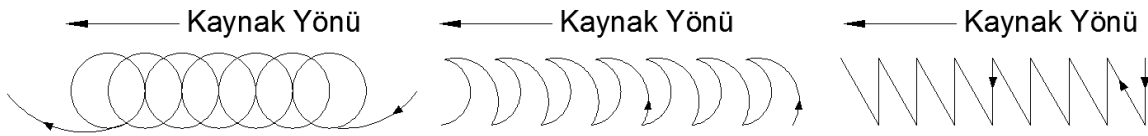
Görsel 12.25: Boru kaynağında torca verilecek hareketler
