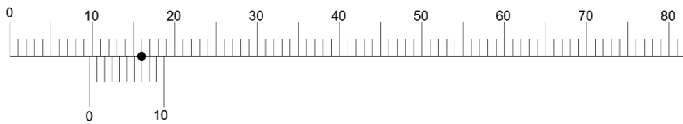
Görsel 2.8: 1/10'luk kumpasta belirlenmiş ölçü
