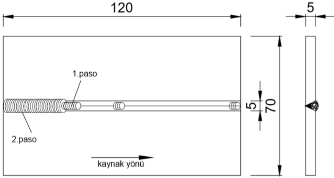
Görsel 9.8: Kaynak uygulaması
