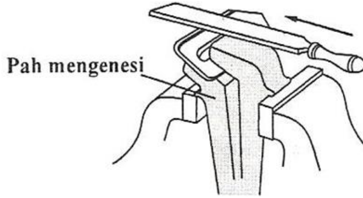
Görsel 3.13:Pah Kırma Mengenesi
