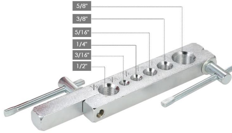
Görsel 6.17: Havşa mengenesine uygun boru çapları
