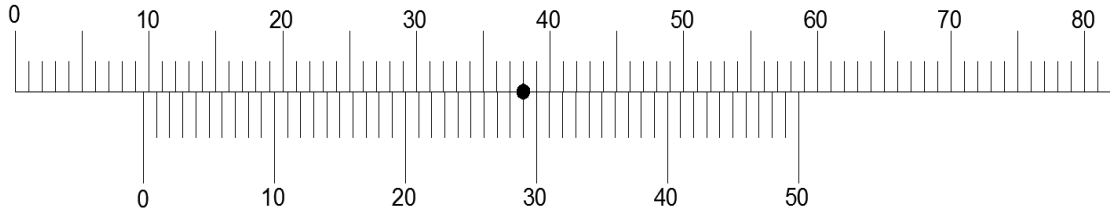
Görsel 2.12: 1/50'lik kumpasta belirlenmiş ölçü
