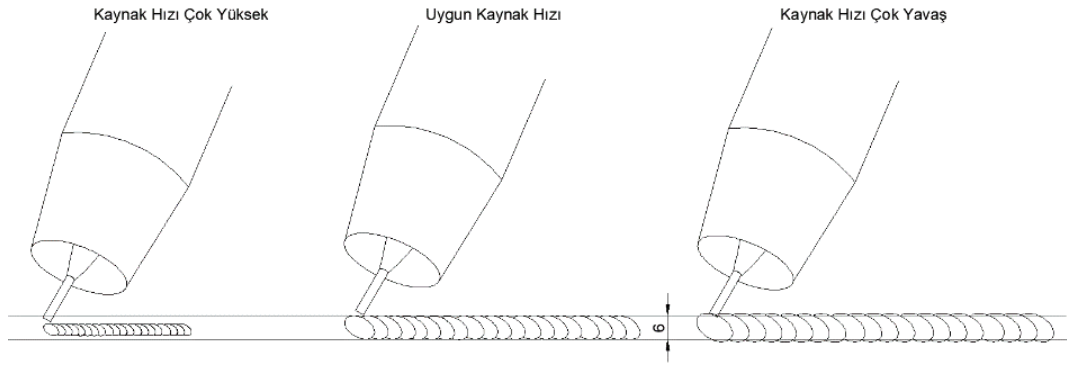
Görsel 12.30: Kaynak konumlarının parça üzerine etkileri
