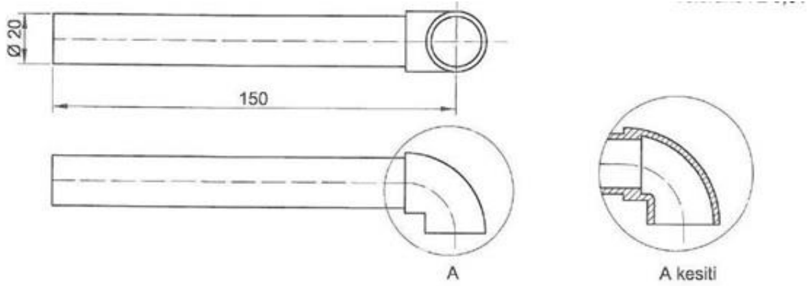
Görsel 5.10: Polipropilen boru kaynak işlemi için boru kesiti
