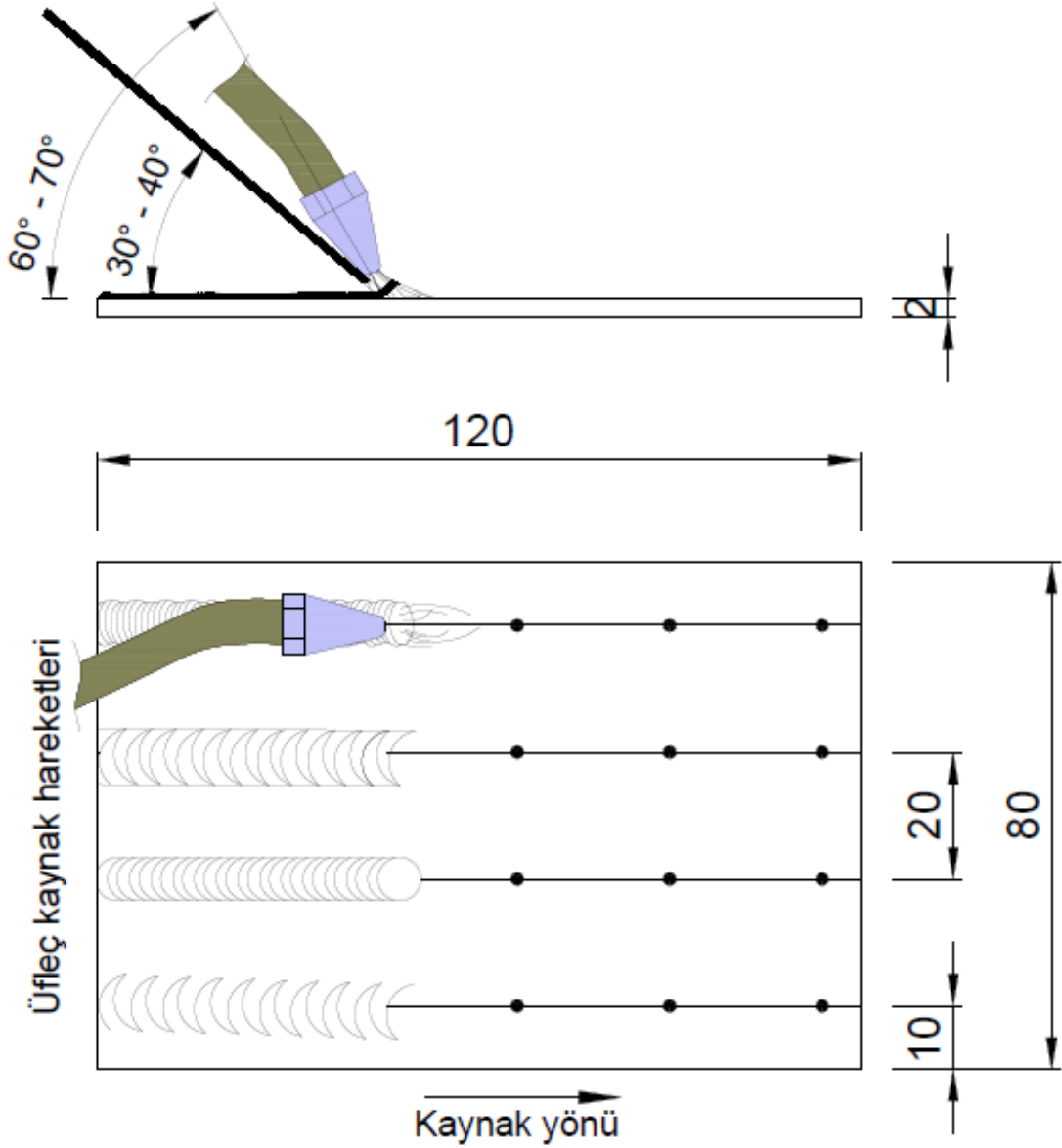
Görsel 9.6: Kaynak uygulaması
