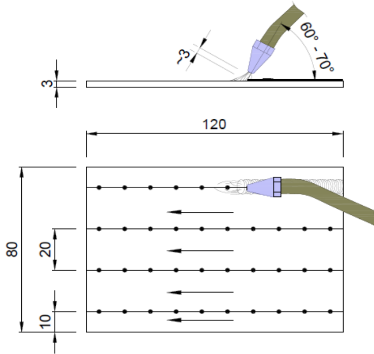
Görsel 9.3: Kaynak uygulaması
