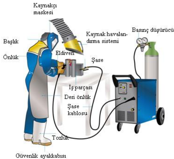
Görsel 13.16: TIG kaynağında güvenlik ekipmanı
