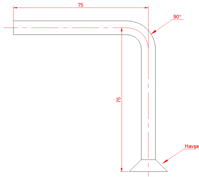
Görsel 6.23: Bakır boru birleştirme çizimi
