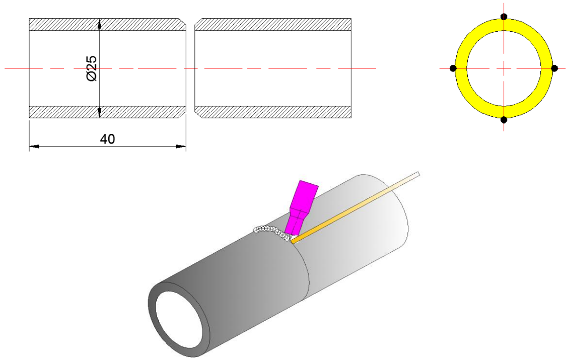
Görsel 13.21:Kaynak yapılacak borunun ölçüleri
