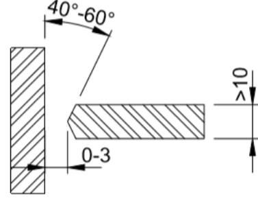
Yarım çift yönlü V kaynak ağızı
