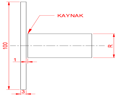
Görsel 12.22: Parçanın kaynağa hazırlanması
