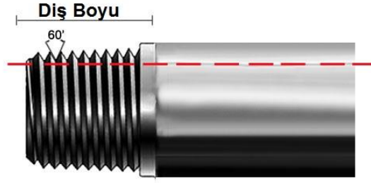
Görsel 4.11: Çelik boru vida bölümleri
