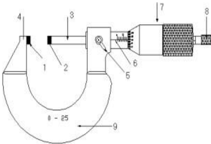
Görsel 2.13: Mikrometre gövde ve yapısı
