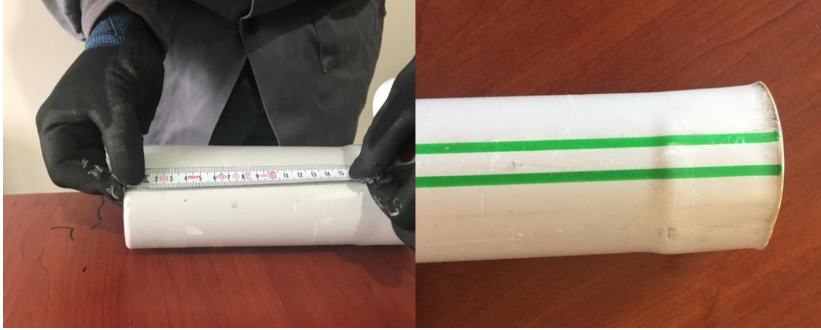
Görsel 5.24 Muf açılmış boruyu birleştirme aşamaları
