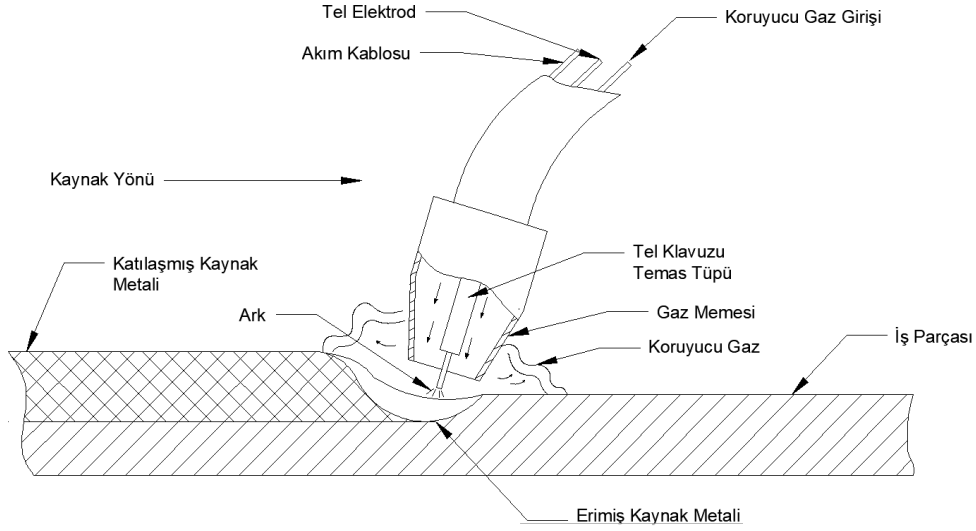
Görsel 12.31: MİG-MAG kaynak tekniği
