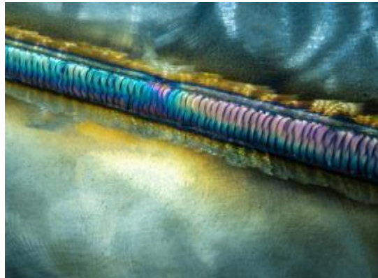
Görsel 13.20: Kaynak dikiş örneği
