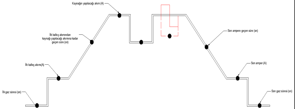
Görsel 13.12: TİG kaynak makinesi parametre şeması
