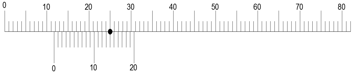
Görsel 2.10: 1/20'lik kumpasta belirlenmiş ölçü
