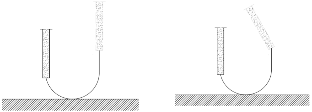
Vurarak ark başlatma
