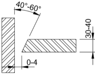
K kaynak ağızı
