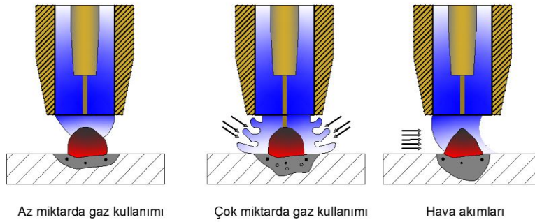
Görsel 12.18: Kaynak hatası oluşum sebepleri
