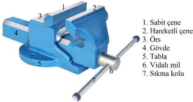
Görsel 3.1: Tesviyeci mengenesi ve kısımları
