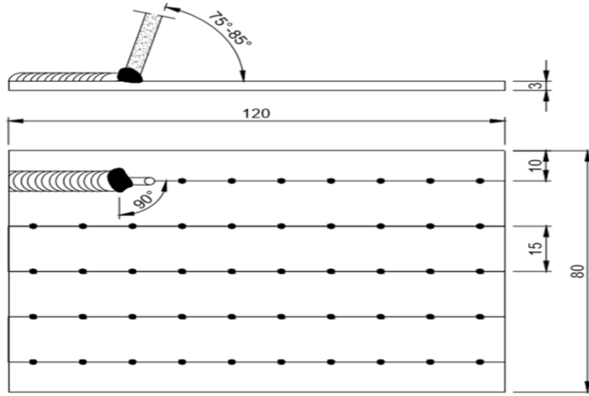
Görsel 11.4: Kaynak işlemi
