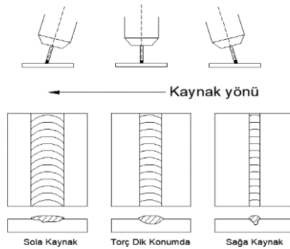
Görsel 12.15: Kaynak konumlarının parça üzerine etkileri
