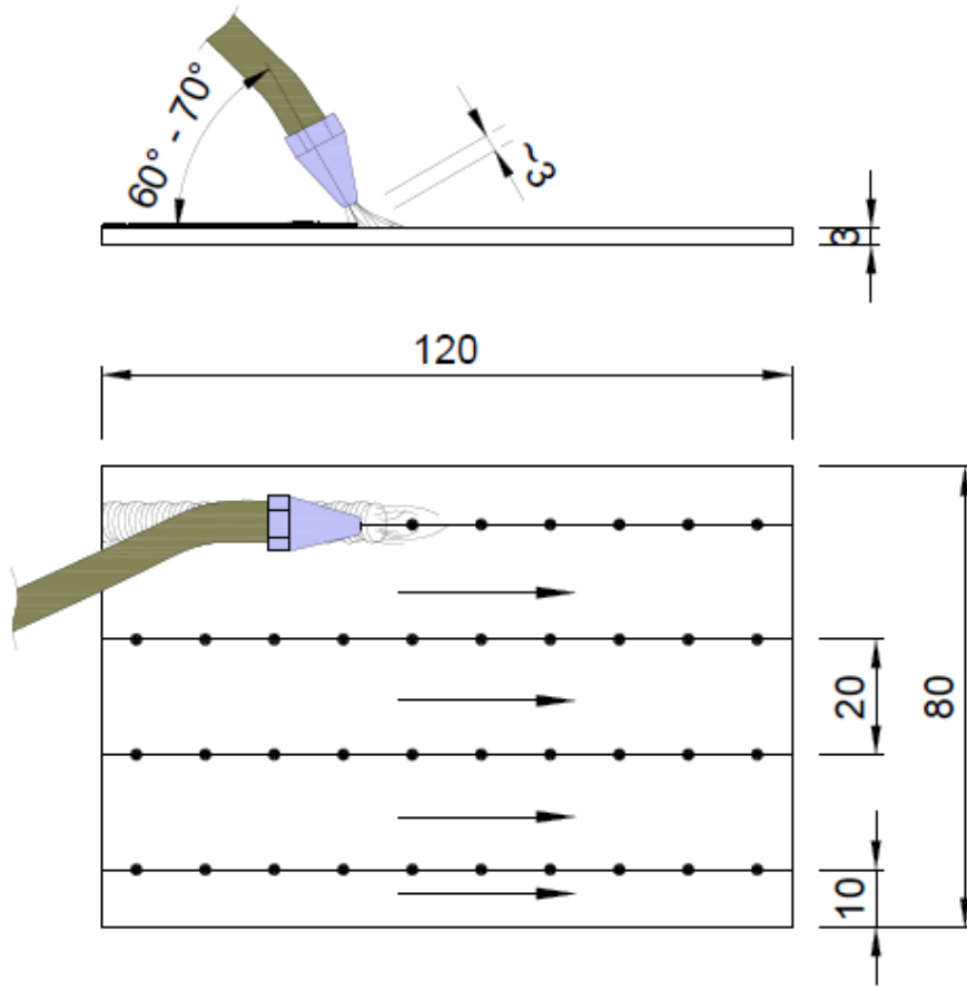
Görsel 9.4: Kaynak uygulaması
