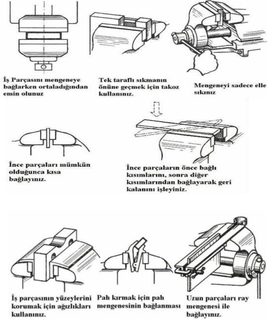
Görsel 3.3: İş parçalarının mengeneye bağlanması
