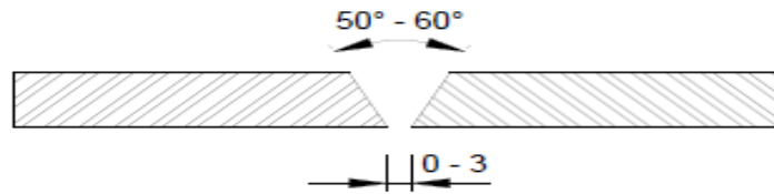
V kaynak ağzı
