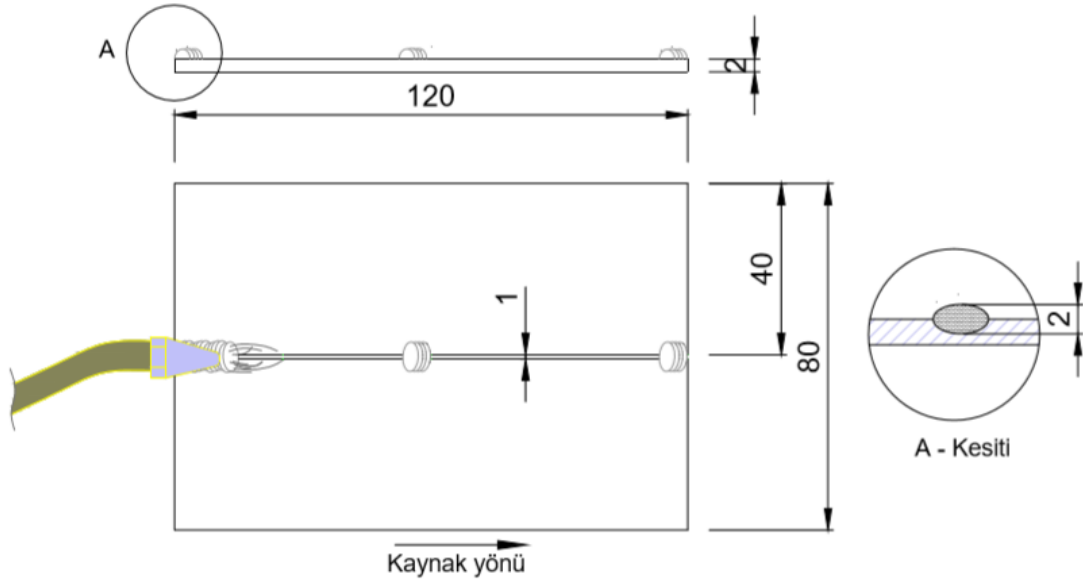
Görsel 9.7: Kaynak uygulaması
