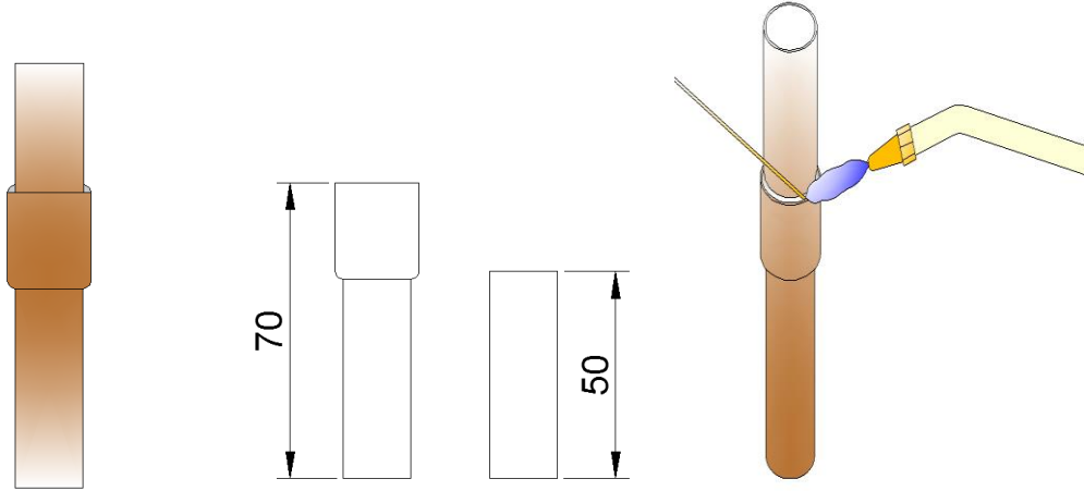
Görsel 7.9: Bakır borulara sert lehimleme
