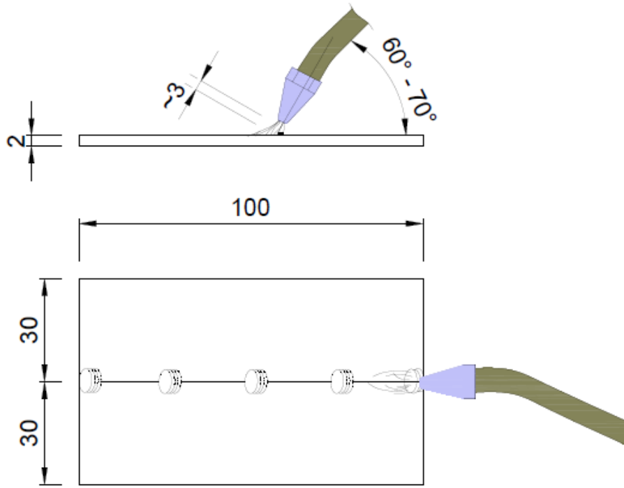
Görsel 9.2: Kaynak uygulaması
