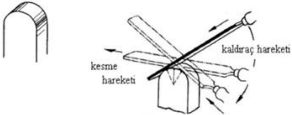
Görsel 3.16: Dışa kavisli yüzeylerin eğelenmesi
