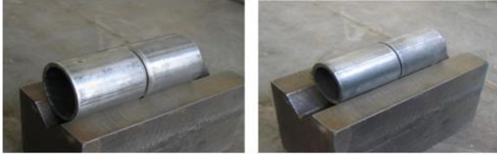
Görsel 12.26: Boruların puntalanmasında kullanılan -V- yatakları
