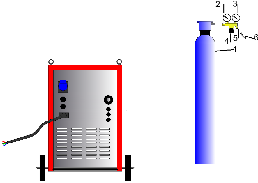
Görsel 12.12:Regülatör bağlantısı
