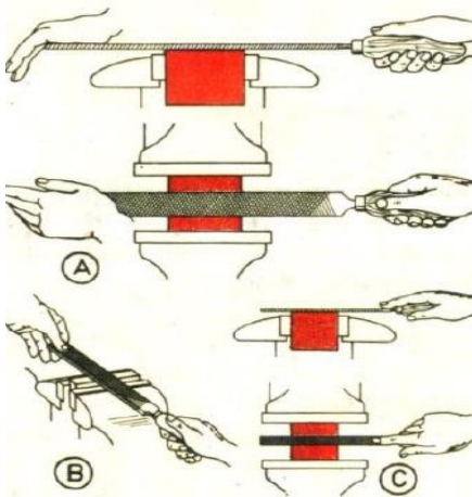
Görsel 3.10:Eğeleme yöntemi
