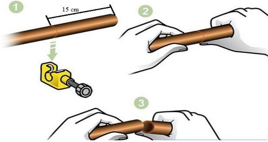
Görsel6.7: Bakır boru kesme işlemi
