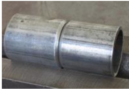
Görsel 13.14: Kaynak ağızı açılmış çelik boru
