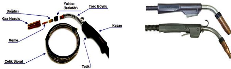
Görsel 12.10: Kaynak torcu
