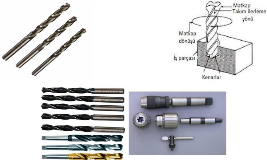
Görsel 3.19: Metal matkap uçları
