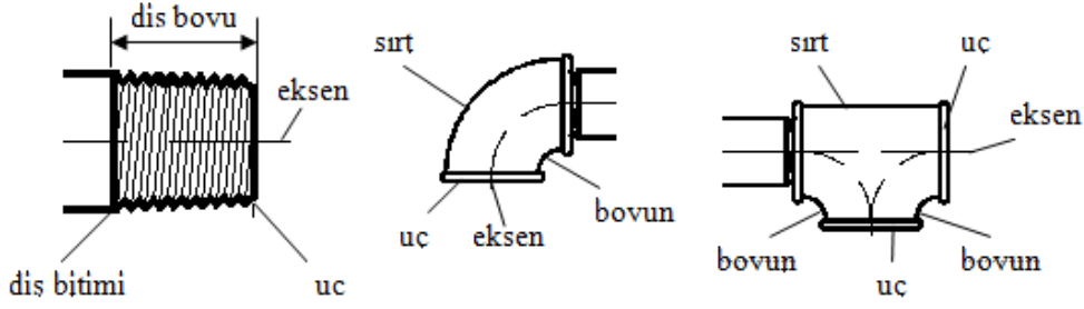
Görsel 4.26: Boru üzerinde ölçü alma terimleri
