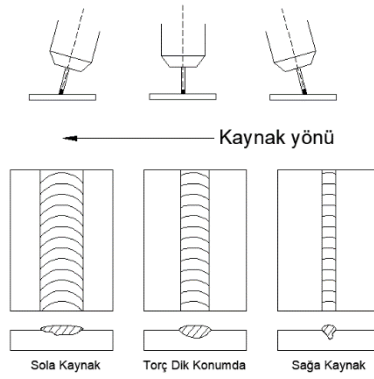
Görsel 12.29: Kaynak konumlarının parça üzerine etkileri
