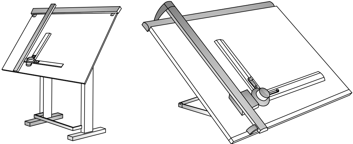
Şekil 1.24 : Resim masaları
