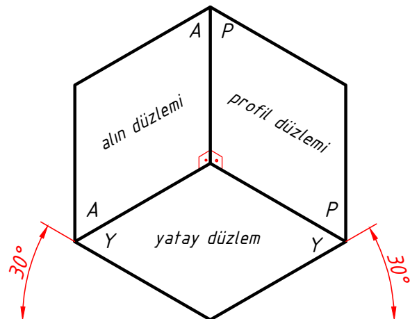
Şekil 2.5: Diedr Düzlemi
