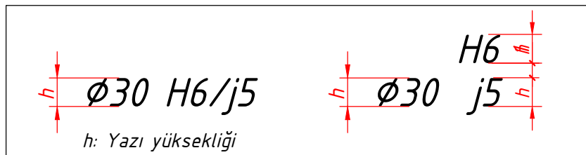
Şekil 3.80: Sembol yükseklikleri
