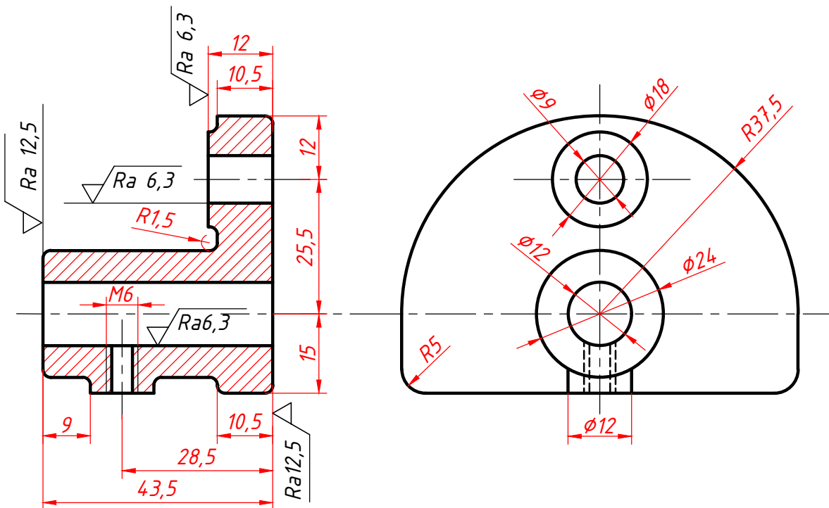
Şekil 3.68: Örnek uygulama çalışması
