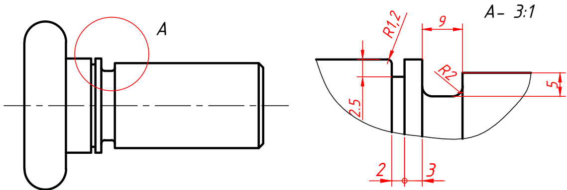
Şekil 2.50: Detay görünüş örneği
