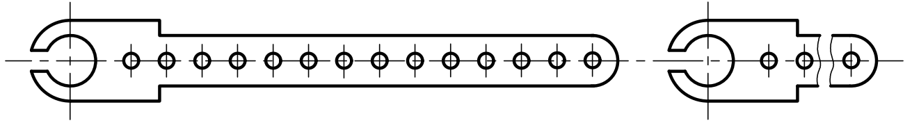
Şekil 2.49: Koparılmış görünüş örneği
