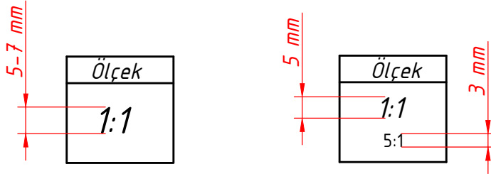
Şekil 3.48: Ölçeklerin antede yazılması
