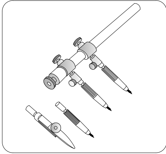
Şekil 1.19 : Baston Pergeli
