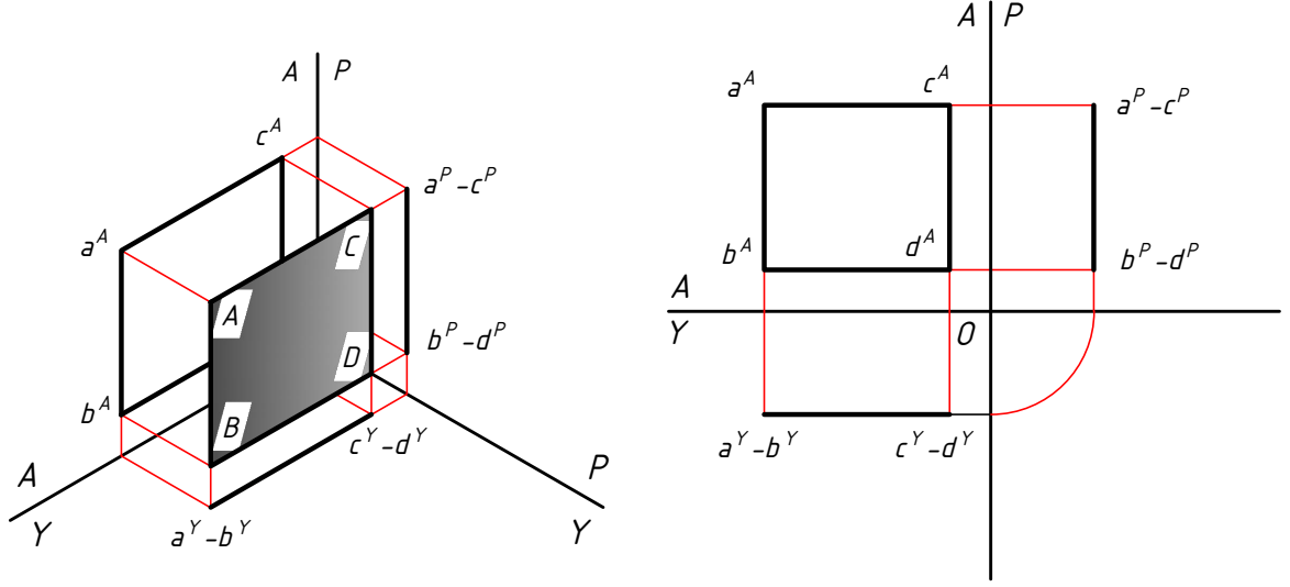
Şekil 2.19: Alın düzlemi
