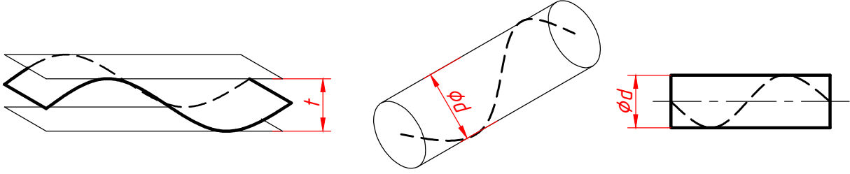
Şekil 3.104: Doğrusallık
