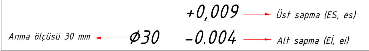
Şekil 3.74: Sapmaların yazılması
