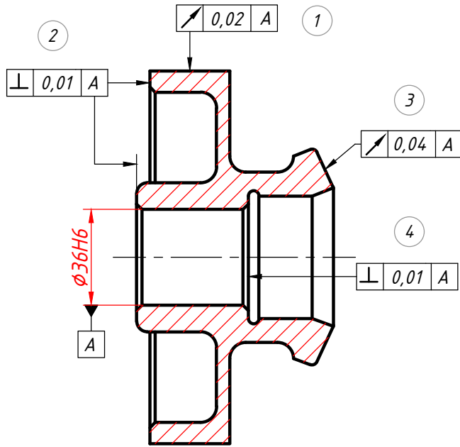
Sürtünme çarkı
