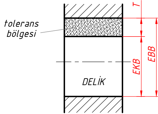
Şekil 3.70: Tolerans bölgesi
