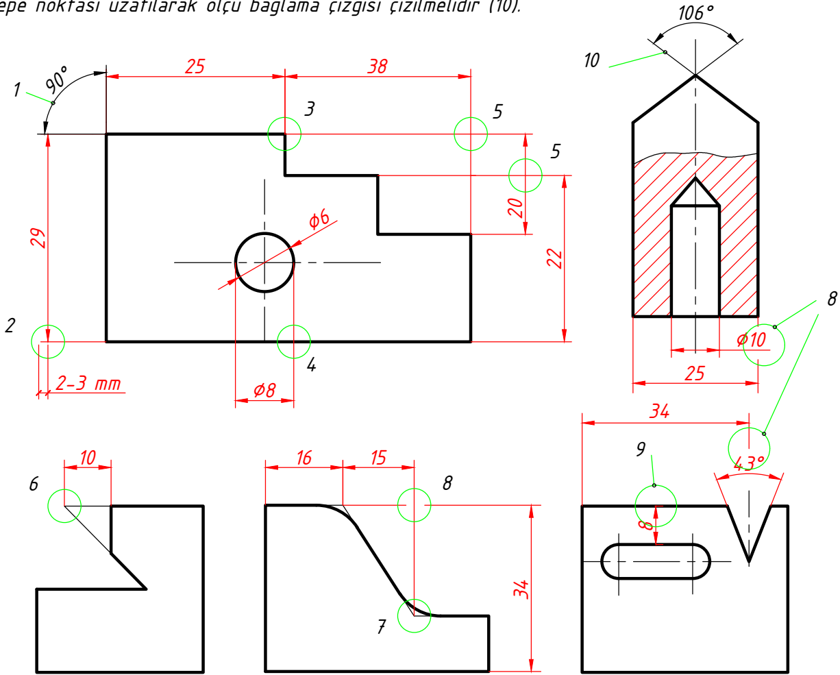
Şekil 3.4: Ölçü bağlama çizgisinin kullanım örnekleri
