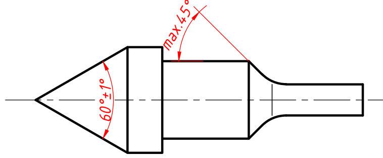
Şekil 3.81: Açıların yazılması
