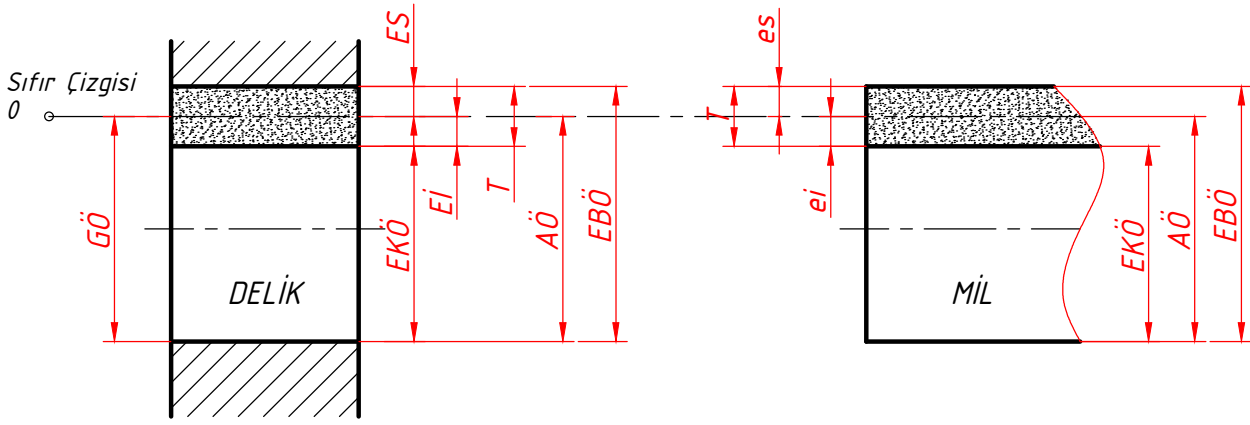
Şekil 3.68: Sıfır Çizgisi
