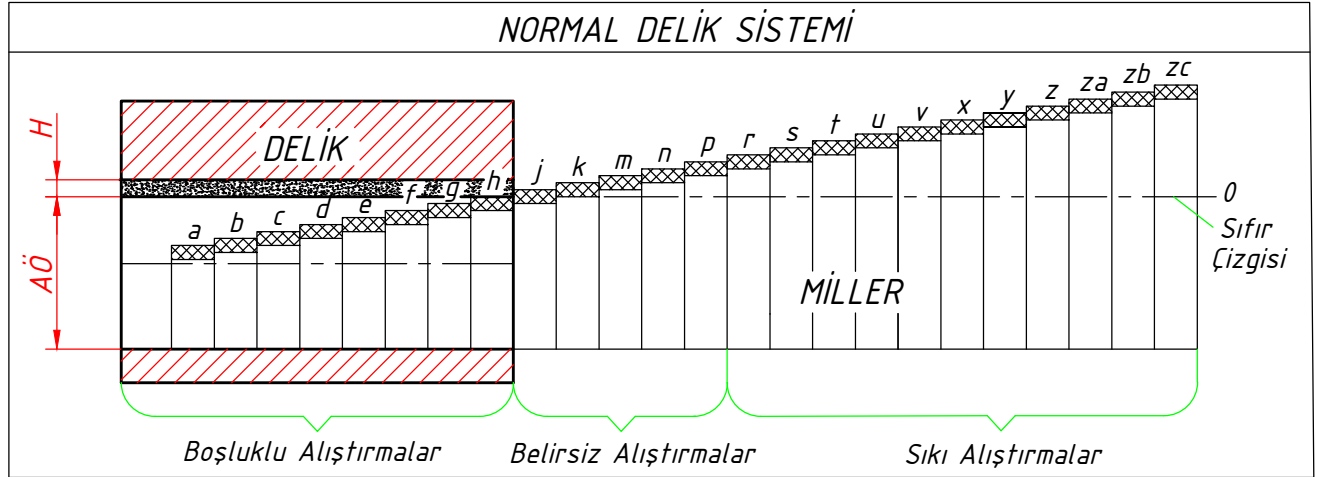
řekil 3.72: Normal delik sisteminde millerin durumu
