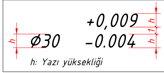
Şekil 3.75: Yazı yüksekliği
