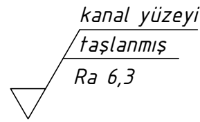
Şekil 3.54: İşleme metodunun gösterilmesi
