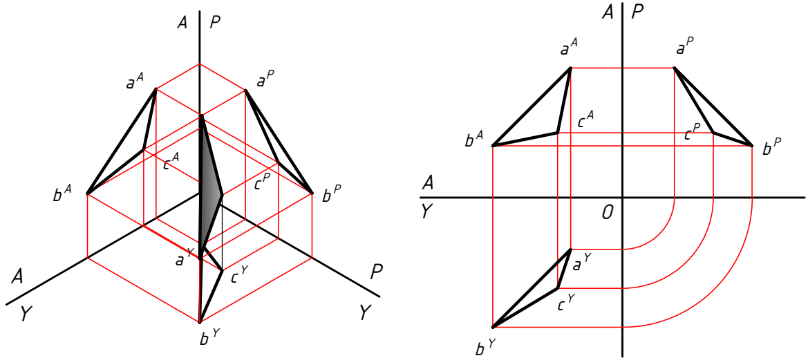
Şekil 2.20: Gelişigüzel düzlem
