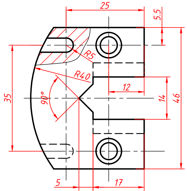
b. Farklı çizgi tipi ve kalınlığı ile çizilmiş resim
