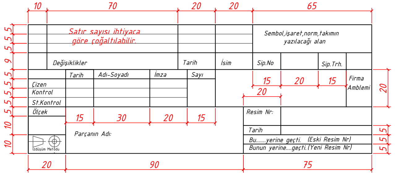
Şekil 1.34 : İmalat sanayinde kullanılan resim anteti örneği ve ölçüleri
