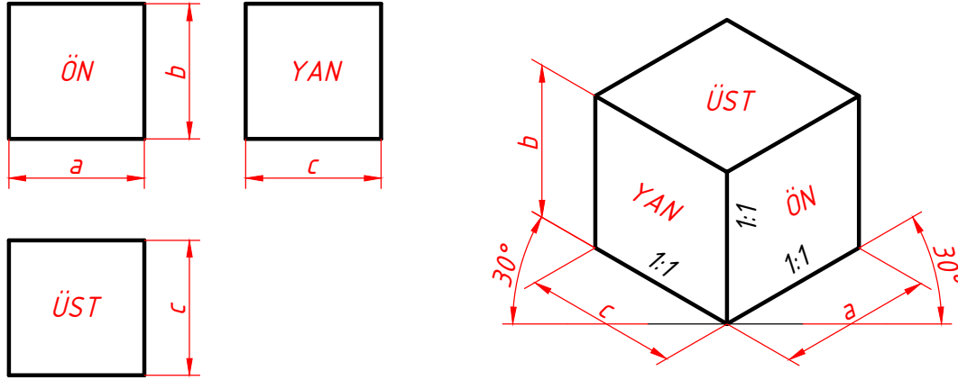
Şekil 4.10: İzometrik perspektif
