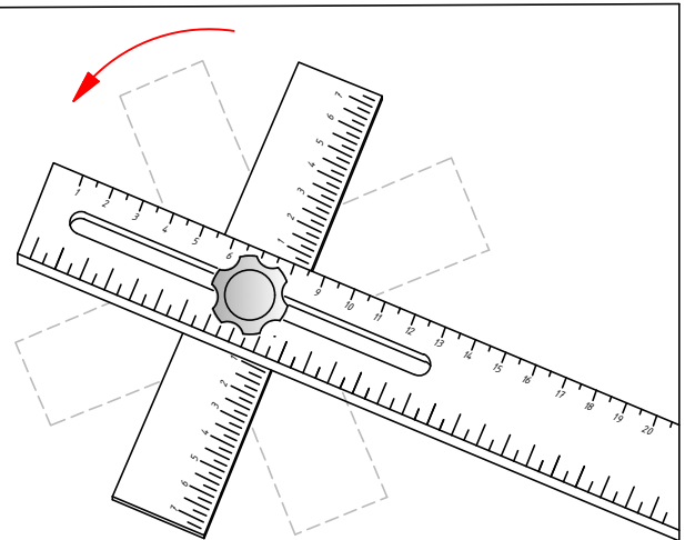
Şekil 1.10 : c. Ayarlanabilir başlı T cetvelleri
