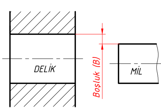
Şekil 3.69: Boşluk
