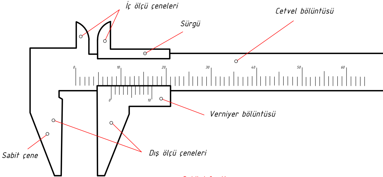
Şekil 4.2 : Kumpas
