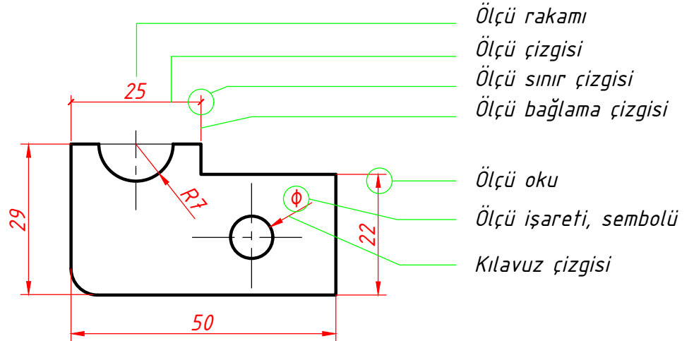
Şekil 3.1: Ölçülendirme elemanları
