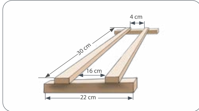
Görsel 1.29: Ksilofonun ahşap iskeleti
