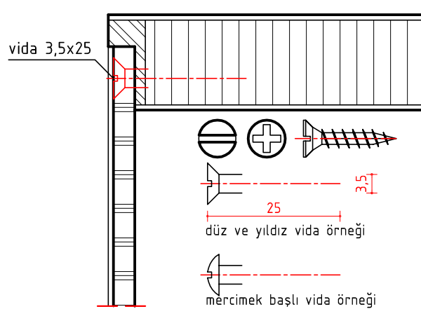
Şekil 3.31: Vidaların gösterilmesi
