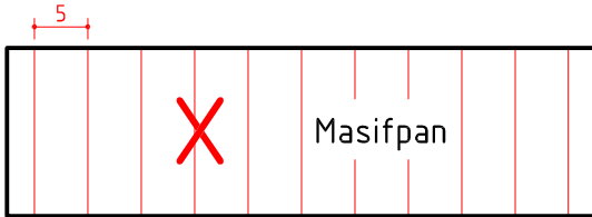
Şekil 3.19a: Masifpan tarama ve makta sembolü
