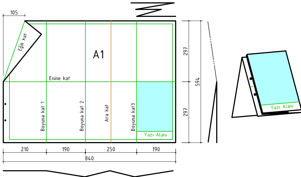
Şekil 1.2c: A1 kâğıdı ve katlaması
