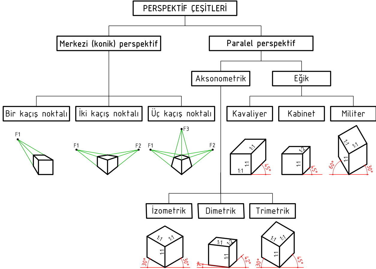
Şekil 3.2: Perspektif çeşitleri
