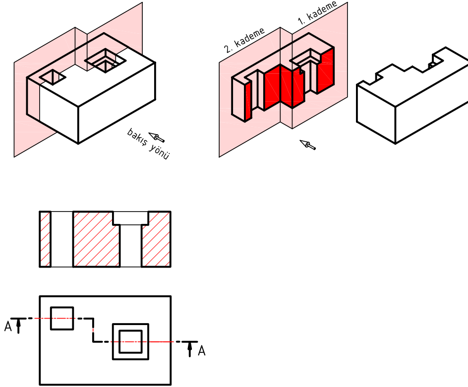
Şekil 2.33: Kademeli kesit
