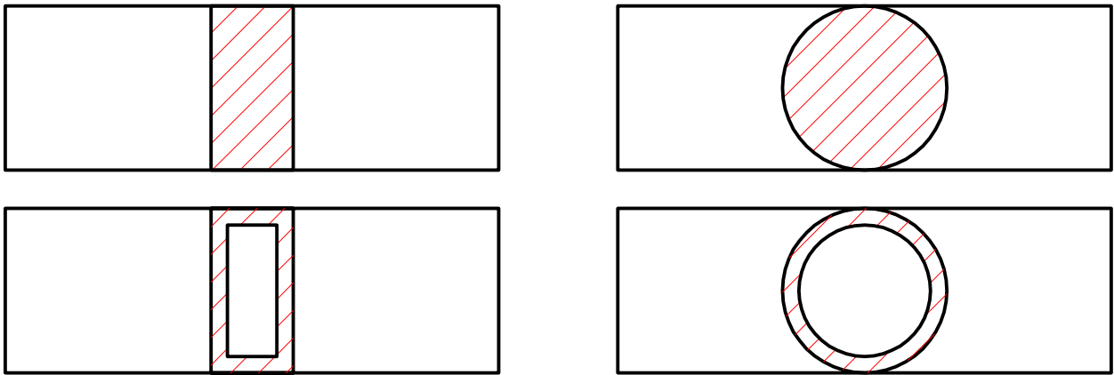
ön görünüş üzerinde profil kesit gösterilişi
