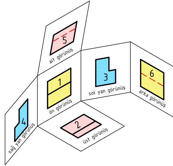
Şekil 2.17b: Küpün açılması
