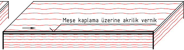
Şekil 3.12b: Yüzey yön (paralel) ve yüzey durumu işareti
