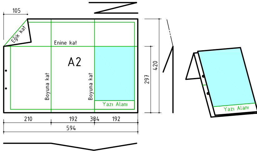
Şekil 1.2b: A2 kâğıdı ve katlaması
