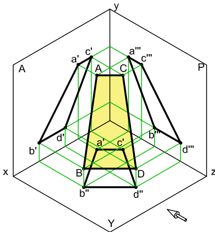
Şekil 2.13: Üç düzleme de eğik olan (aykırı) düzlemin iz düşümleri ve epürdeki konumu
