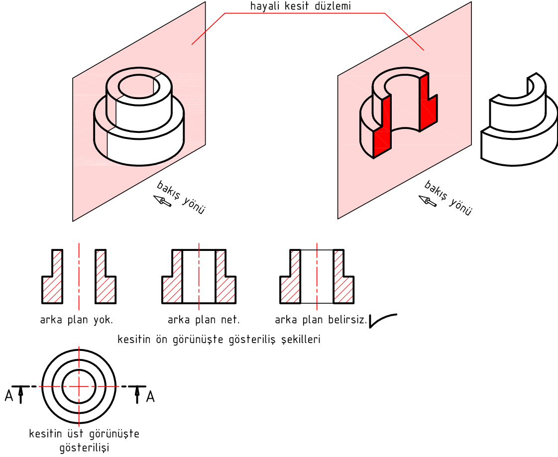
Şekil 2.31: Tam kesit
