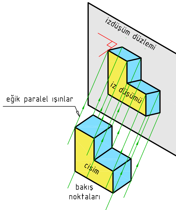
Şekil 2.2a: Dik izdüşüm
