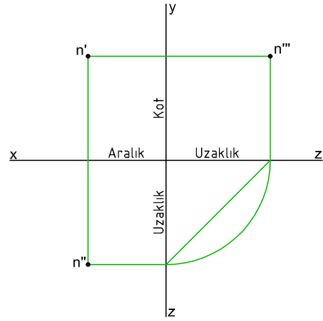
Şekil 2.6b: Epür koordinatları
