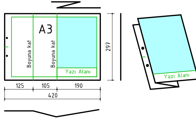
Şekil 1.2a: A3 kâğıdı ve katlaması
