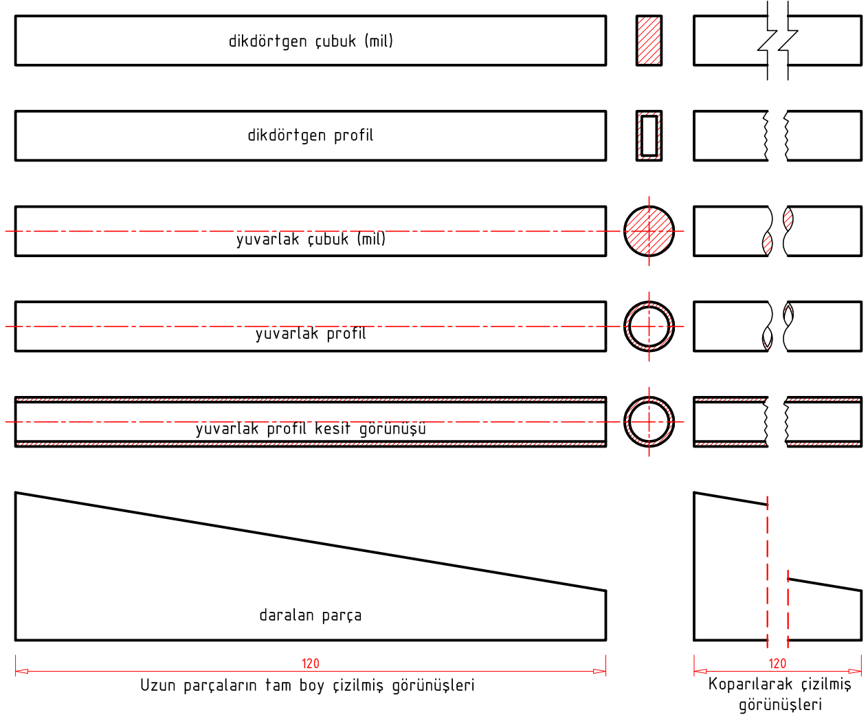
Şekil 2.29: Koparılmış görünüşler
