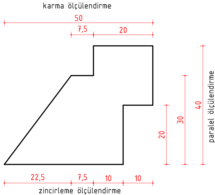
Şekil 3.17: Ölçülendirme yöntemleri
