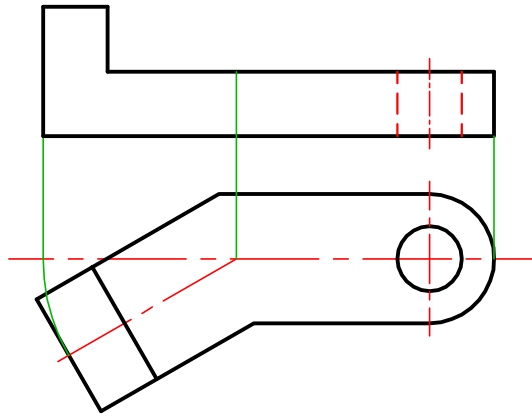
Şekil 2.27: Döndürme metodu ile yardımcı görünüş
