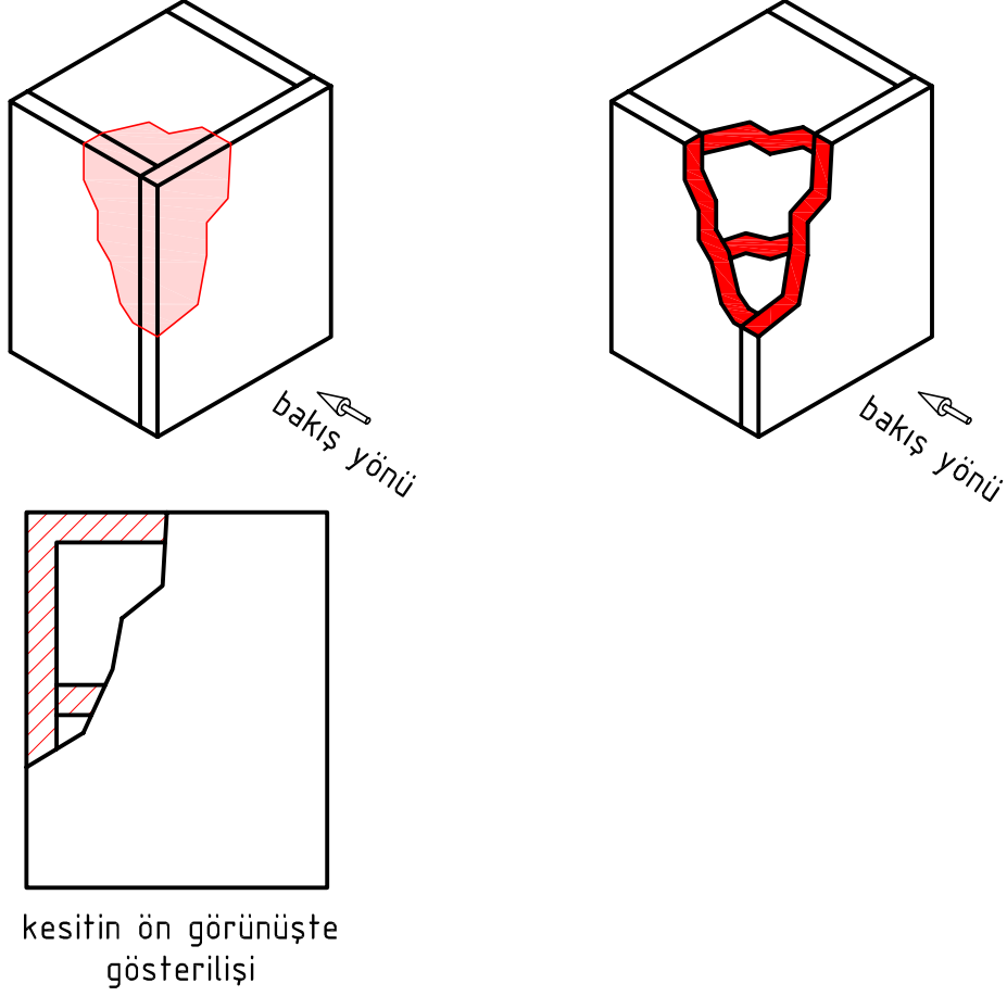
Şekil 2.35: Kısmi kesit
