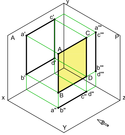
Şekil 2.11: Alın düzlemine paralel düzlemin iz düşümleri ve epürdeki konumu
