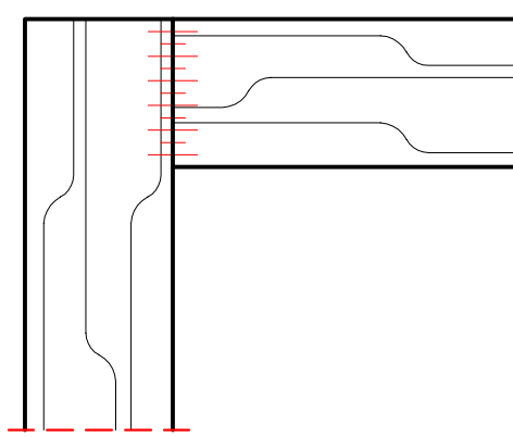
Şekil 3.29: Tutkallama işareti
