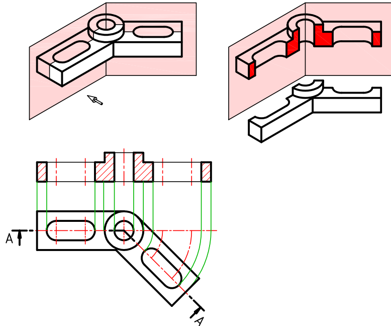
Şekil 2.34: Döndürülmüş kesit
