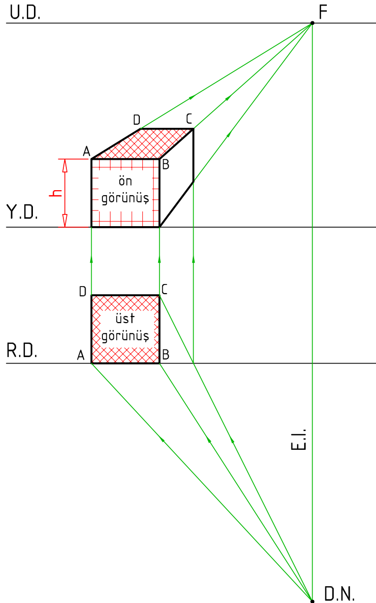
Şekil 3.6: Merkezi perspektif
