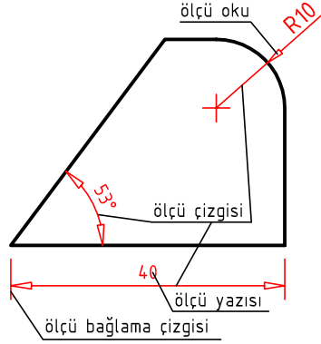
Şekil 3.9a: Ölçülendirme elemanları
