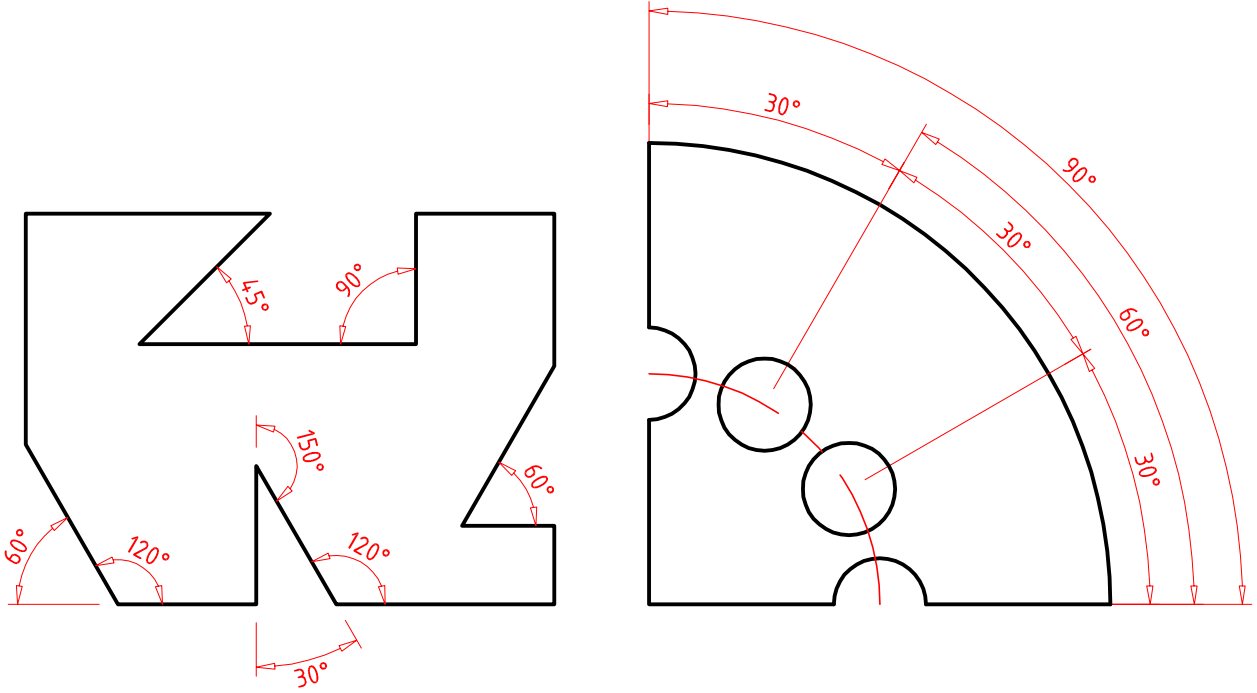
Şekil 3.14: Açı ölçülendirmeleri
