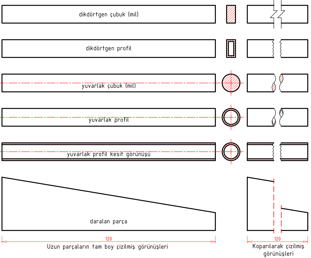
Şekil 2.29: Koparılmış görünüşler
