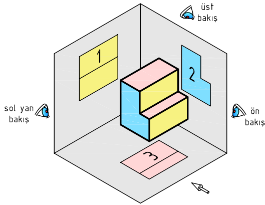
Şekil 2.3: Esas izdüşüm bölgeleri
