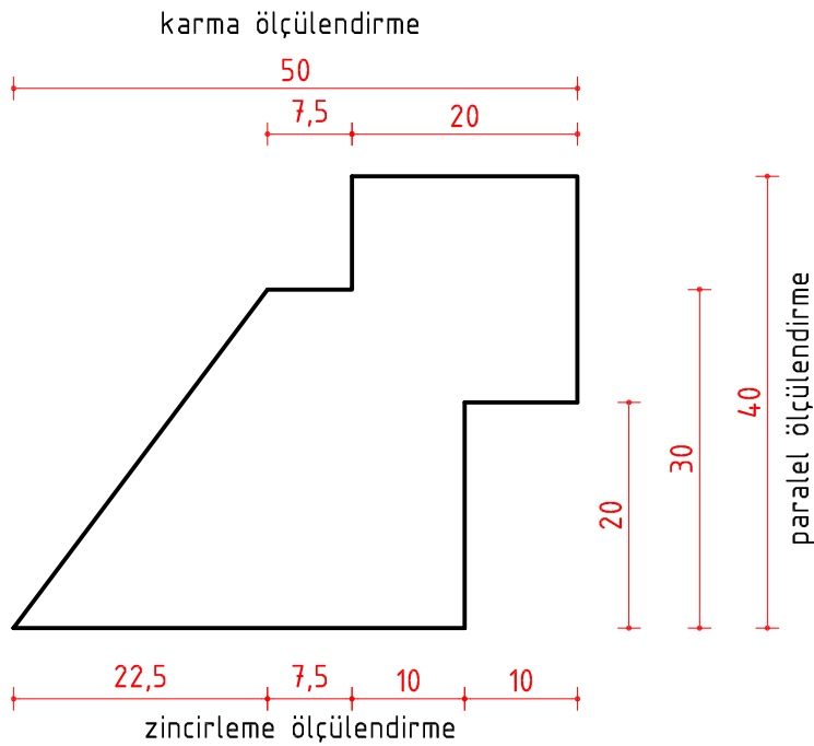
Şekil 3.17: Ölçülendirme yöntemleri
