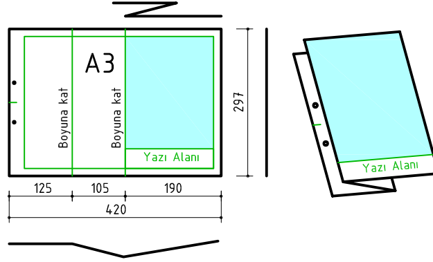
Şekil 1.2a: A3 kâğıdı ve katlaması
