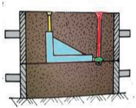
Resim 2.38: Kalıpta yolluk sistemi
