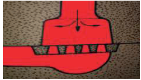
Resim 2.44 Cürufluğa yerleştirilmiş süzgeç
