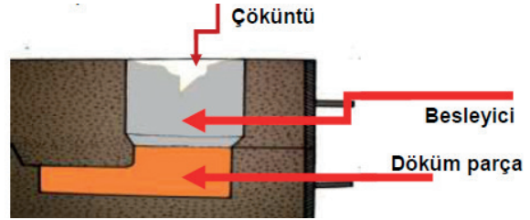
Resim 2.46: Kalıplama sırasında modelin kalın ve üst kısmına yerleştirilen açık besleyici ve çöküntü
