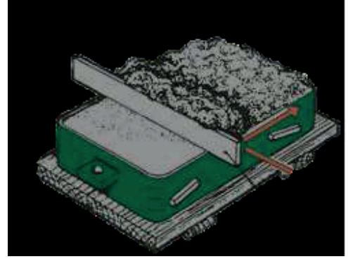
Resim 2.1: Fazla kumun mastar ile sıyırılması
