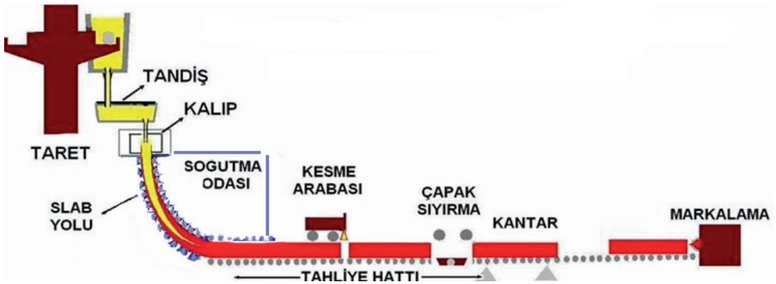
Resim 2.37: Sürekli döküm sistemi
