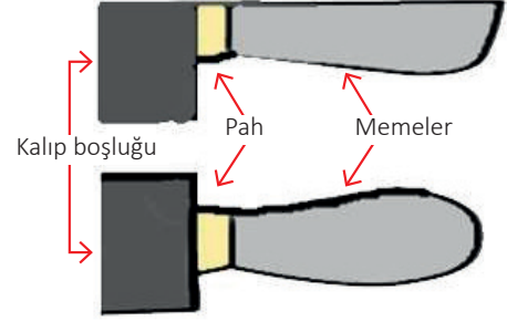
Resim 2.40: Meme ağzına pah kırma işlemi
