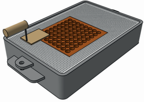
Resim 2.57: Çivinin mala ile bastırılması
