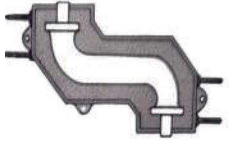
Resim 2.3: Modele uygun özel derece
