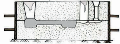
Resim 2.49: Kalıplamada besleyicilerin konumu
