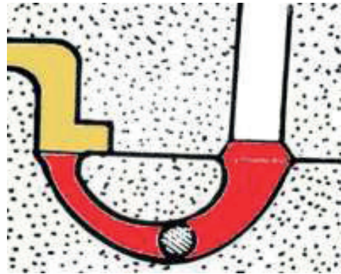
Resim 2.42: Boynuz yolluk
