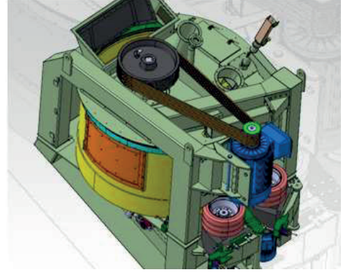
Resim 1.3: Kum hazırlama mikseri
