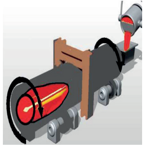
Resim 2.36: Savurma döküm sistemi
