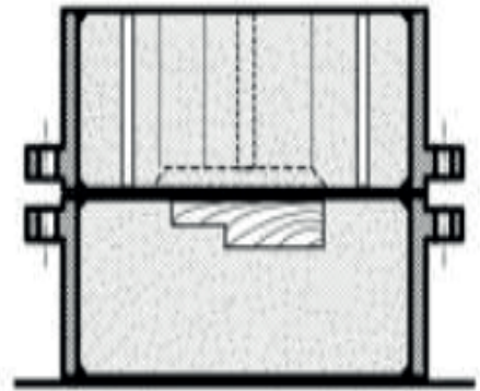
Resim 2.30: Master çekilmiş üst dereceye şiş çekilmesi
