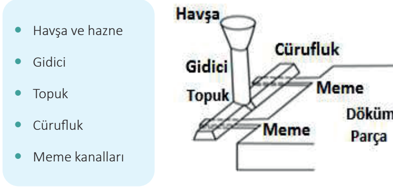
Resim 2.39: Yolluk sistemi
