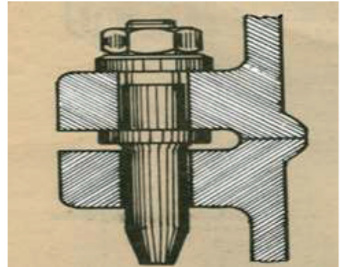
Resim 2.4: Pim, pim delikleri, el sapları
