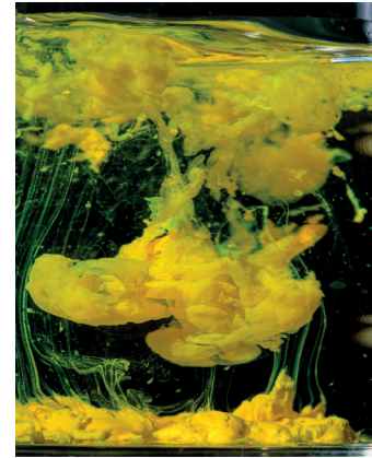
Görsel 2.1.19: Kurşun (II) kromatın çökmesi
