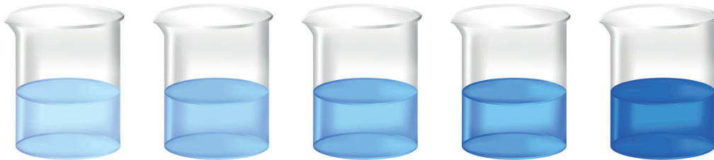
Görsel 3.1.3: Seyreltik çözelti ile derişik çözeltinin karşılaştırılması
