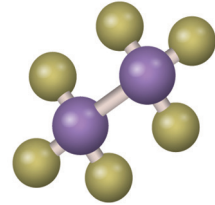
Görsel 2.1.7: \text{C}_2\text{H}_6 molekülü
