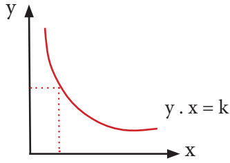
Grafik: 1.1.2: Ters orantı grafiğı
