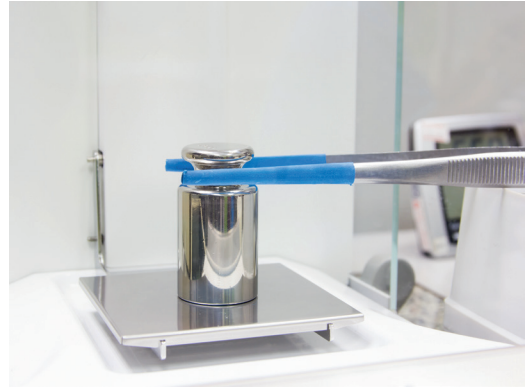
Görsel 1.1.3: Analitik terazinin kalibrasyon doğrulaması.
