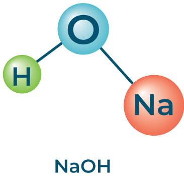
Şekil 2.3: Sodyum hidroksit
