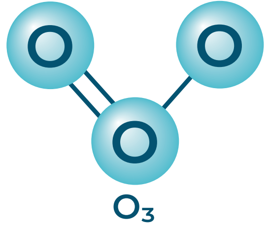
Şekil 4.2: Ozon molekülü
