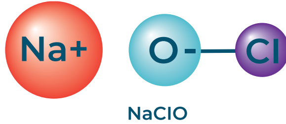
Şekil 2.7: Sodyum hipoklorit
