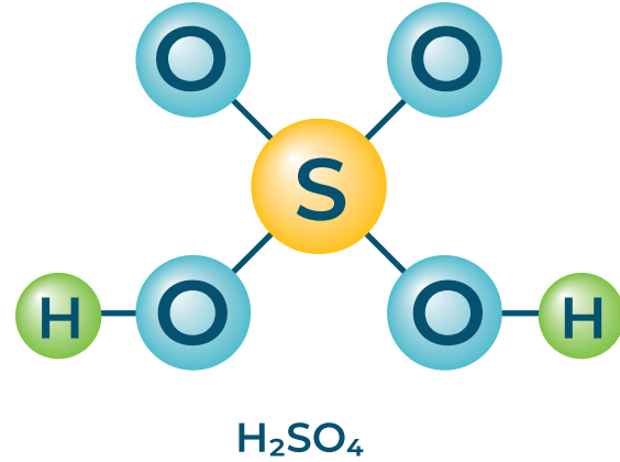
Şekil 2.6: Sülfirik asit
