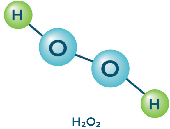
Şekil 2.9: Hidrojen peroksit
