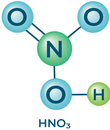
Şekil 2.5: Nitrik asit
