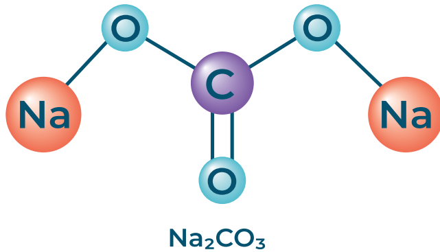
Şekil 2.4: Sodyum karbonat
