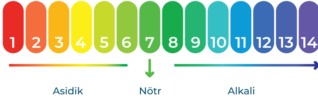
Şekil 2.2: pH ölçeği
