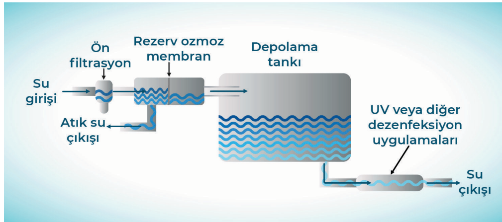
Görsel 4.5: Ters ozmoz sistemi
