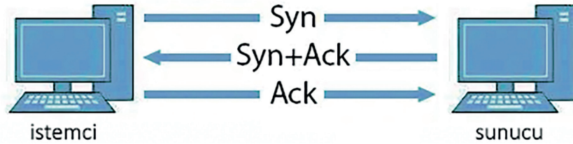
Görsel 7.24: Üçlü el sıkışma
