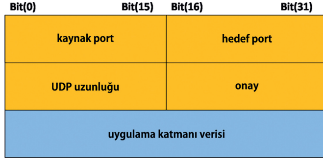
Görsel 7.26: UDP başlığı
