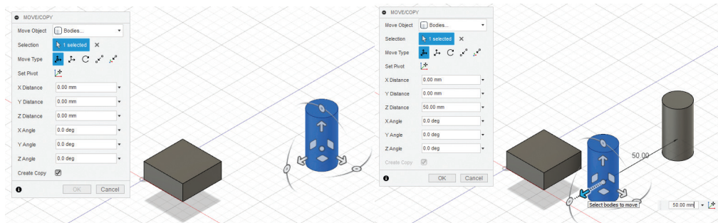
Görsel 3.73: Move / Copy komutuyla Point to Point kopyalama işlemi
