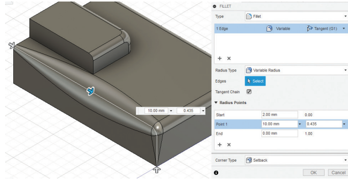
Görsel 3.105: Değişken yarıçaplı yuvarlatma
