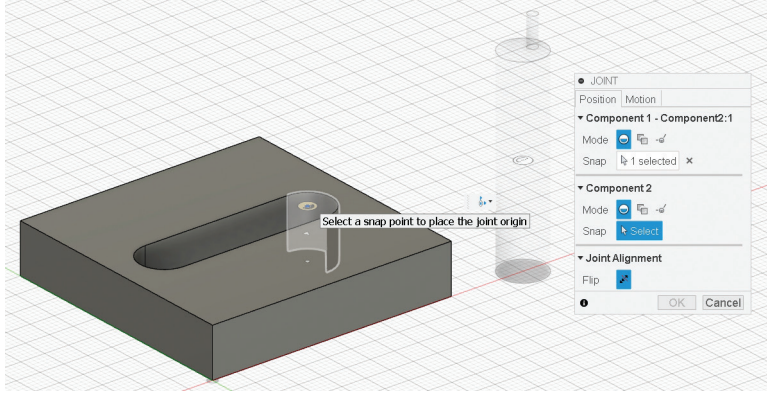
Görsel 3.129: Yatak parçası montaj noktası belirleme
