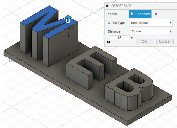
Görsel 3.114: Seçilen yüzeyi öteleme
