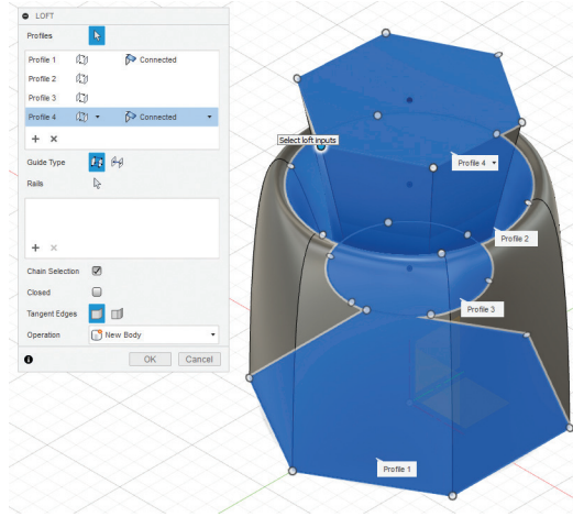
Görsel 3.62: Loft komutu ile nesne oluşturma seçim sırası değişirse farklı bir nesne oluşumu
