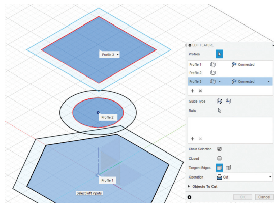
Görsel 3.88: Loft komutu ile nesnenin çıkarılması
