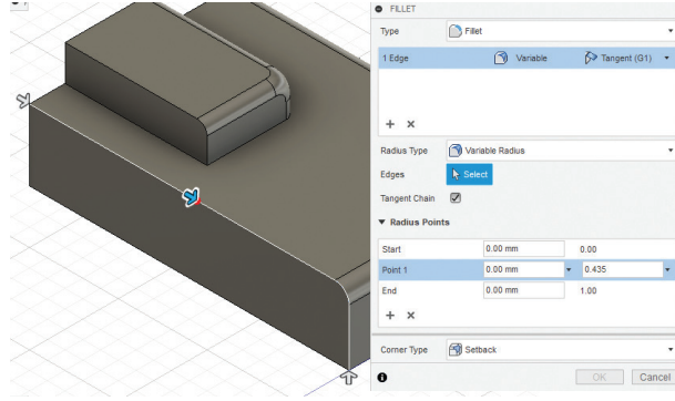
Görsel 3.104: İkinci yuvarlatma noktası belirleme
