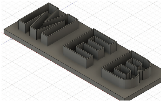
Görsel 3.109: Et kalınlığı verilecek yüzey seçimi
