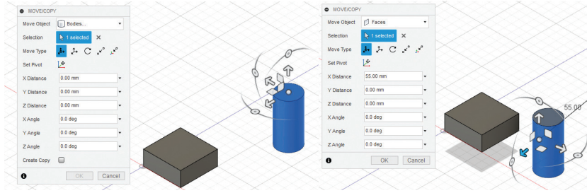
Görsel 3.71: Move / Copy komutuyla taşıma işlemi
