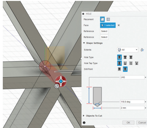
Görsel 3.70: Hole komutu ile delik açma
