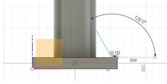
Görsel 3.64: Payanda için yardımcı doğru parçası çizimi
