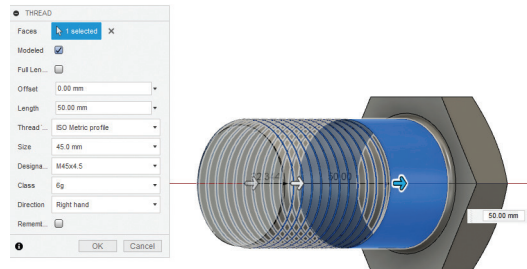
Görsel 3.93: Belirlenen uzunlukta diş açılması
