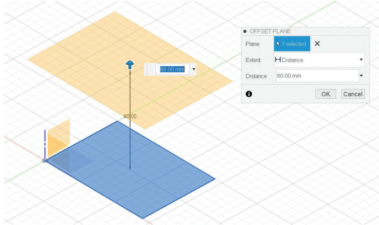
Görsel 3.38: Düzlem ötele
