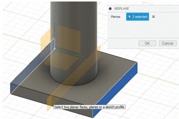
Görsel 3.63: Midplane (orta düzlem) oluşturma
