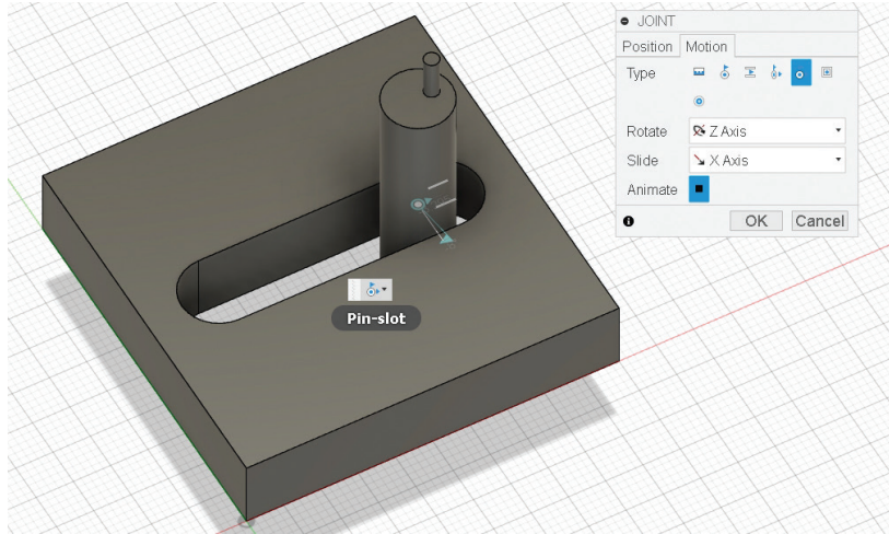
Görsel 3.130: Pin- Slot Joint işlem sonucu
