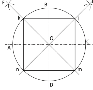
Grsel 1.29: Eřkenar drtgeni oluřturma
