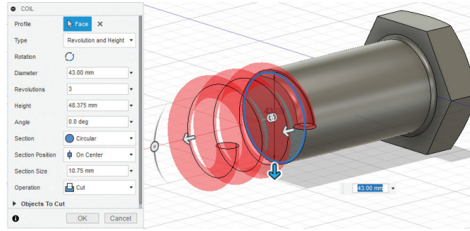
Görsel 3.94: Coil komutuyla yay oluşturma
