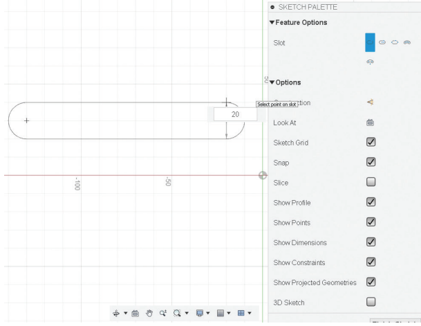
Görsel 3.25: İki eksen arası ölçüyle yarıçap ölçüsünü işaretleyerek kanal çizme
