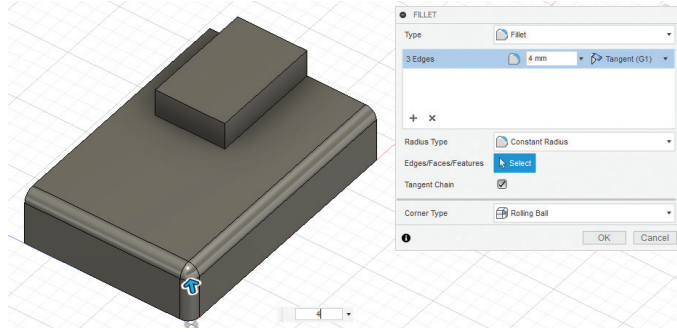
Görsel 3.101: Fillet komutu ile sabit yarıçaplı yuvarlatma
