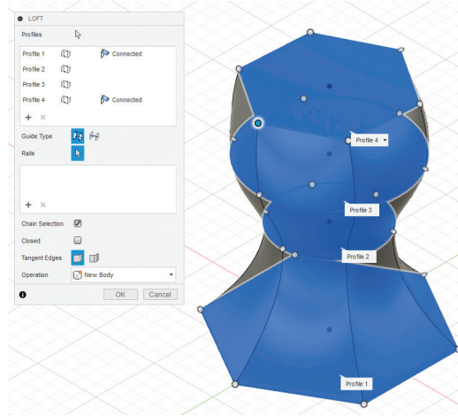
Görsel 3.61: Loft komutu ile nesne oluşturma
