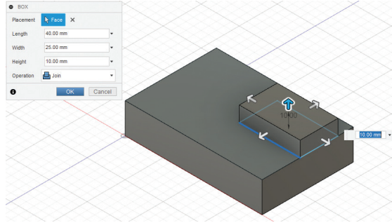
Görsel 3.96: Box komutu ile ikinci nesnenin oluşturulması
