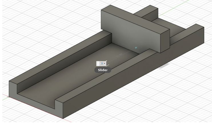
Görsel 3.124: Slider Joint işlem sonucu
