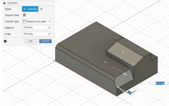
Görsel 3.99: Chamfer komutu ile Distance and Angle (Uzaklık ve Açı) pah kırma
