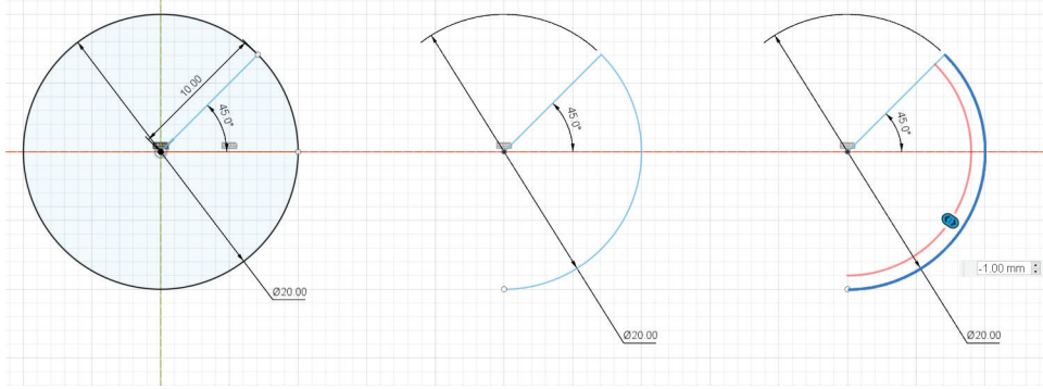
Görsel 3.132: İçi boş küre taslak çizimi
