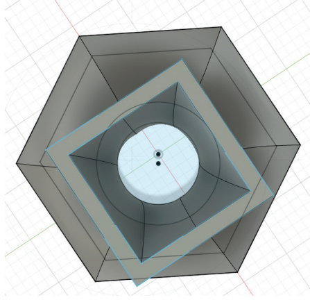
Görsel 3.90: Çıkarma işlemi sonrası nesnenin üstten görünümü
