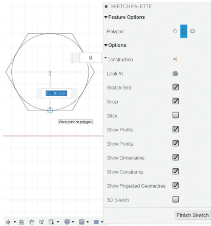
Görsel 3.28: Daire dışına çokgen çizme
