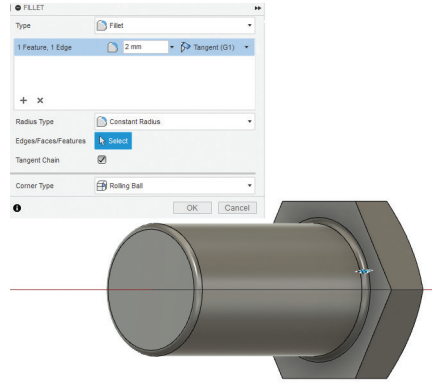
Görsel 3.92: Silindirin başlangıç ve birleşim yüzeylerinin yuvarlanması
