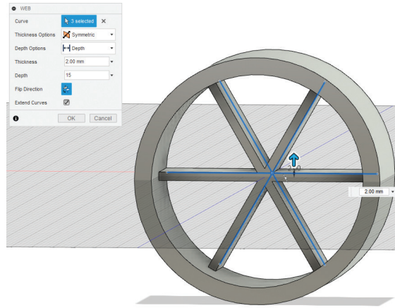
Görsel 3.69: Web komutu ile destek elemanlarını oluşturma
