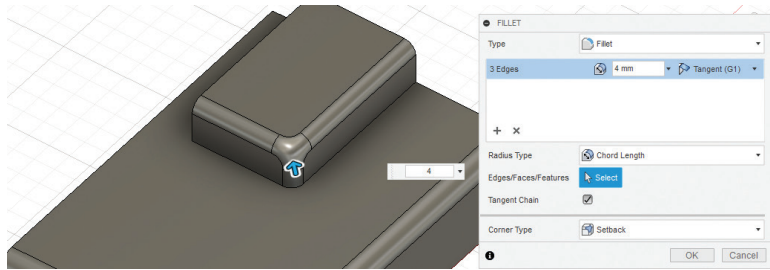
Görsel 3.102: Fillet komutu ile sabit uzunlukla yuvarlatma
