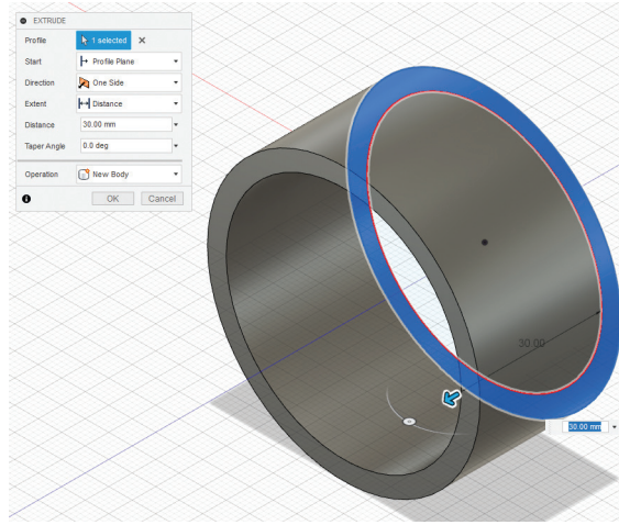
Görsel 3.67: Extrude ile kalınlık verme
