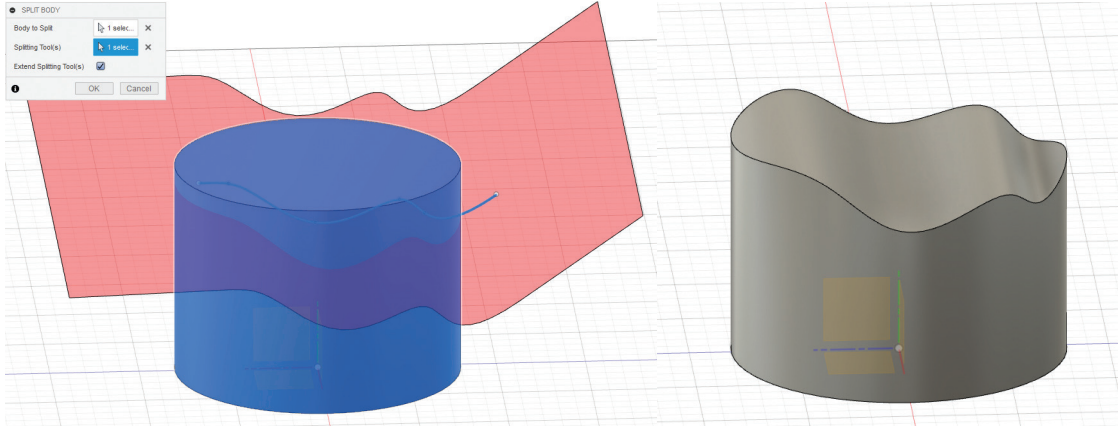
Görsel 3.111: Split komutu ayarları ve nesneyi bölme
