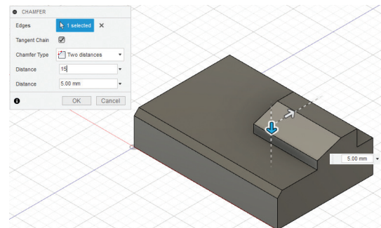
Görsel 3.98: Chamfer komutu ile Two Distance (İkili Uzaklık) pah kırma
