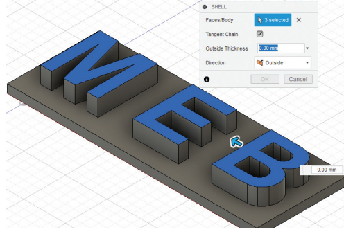
Görsel 3.108: Et kalınlığı verilecek yüzey seçimi
