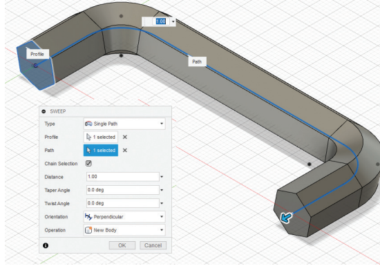
Görsel 3.58: Sweep komutu
