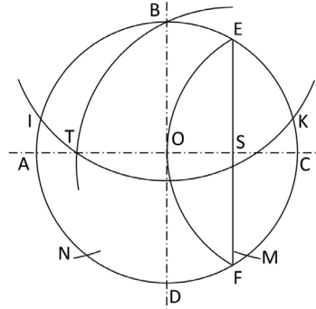
Grsel 1.31: T ve K noktalarını bulma
