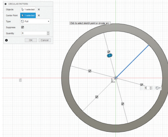
Görsel 3.68: Sketch ortamında doğru parçası çizimi ve çoğaltma
