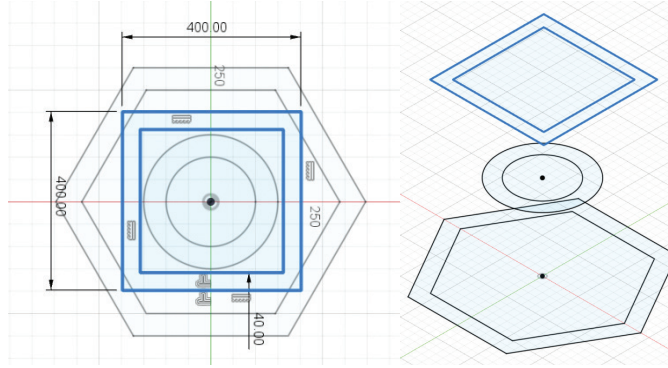
Görsel 3.86: Çizimlerin yukarıdan ve yandan görünüşü
