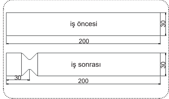
Görsel 13.1: İş parçası lama
