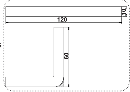
Görsel 12.4: Çelik çubuk
