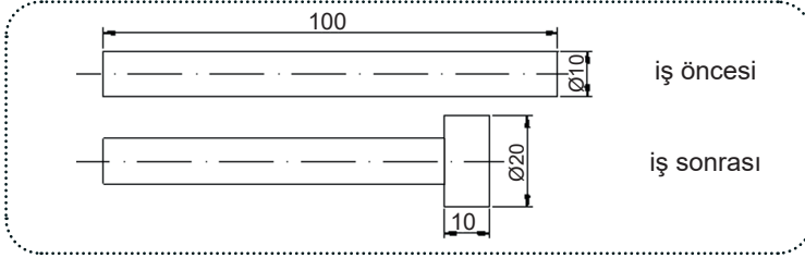
Görsel 12.2: Çelik çubuk
