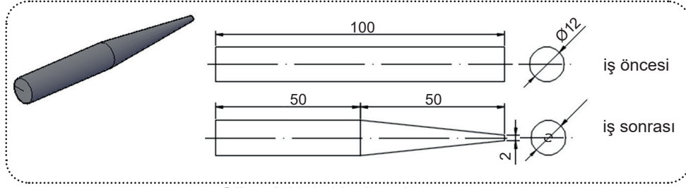
Görsel 11.6: Konik çekme
