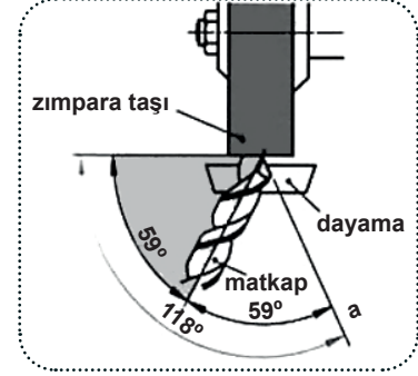
Görsel 8.1.b: Bileme açısı
