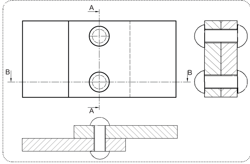
Görsel 10.2: Bindirmeli perçinli birleştirme yapımı
