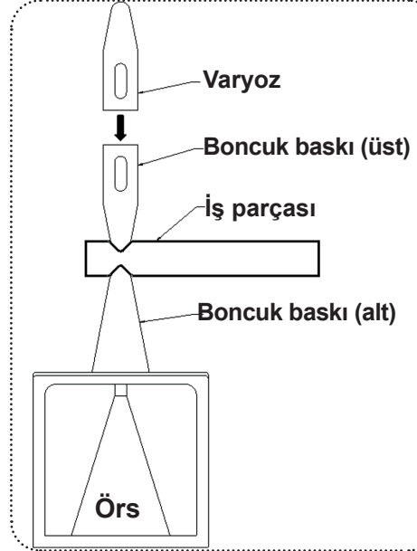
Görsel 13.2: Boğma işlemi
