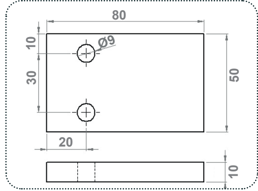
Görsel 8.1.c: Delme kontrolü
