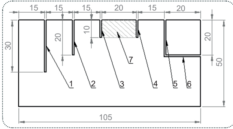
Görsel 5.1.a: İş parçası ölçü
