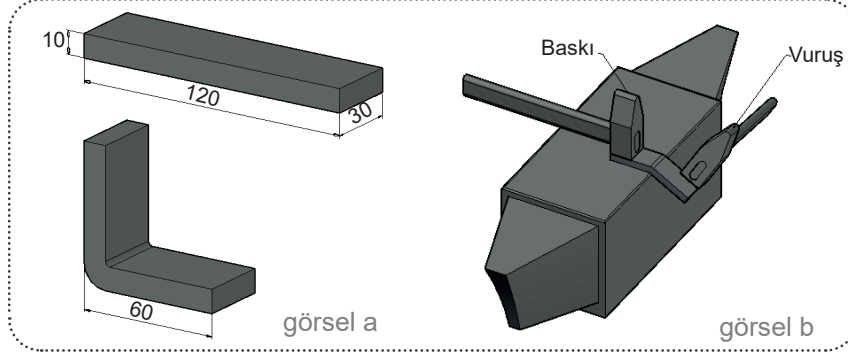
Görsel 12.1: Sıcak bükme
