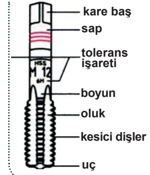
Görsel 9.1.b: Kılavuz
