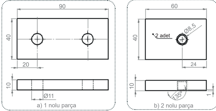
Görsel 8.2: Delme işlemi, havşa açımı
