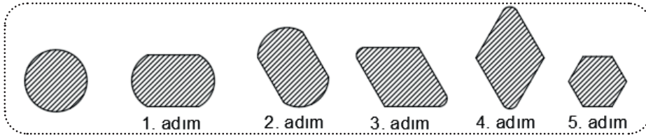
Görsel 11.4: Altıgen çekme
