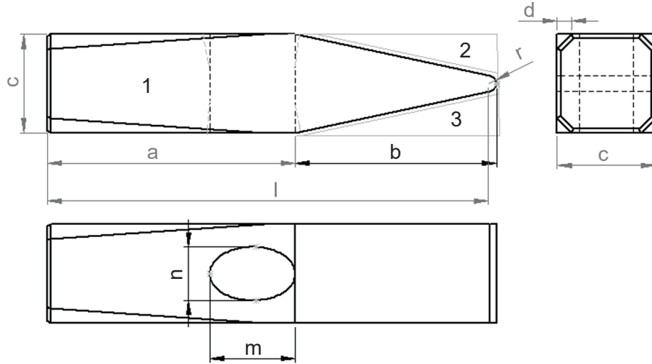
Görsel 6.3: Çekiş yapımı
