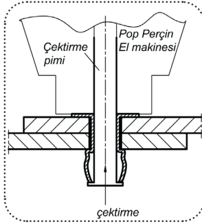
Görsel 10.7: Pop perçin işlemi
