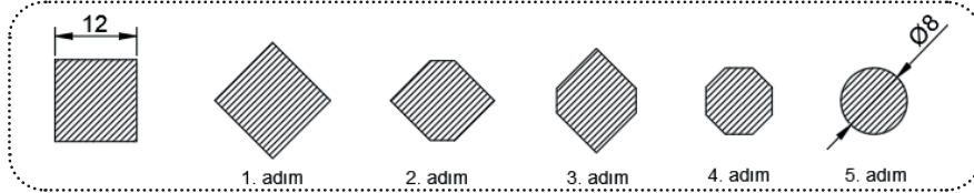
Görsel 11.5: Yuvarlak çekme
