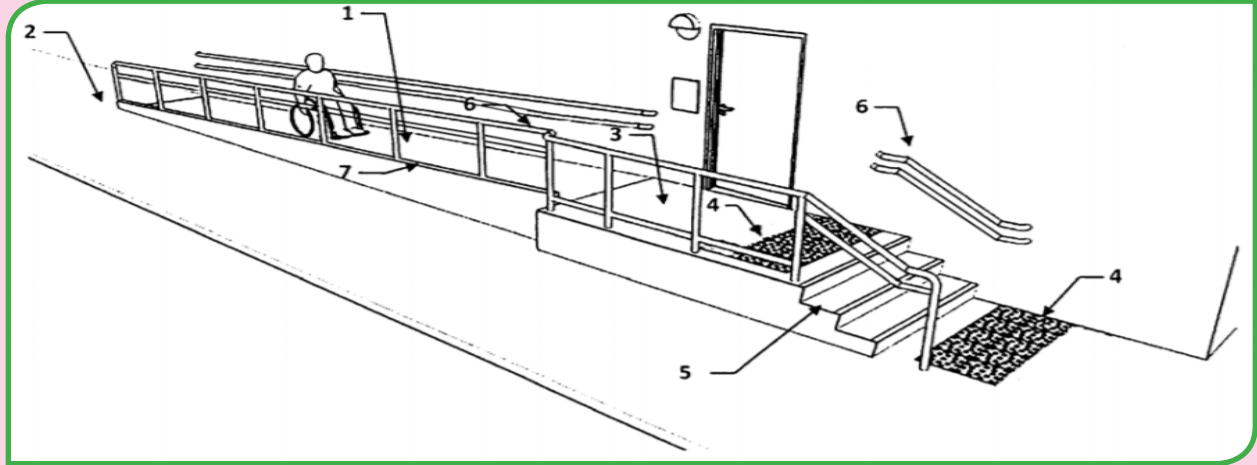
Şekil 1.18: Konut girişi rampa örneği
