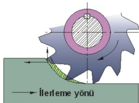
Şekil 1.4.3: Zıt yönlü frezeleme
