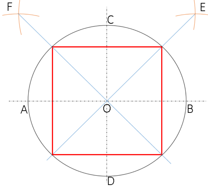
Şekil 1.1.18: Dörtgen çizimi
