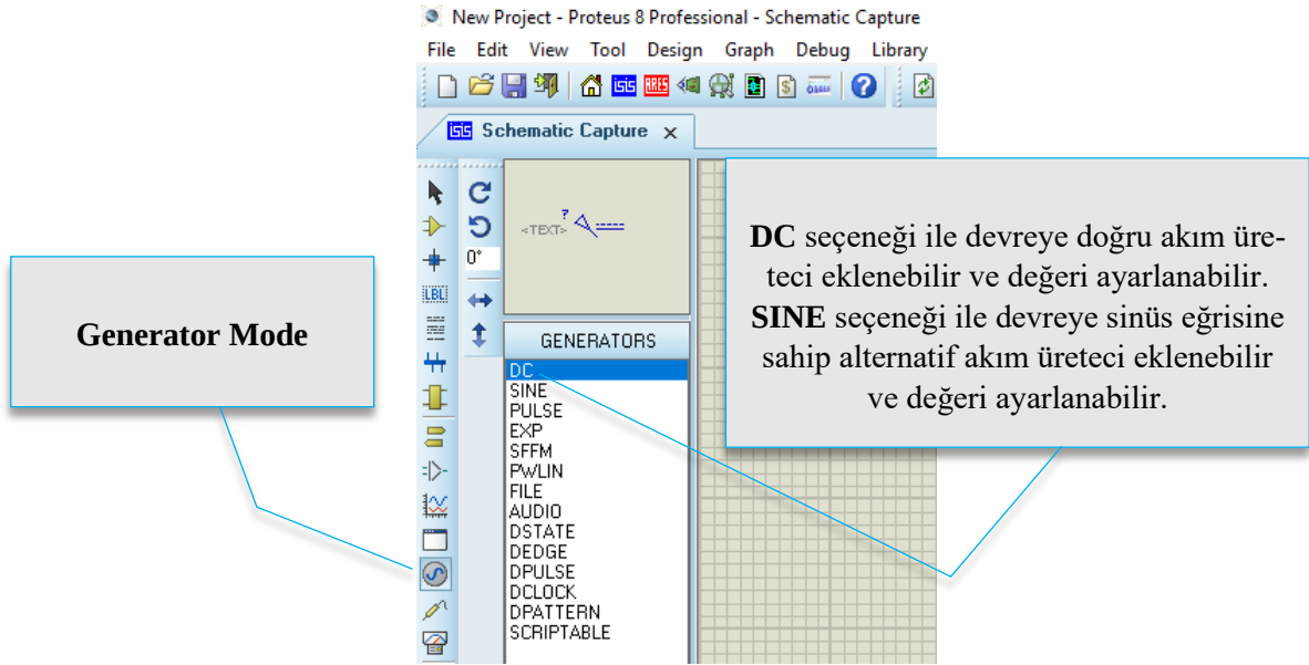
Şekil 2.1.7: Generator Mode
