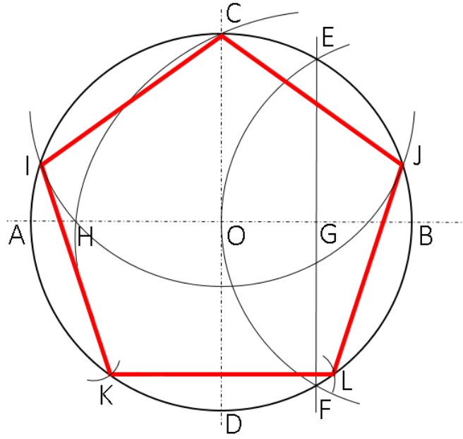
Şekil 1.1.19: Beşgen çizimi
