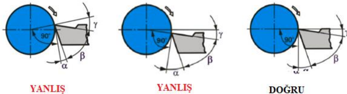
Şekil 1.3.5: Kalem yüksekliği
