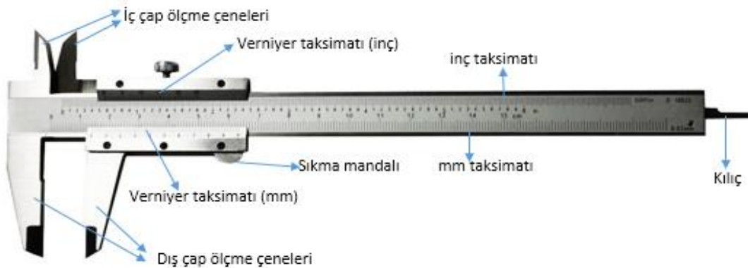
Şekil 1.2.3: Verniyerli kumpas ve kısımları
