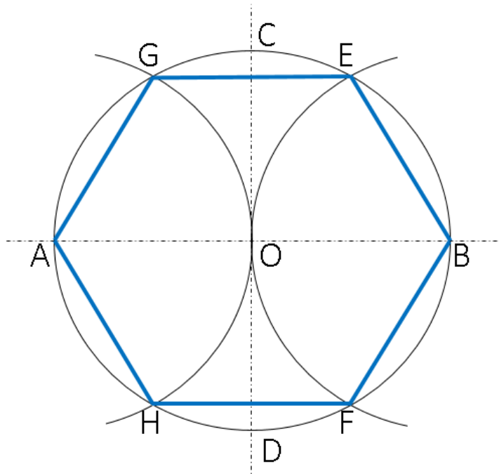
Şekil 1.1.20: Altıgen çizimi
