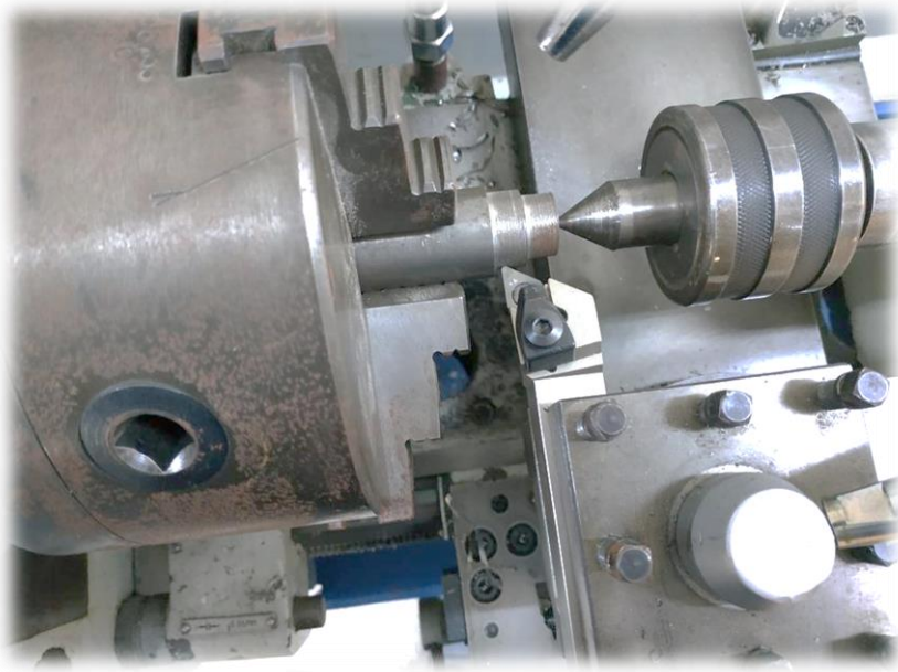
Şekil 1.3.10: Kademeli tornalama
