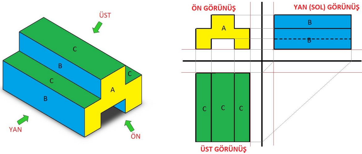
Şekil 1.1.25: Görünüş çıkarma
