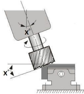
Şekil 1.4.6: Eğik frezeleme
