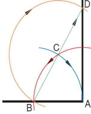
Şekil 1.1.16: Doğru parçasına dik açı çizme
