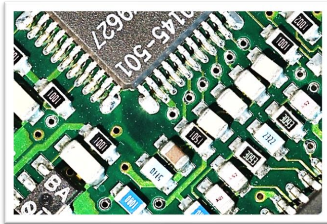
Şekil 4.4.3: Çift taraflı PCB kart
