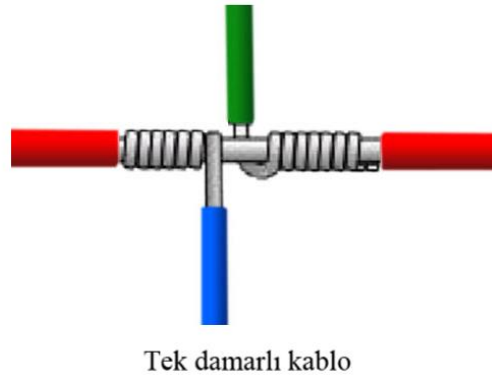
Şekil 4.2.4: Çift T ek bağlantısı
