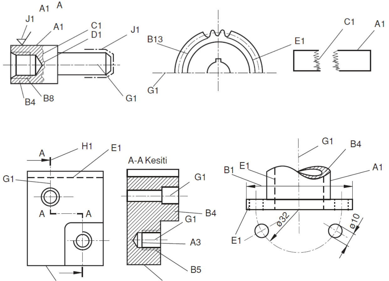
Şekil 1.1.10: Çizgi çizim örnekleri
