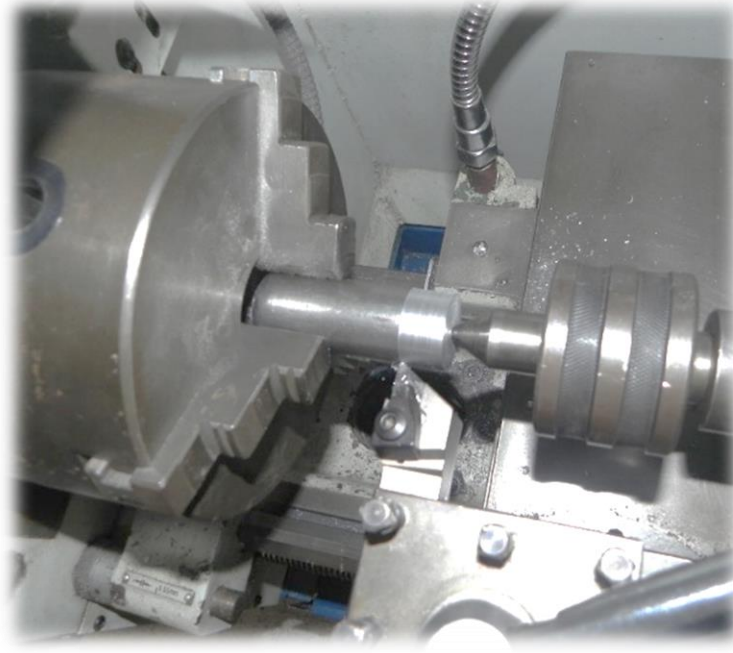
Şekil 1.3.9: Yüzey tornalama
