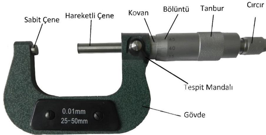
Şekil 1.3.13: Mikrometre
