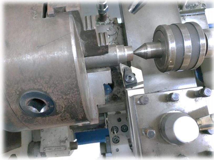
Şekil 1.3.10: Kademeli tornalama
