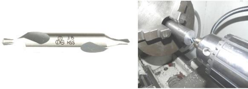
Şekil 1.3.8: Punta deliği delme
