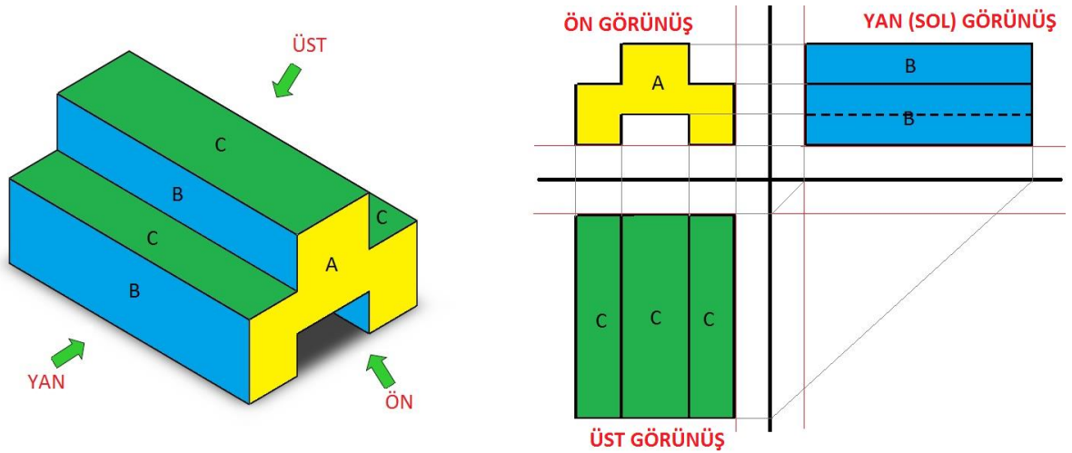
Şekil 1.1.25: Görünüş çıkarma
