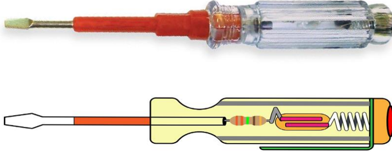
Şekil 4.1.4: Kontrol kalemi
