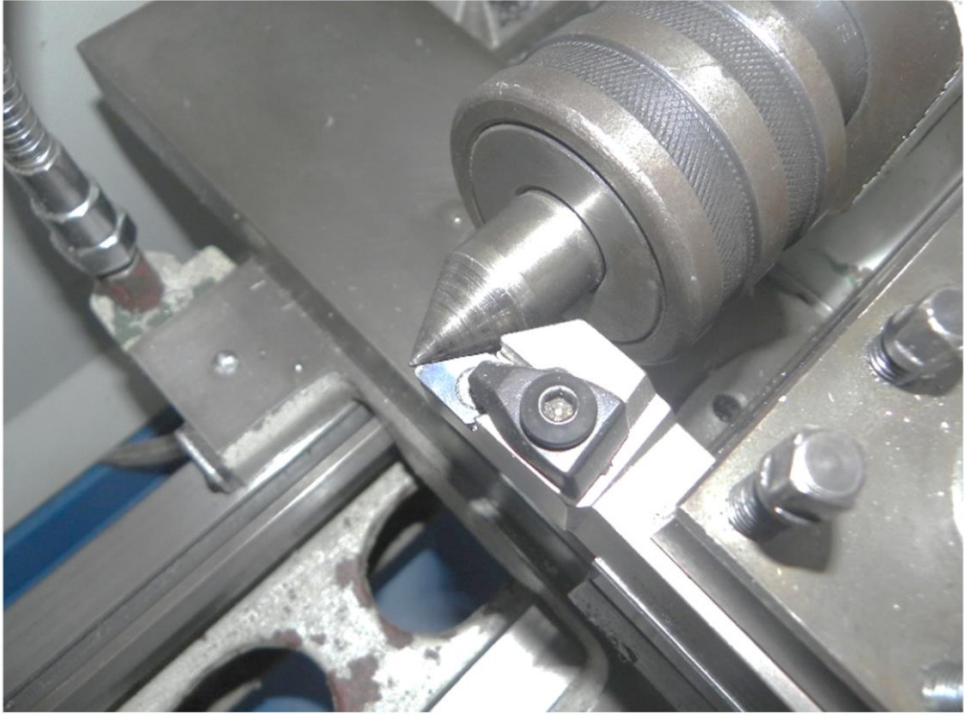
Şekil 1.3.6: Punta yüksekliğinde bağlanmış kesici takım
