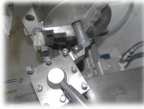
Şekil 1.3.7: Alın tornalama işlemi
